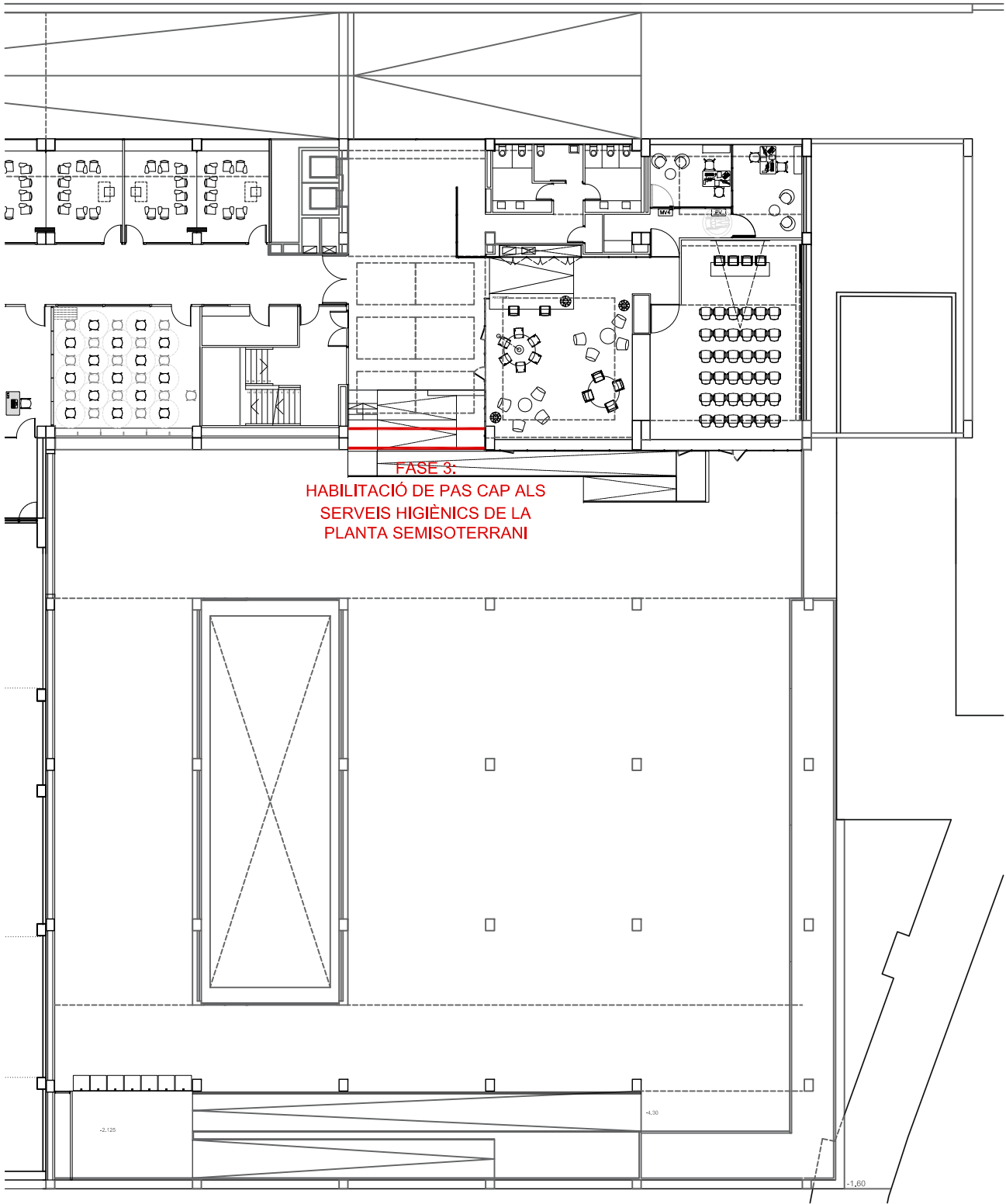
PLANTA SEMISOTERRANI
