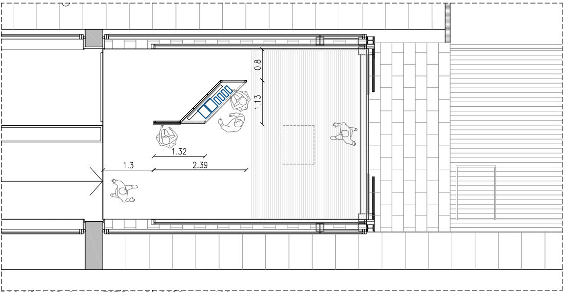
POSICIÓ MOB G AL VESTÍBUL D'ACCÉS e. 1:100
