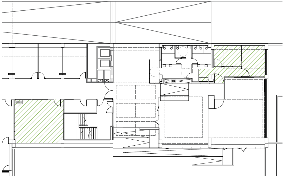
PLANTA SEMISOTERRANI CEL RASOS
