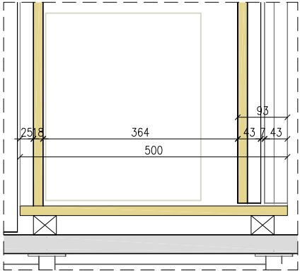
DETALL 3 e. 1/10
