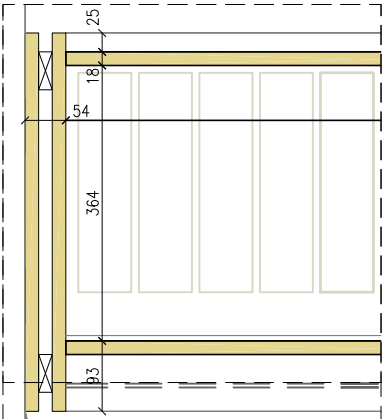
DETALL 1 e. 1/10
