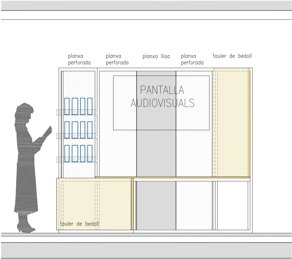
ALÇAT AA'. MOBLE G e.1:25
