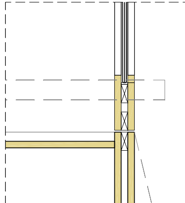
DETALL 4 e. 1/10
