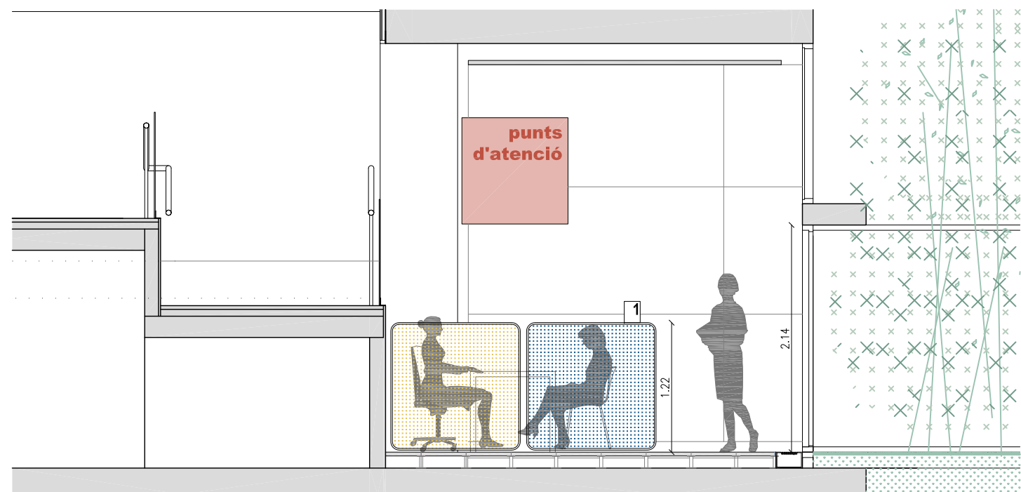
SECCIÓ BB' e.1:25
