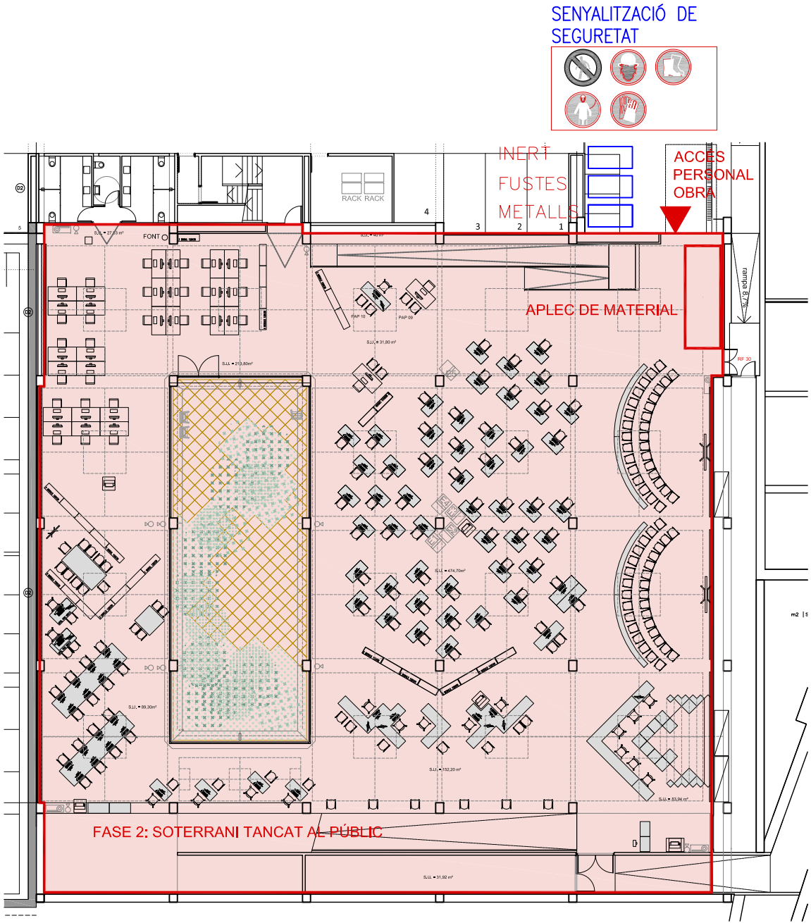
PLANTA SOTERRANI
