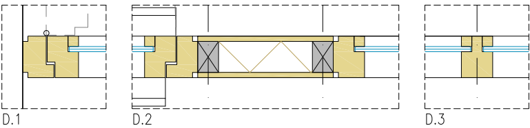
DETALLS FUSTERIA DE FUSTA, en planta e.1:10
