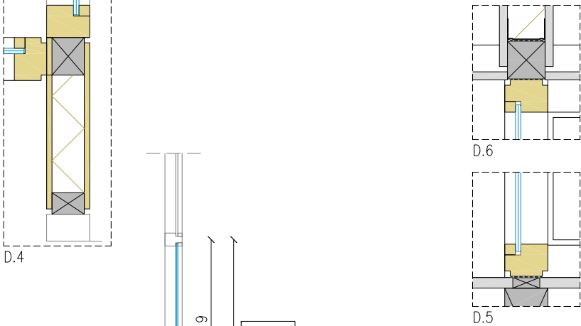
DETALLS FUSTERIA DE FUSTA, en secció e.1:10
