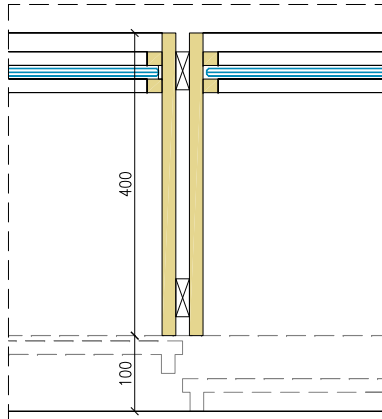
DETALL 3 e. 1/10
