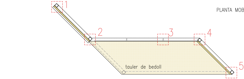
DETALLS FUSTERIA MOB G e. 1:10
