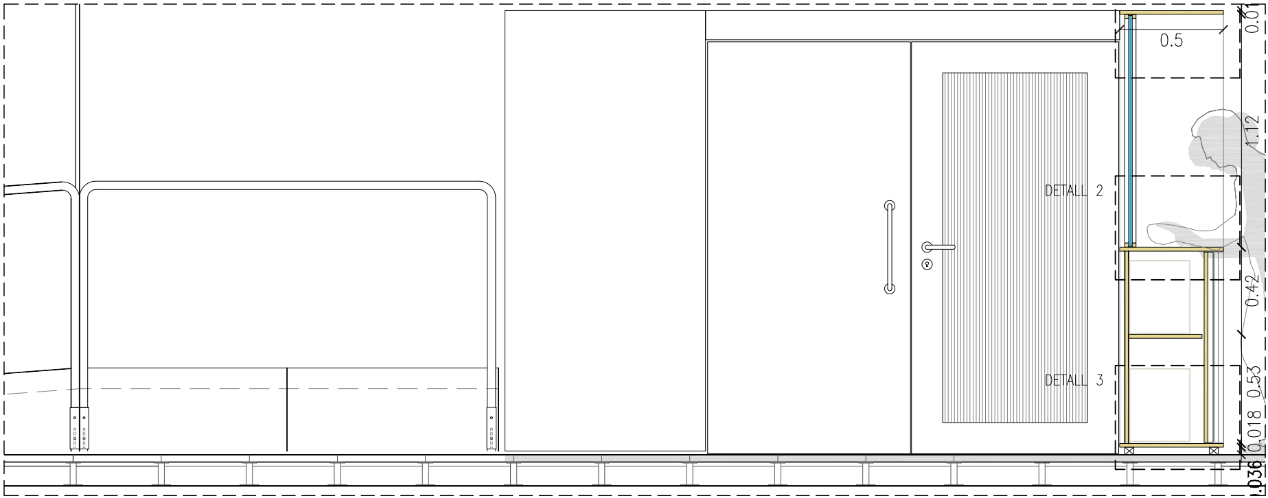
ALÇAT AA' e. 1/25
