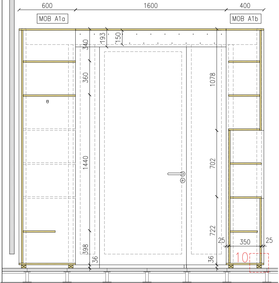
SECCIÓ BB'. MOB A1, MÒDULS A1a i A1b e.1:25
