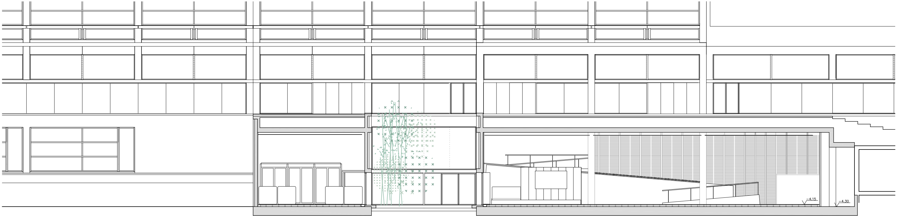
SECCIÓ B-B'
