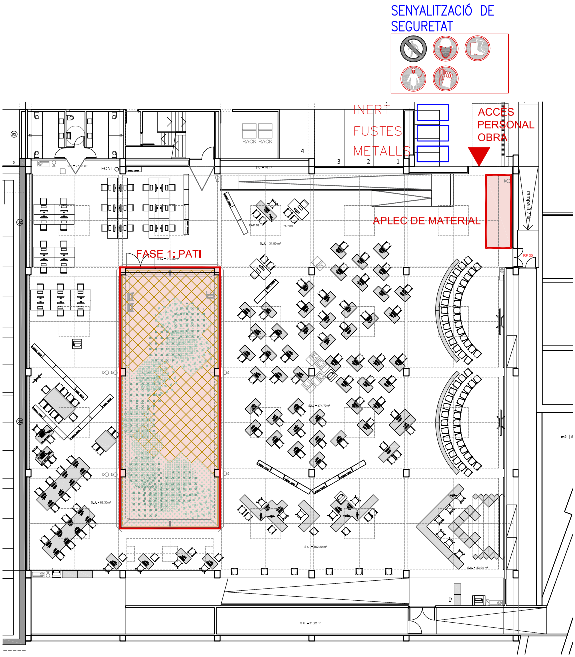
PLANTA SOTERRANI
