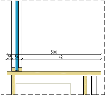
DETALL 2 e. 1/10
