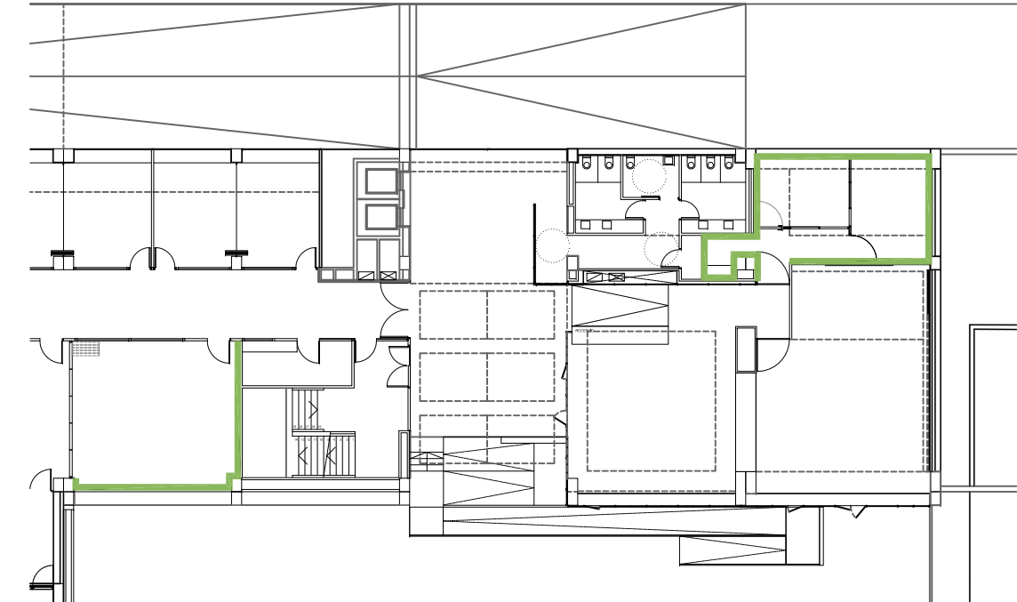
PLANTA SEMISOTERRANI
