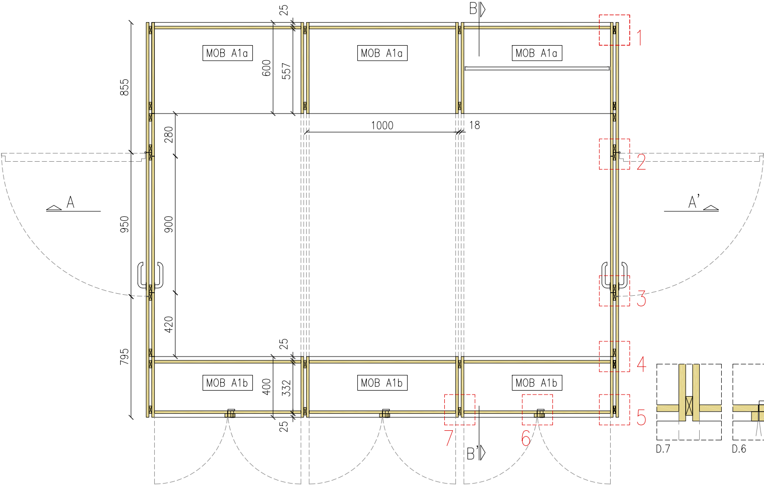
PLANTA MOB A e.1:25
