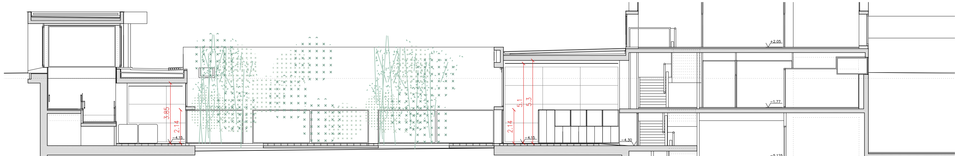
SECCIÓ D-D'
