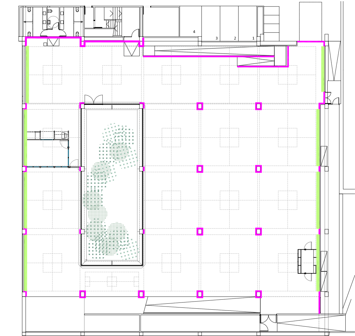
PLANTA SOTERRANI
