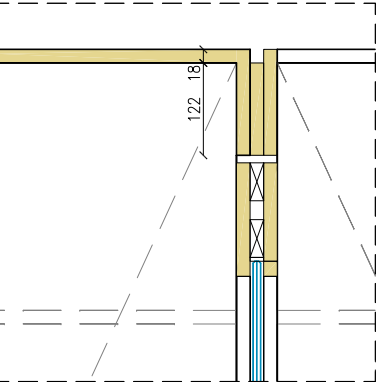
DETALL 5 e. 1/10
