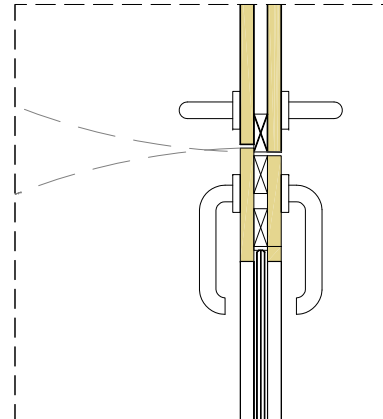
DETALL 5 e. 1/10
