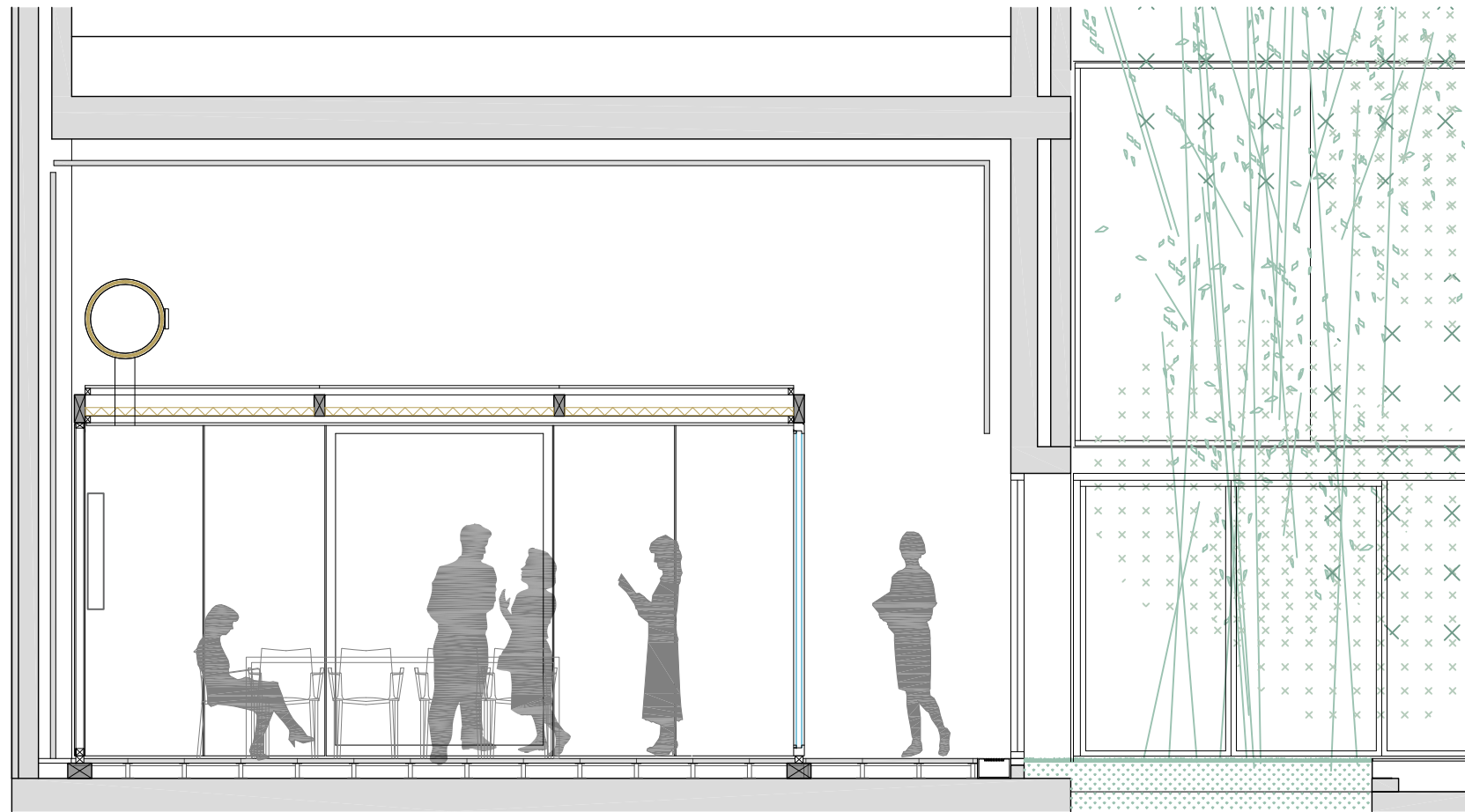
SECCIÓ AA'
