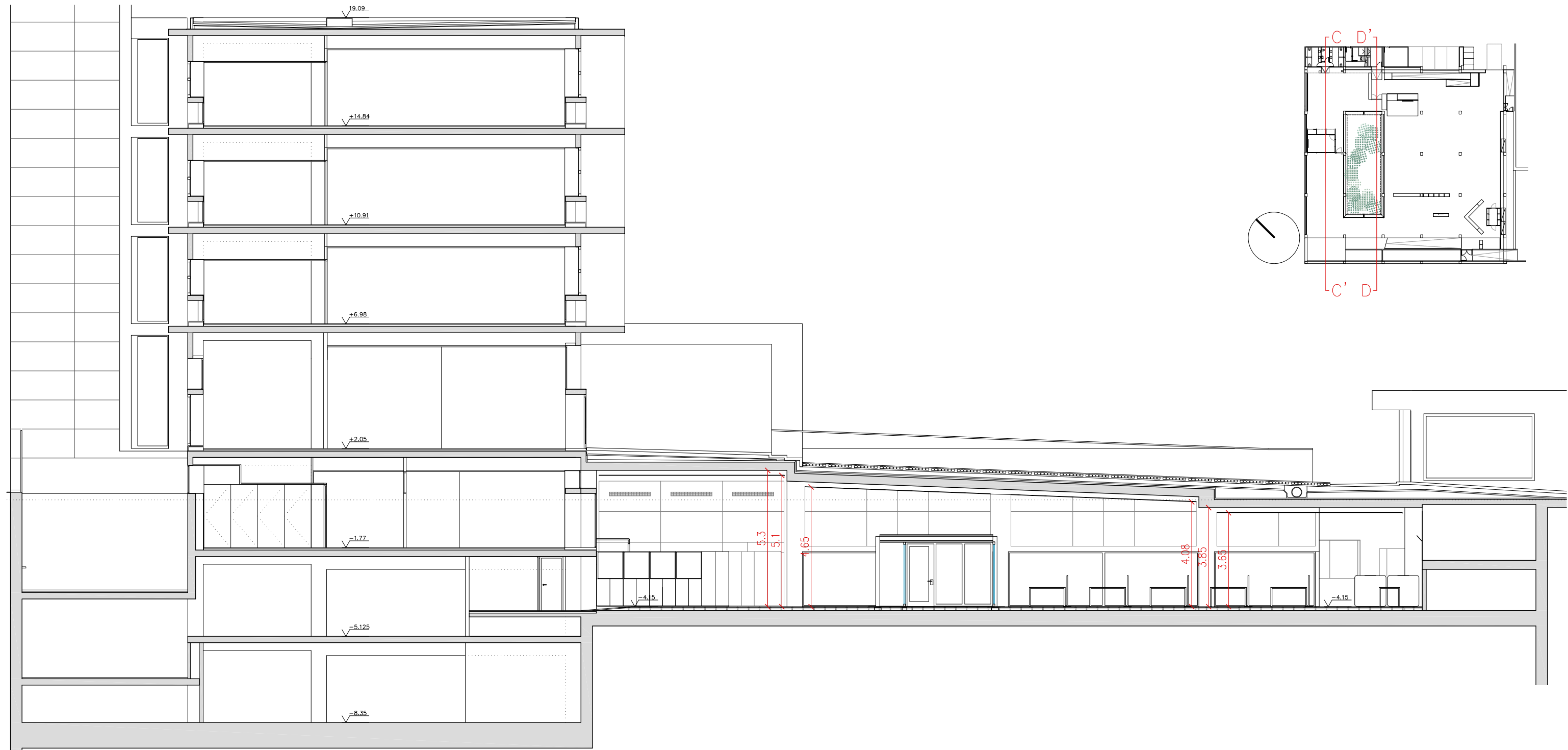
SECCIÓ C-C'
