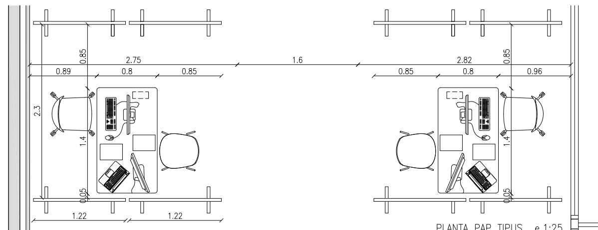
PLANTA PAP TIPUS e.1:25
