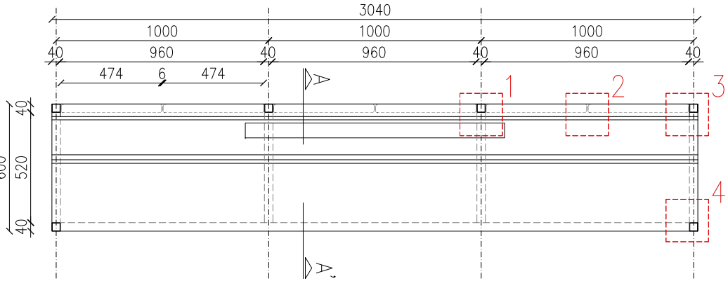
PLANTA MOB B. e.1:25
