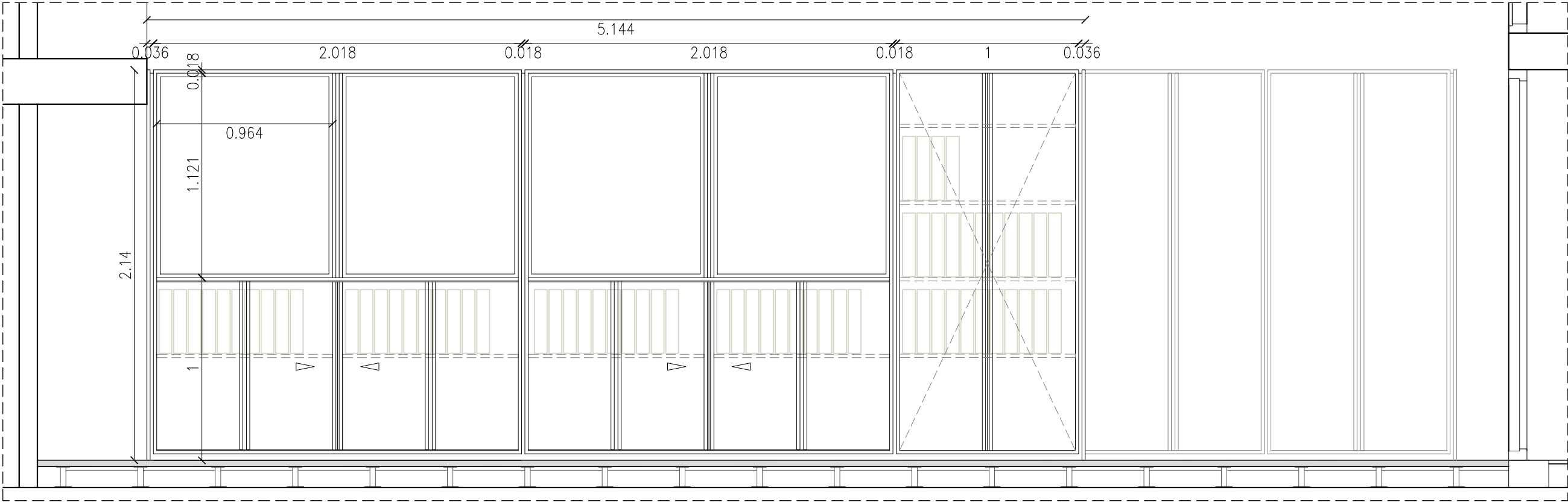
ALÇAT CC' e. 1/25
