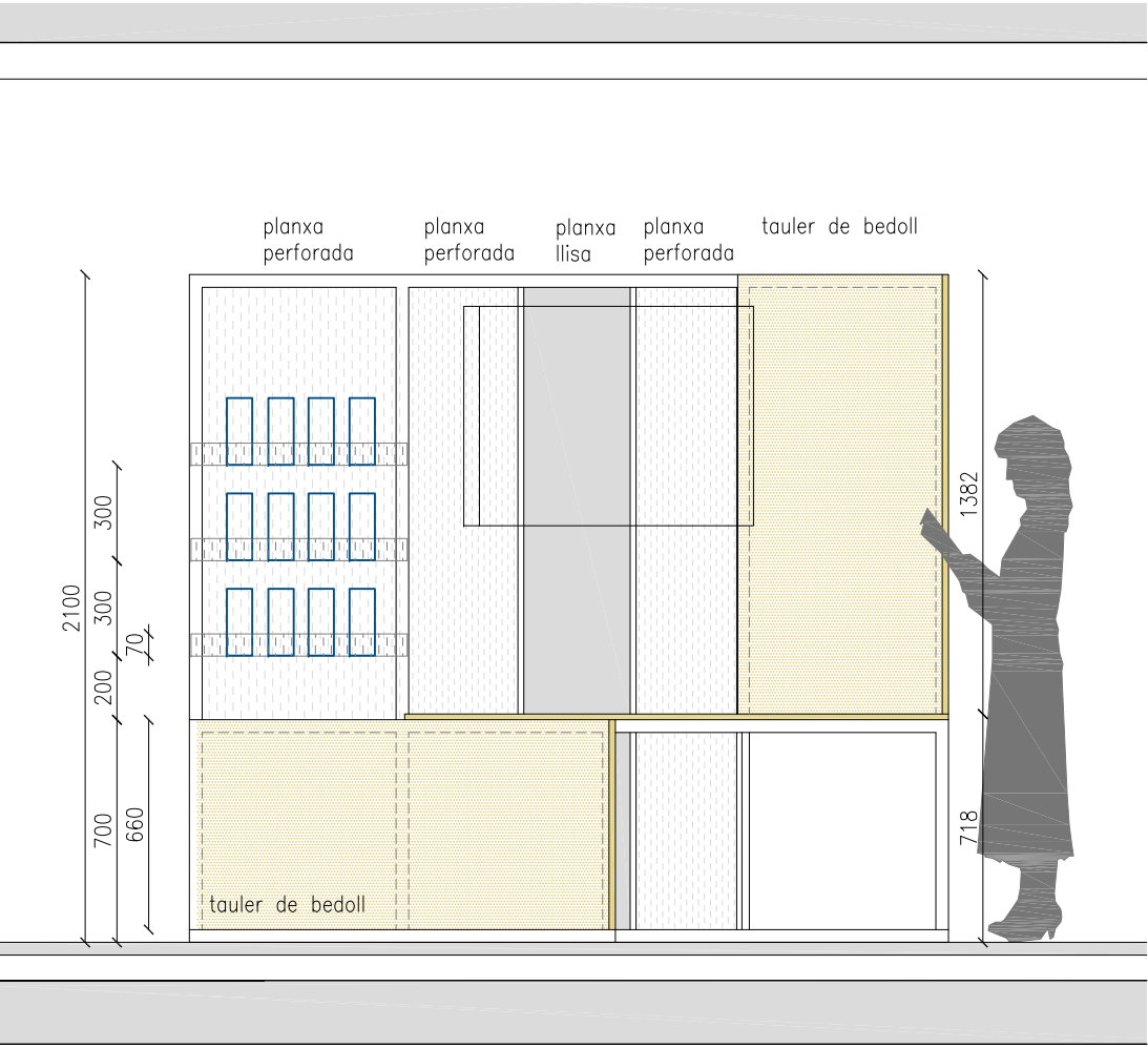
ALÇAT BB' MOB G. e.1:25
