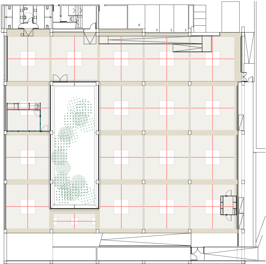
PLANTA SOTERRANI CEL RASOS
