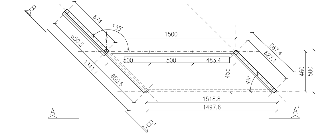
ALÇAT AA'. MOBLE G e.1:25
