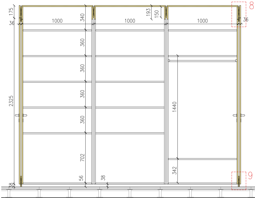
SECCIÓ AA'. MOB A1, MÒDULS A1a e.1:25
