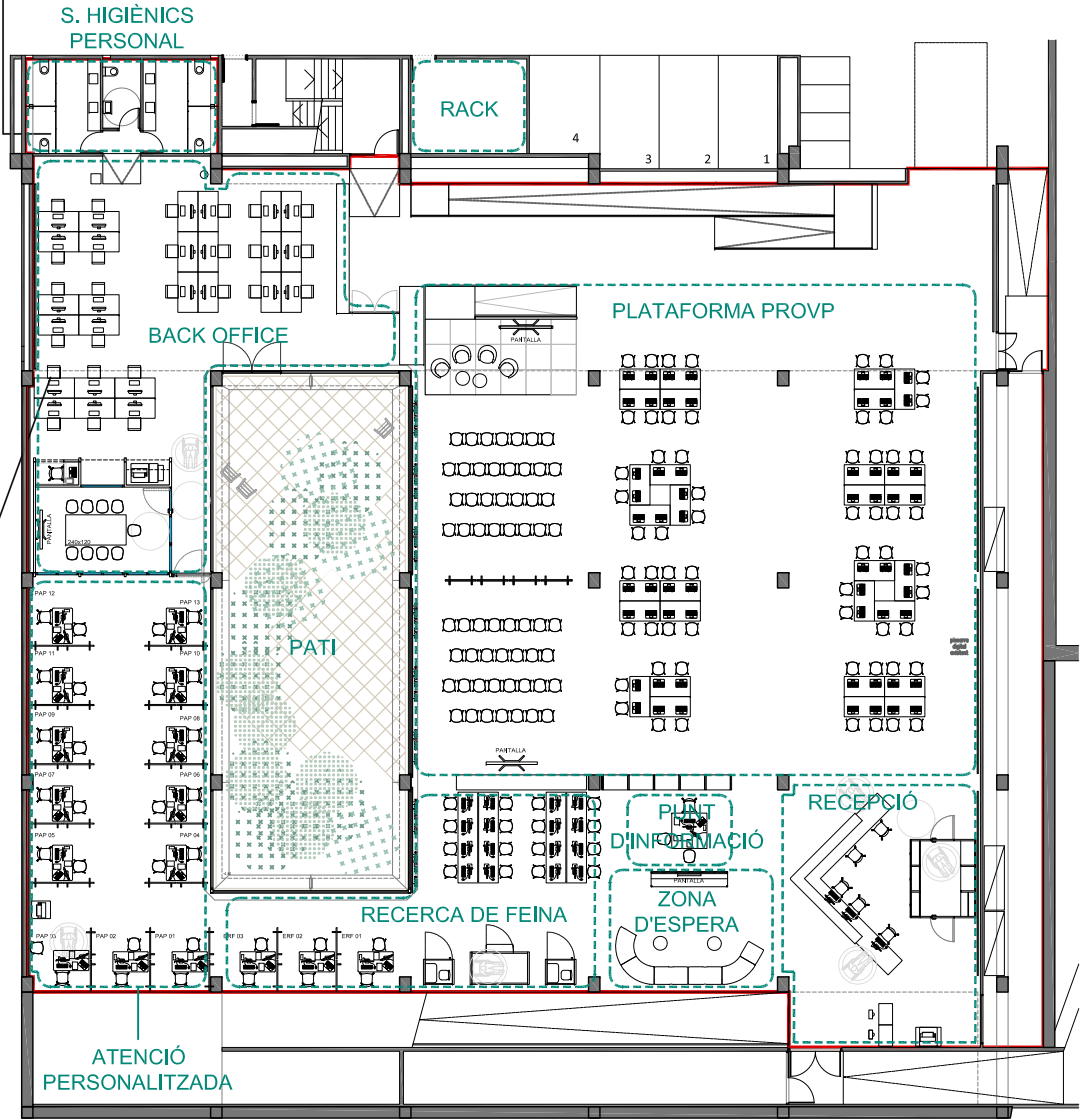
PLANTA SOTERRANI
