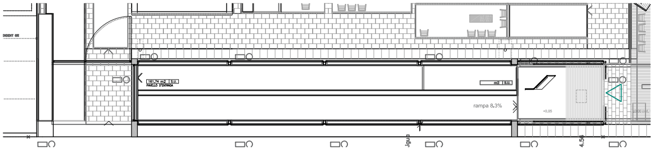
PLANTA SEMISOTERRANI
