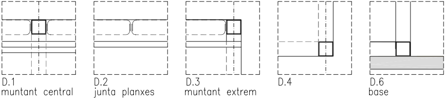
DETALLS FUSTERIA METÀL·LICA MOB B e. 1:10
