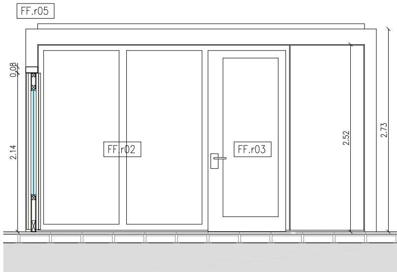
ALÇAT GG'
