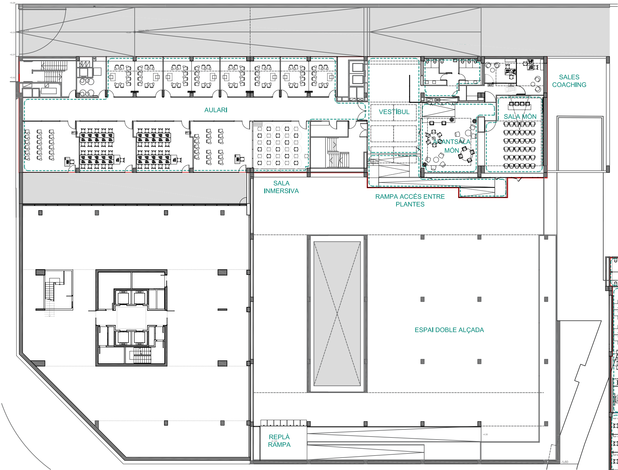
PLANTA SEMISOTERRANI
