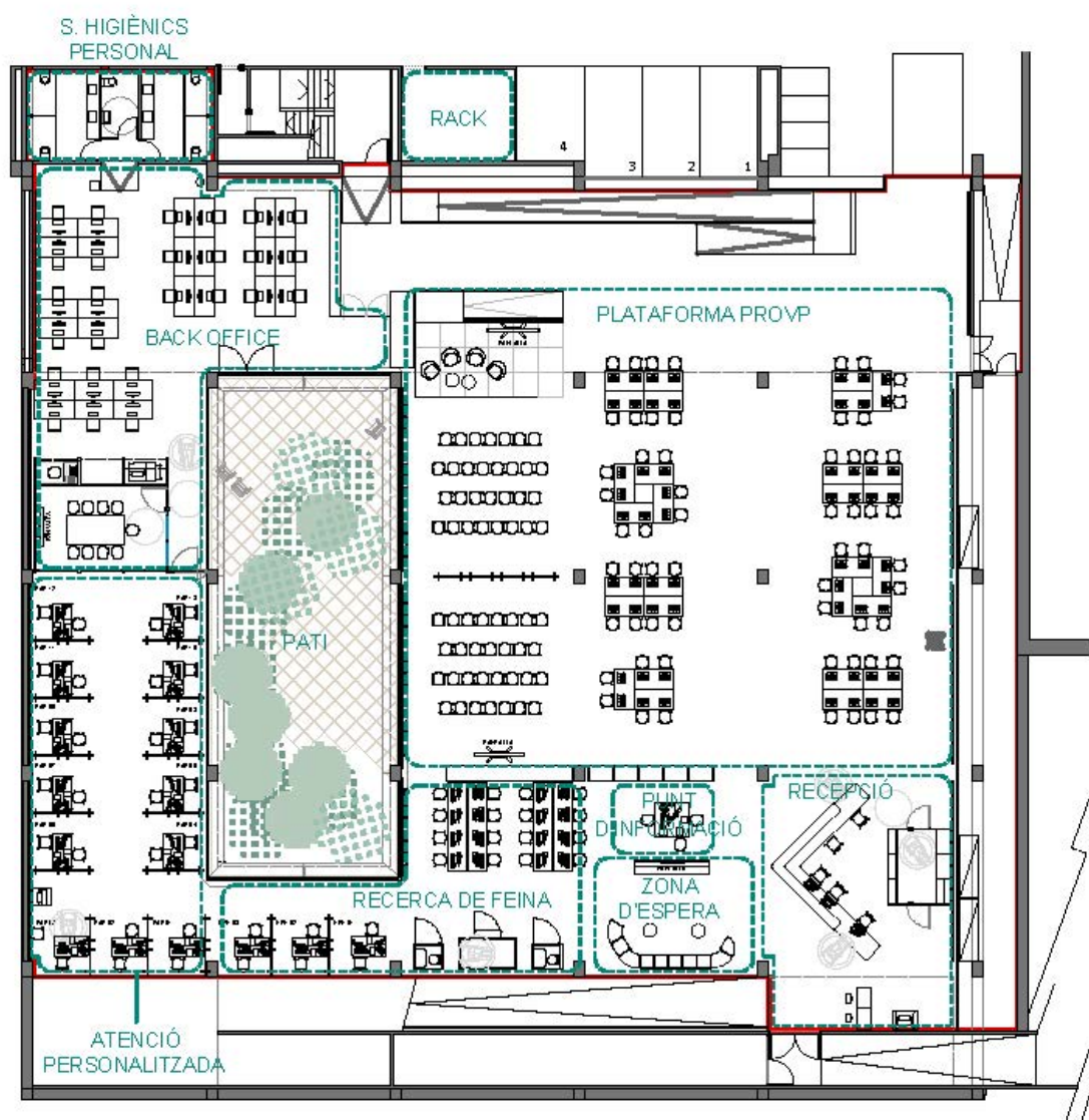
Planta soterrani
