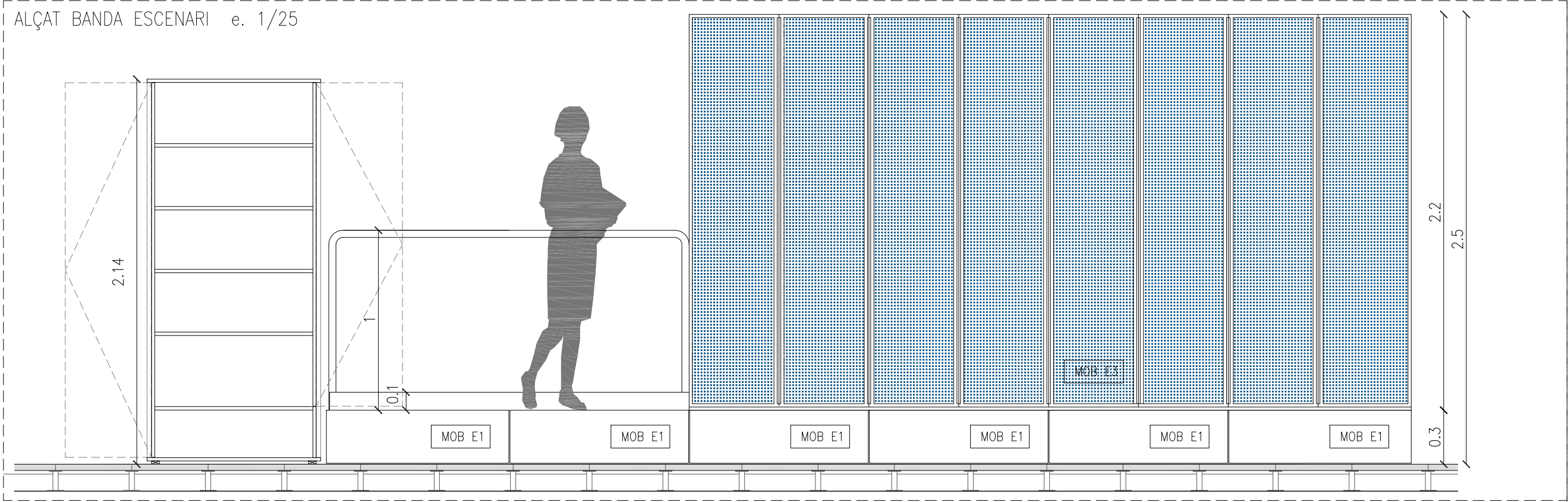
SECCIÓ BANDA ESCENARI e. 1/25
