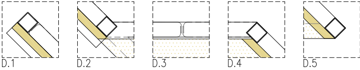
DETALLS FUSTERIA MOB G e. 1:10
