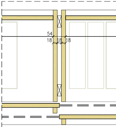
DETALL 2 e. 1/10
