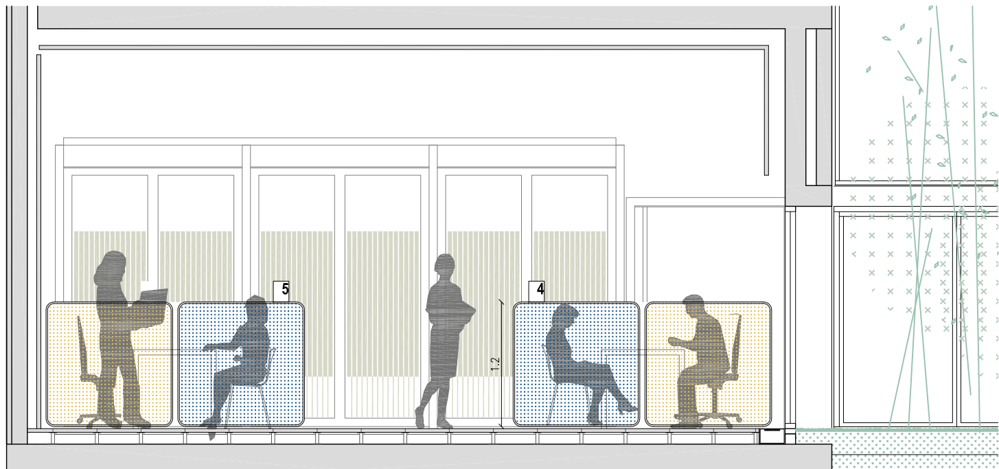
SECCIÓ AA' e.1:25
