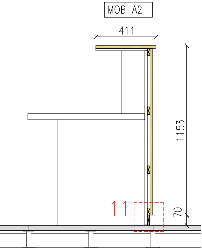
SECCIÓ TIPUS MOB A2. e.1:25
