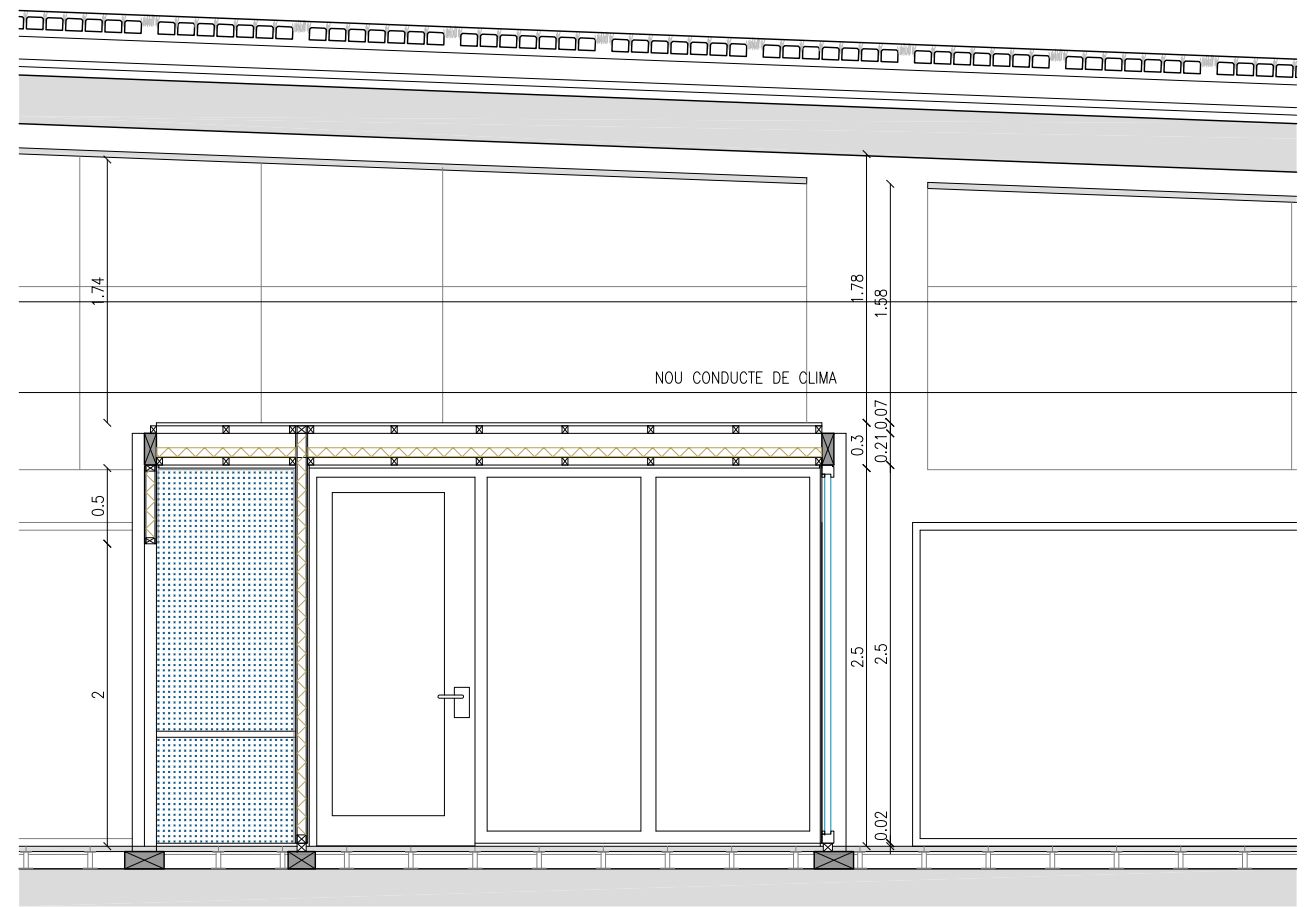
SECCIÓ BB'
