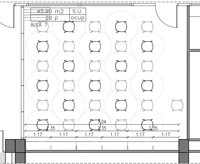
POSICIÓ MOB H A L'AULA IMMERSIVA e. 1:100
