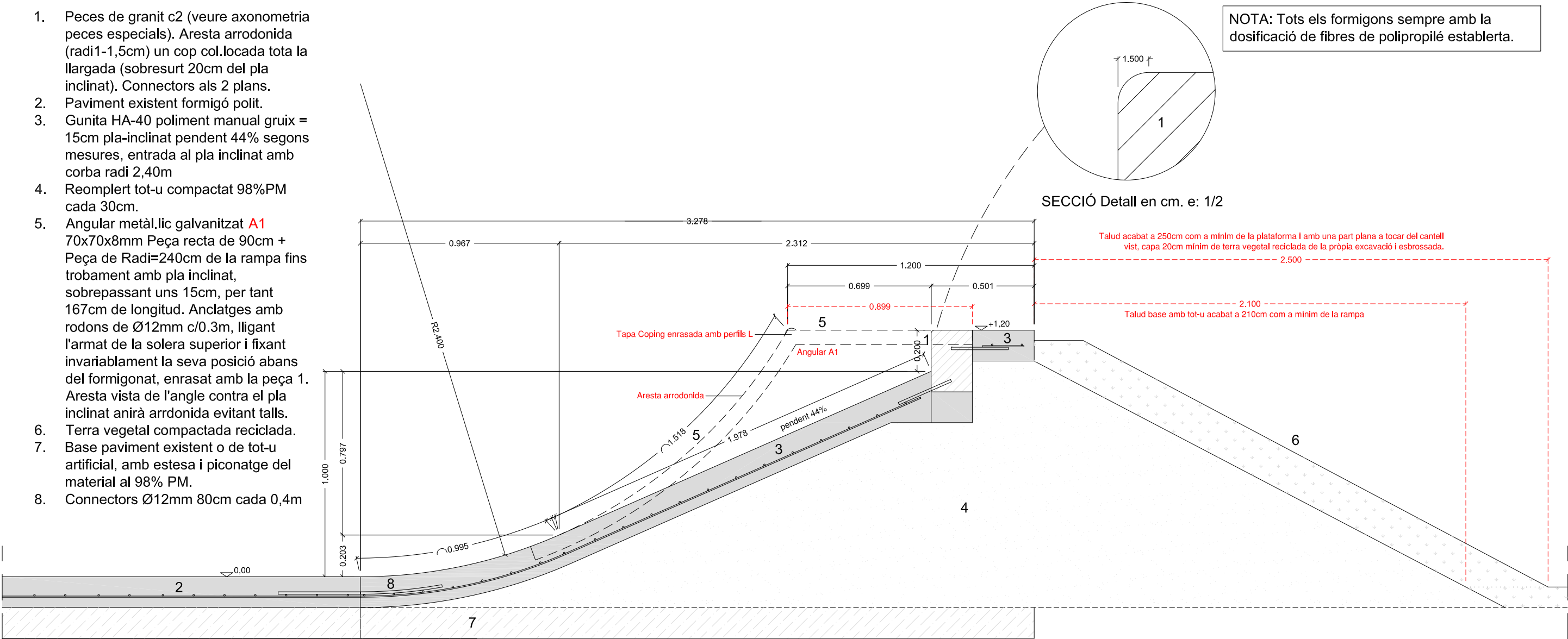
SECCIÓ 1
