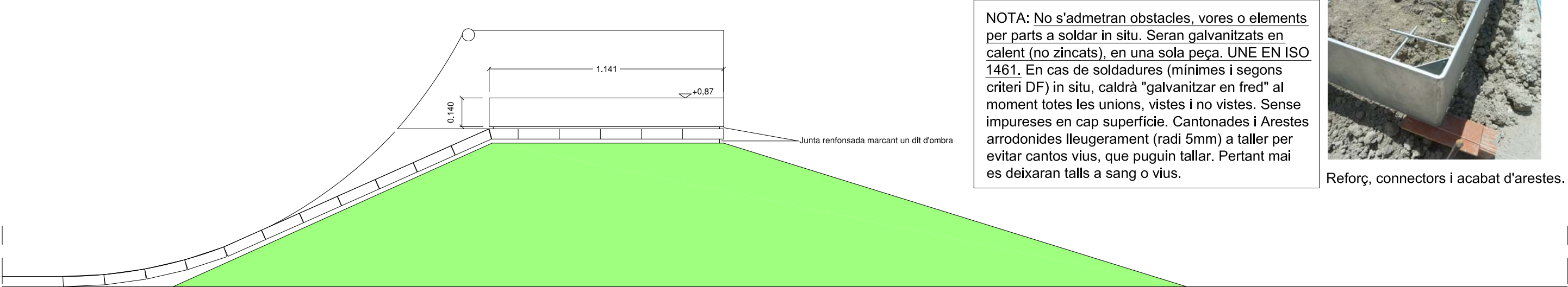
DETALL ALÇAT 1
