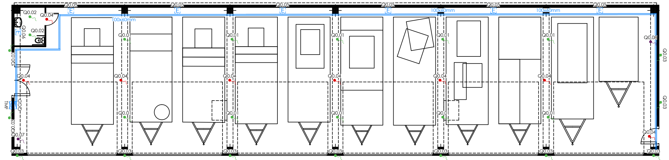
PLANTA BAIXA
