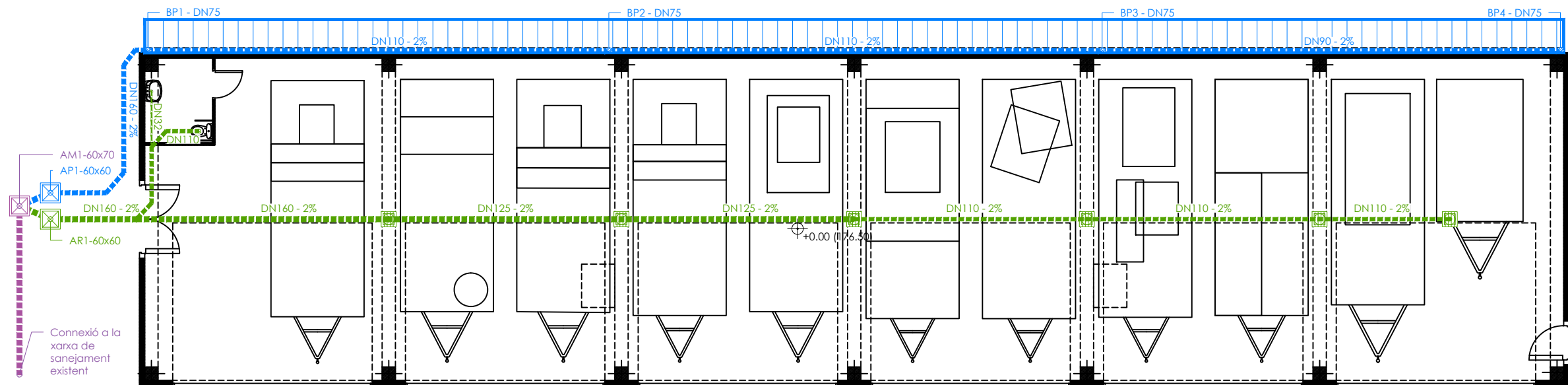
PLANTA BAIXA
