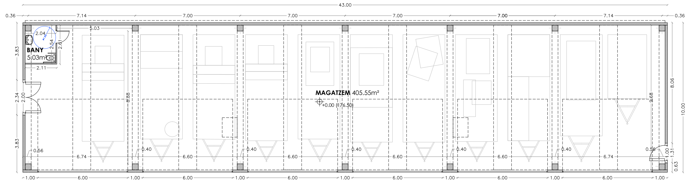
PLANTA BAIXA
