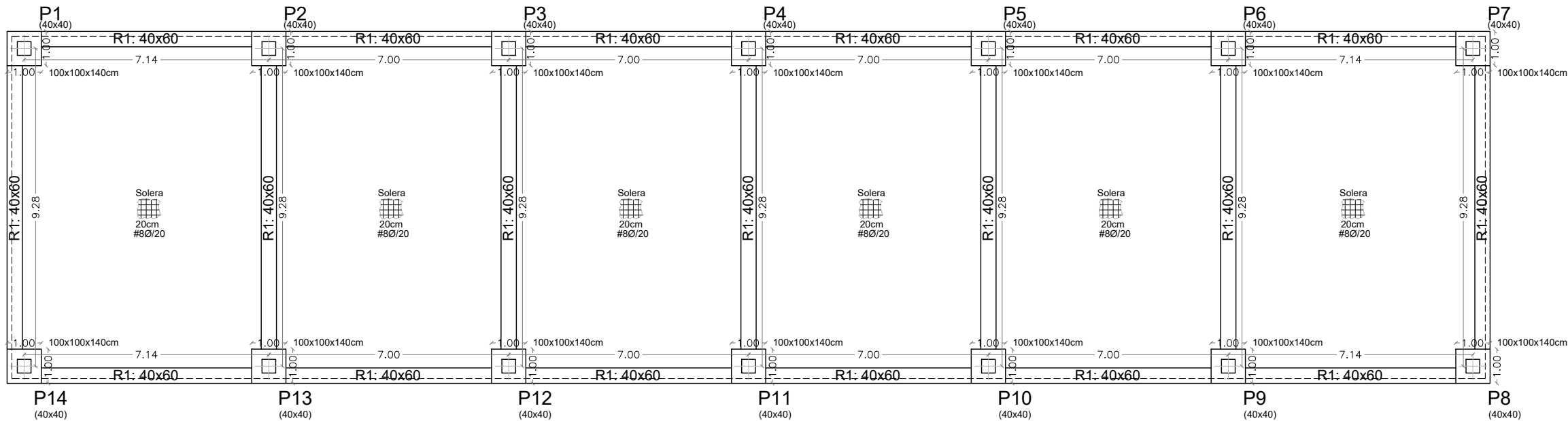
PLANTA FONAMENTS
