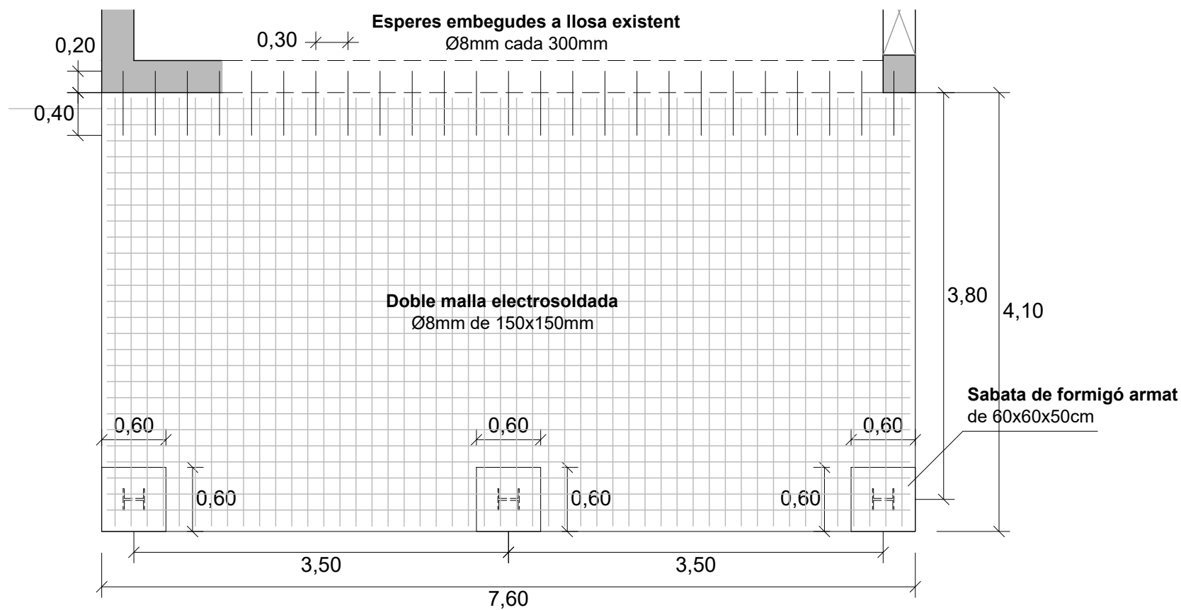
FONAMENTS - Sabates aïllades + Llosa de solera
