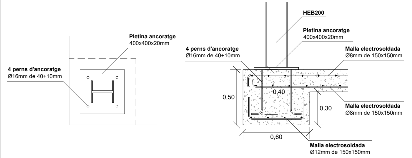
DETALL DE SABATA AÏLLADA / escala 1:20
