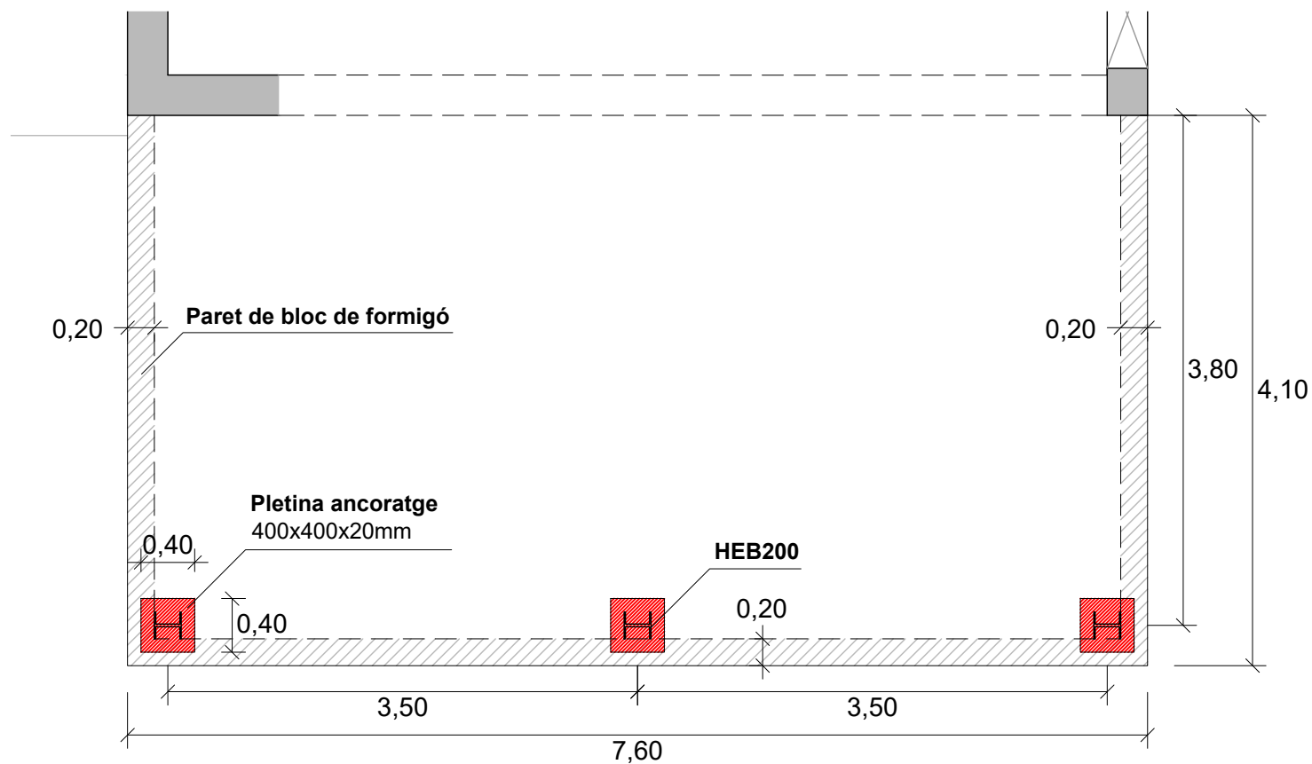
SOBRE SOLERA - Pletines ancoratge + Muret perimetral
