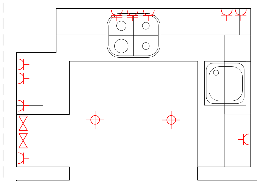
Planta cuina
