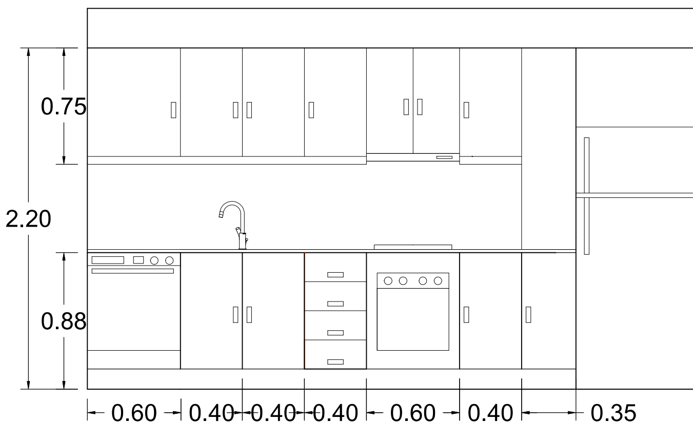
ALÇAT CUINA
