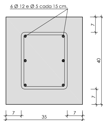
Riostra detall A escala 1:10
