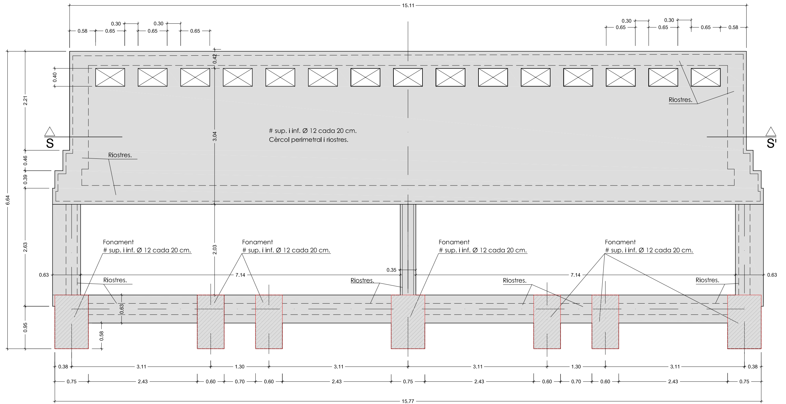
PLANTA FONAMENTS
