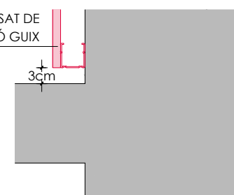
DETALL B
