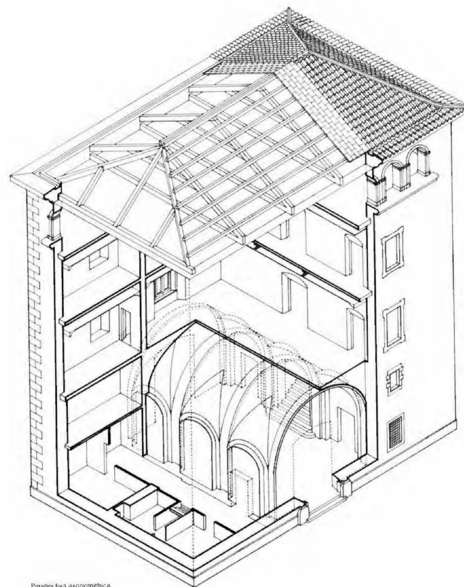
Perspectiva axonòmica de l'edifici publicada l'any 1983. Reflecteix l'edifici abans de la remodelació iniciada el 1984 103 .
