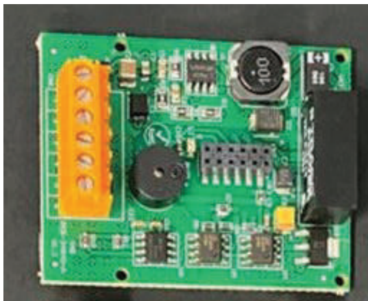
Imatge 5: Vista placa alimentació RFID interruptor CAN
