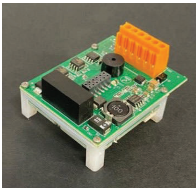
Imatge 4: Vista dels components restants una vegada muntats
