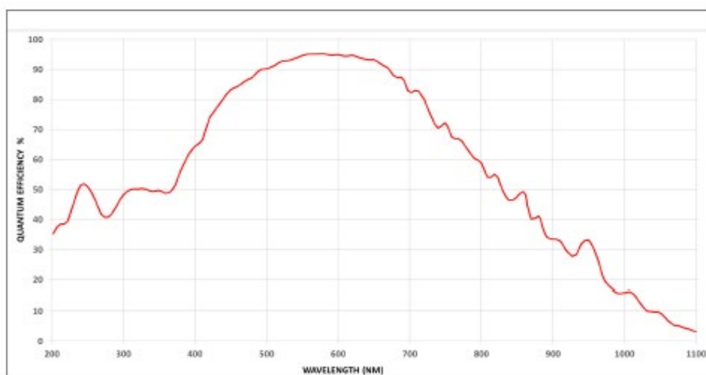
Eficiencia cuántica vs longitud de onda de la cámara Leica K8
