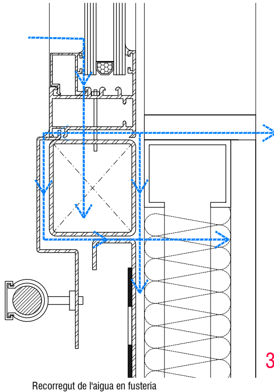
Recorregut de l'aigua en fusteria
