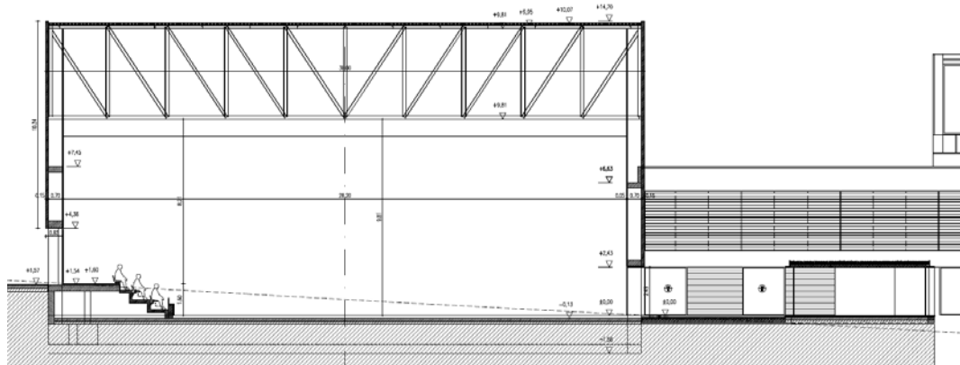
Figura A-9 Secció Transversal
