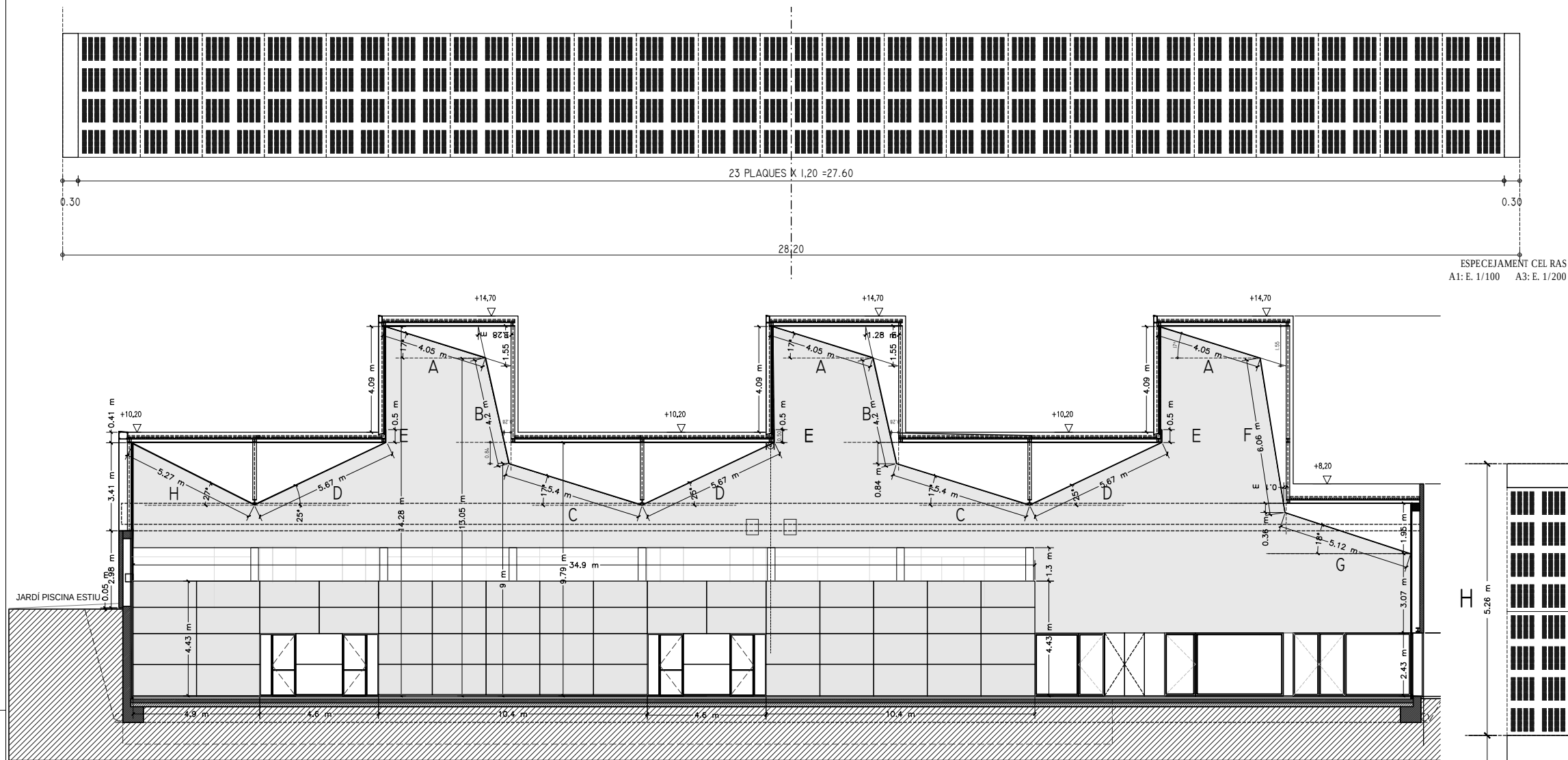
ALÇAT ACCÉS VESTIDORS A1: E. 1/100 A3: E. 1/200
