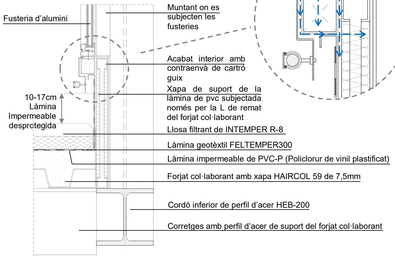
Figura RT-7 Detall observat durant les visites a la coberta i punts d'entrada d'aigua
