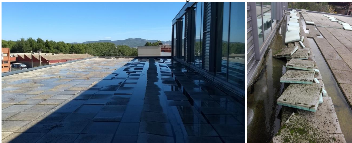
Figura A-12 Prova d'estanquitat i extracció de paviment
