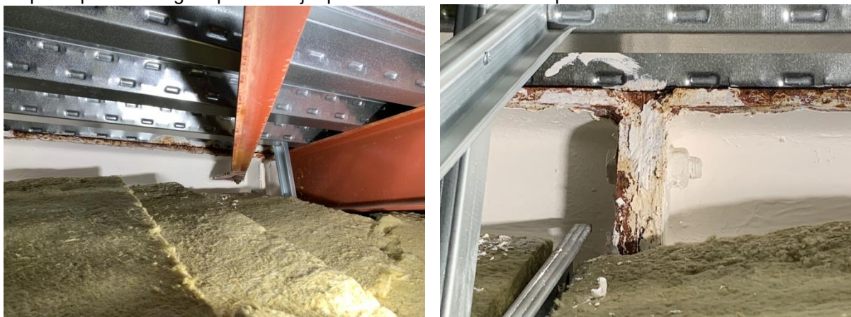
Figura RT-9 Fotografies dels perfils de coberta vistos a la Cala E1
