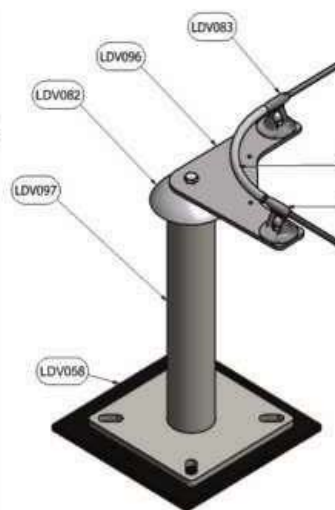
Fig. 3 Configuración en curva
