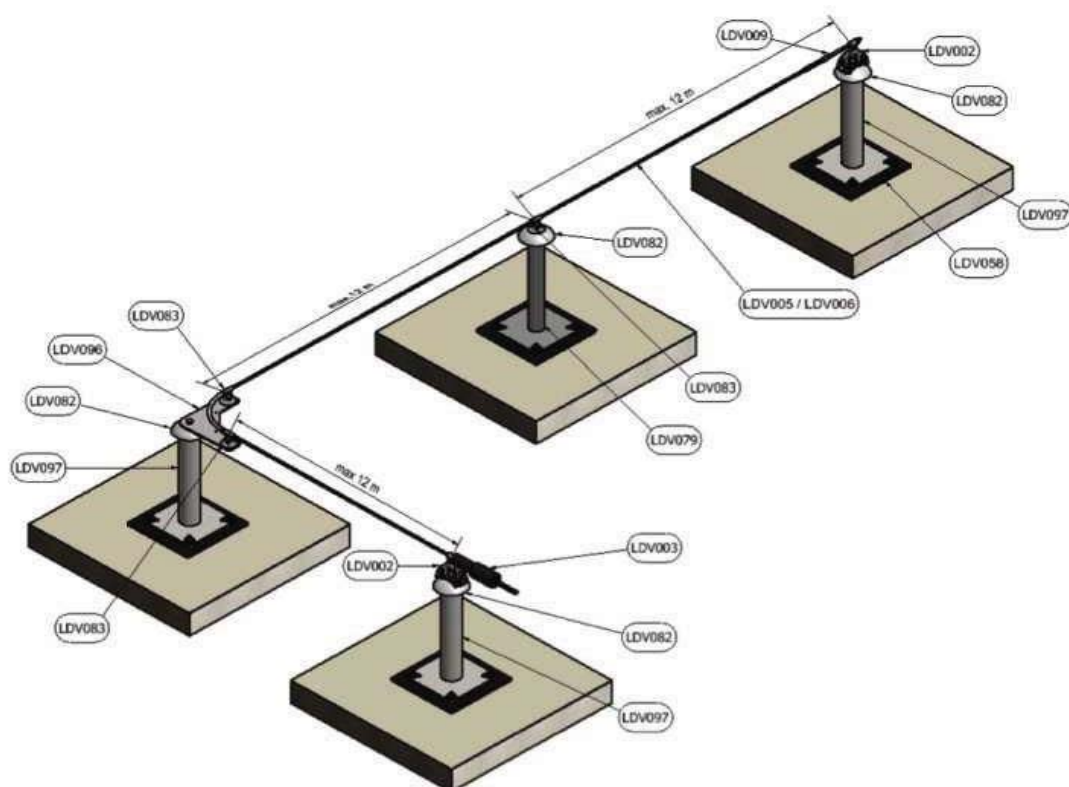
Fig. 5 Configuración de la línea básica de vida SecuRope en poste con anclaje intermedio EVO
