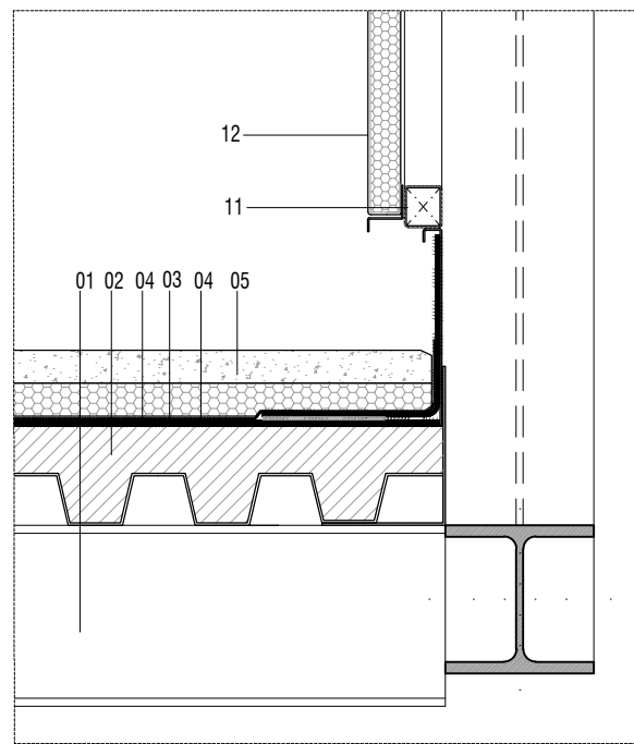
DETALL 2 A1 E.1/5 A3 E.1/10
