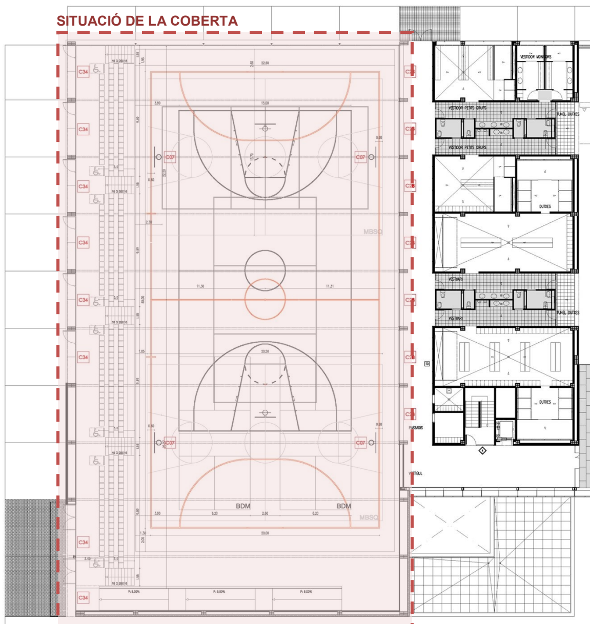
Figura A-8 Planta Primera
