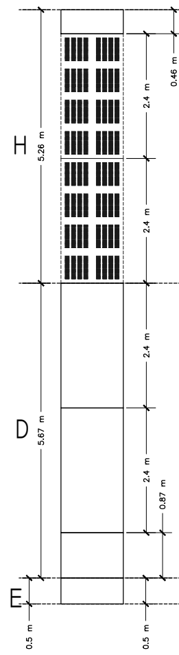
ALÇAT ACCÉS VESTIDORS A1: E. 1/100 A3: E. 1/200
