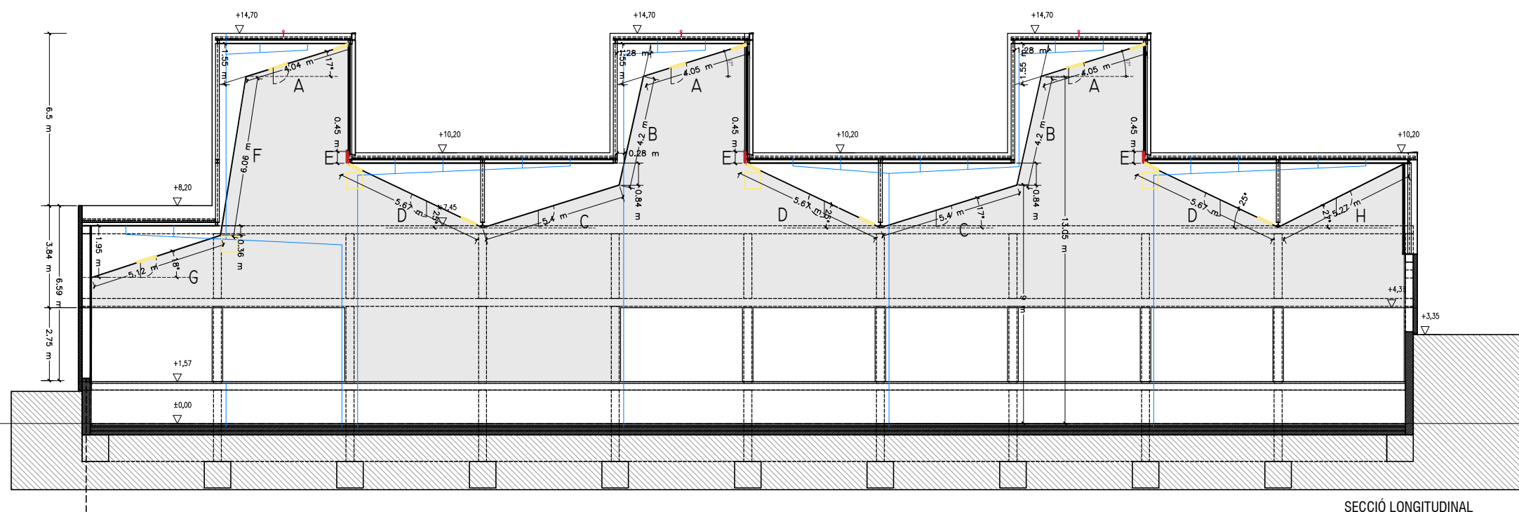
SECCIÓ LONGITUDINAL
