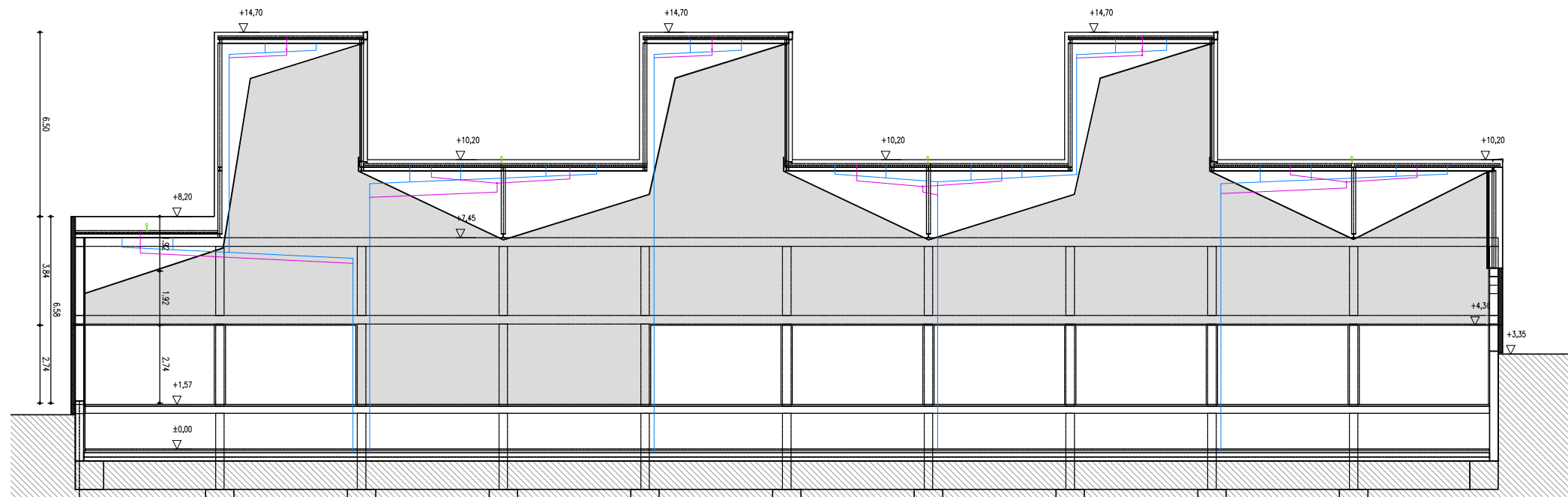
SECCIÓ LONGITUDINAL
