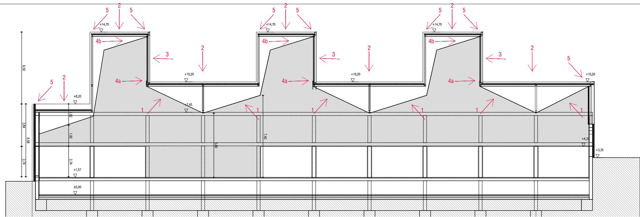
SECCIÓ LONGITUDINAL
