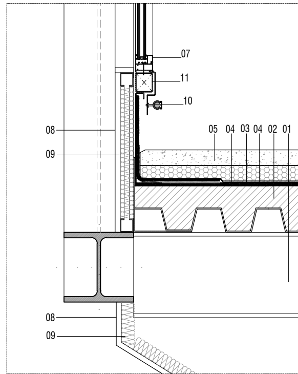
DETALL 1 A1 E.1/5 A3 E.1/10
