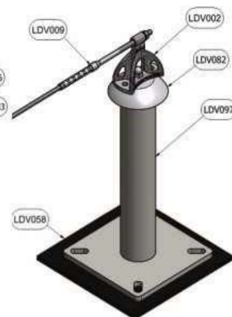
Fig. 4 Configuración de anclaje de un extremo con barra roscada
