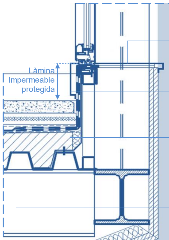
Figura RT-6 Detall extret del projecte ASBUILT
