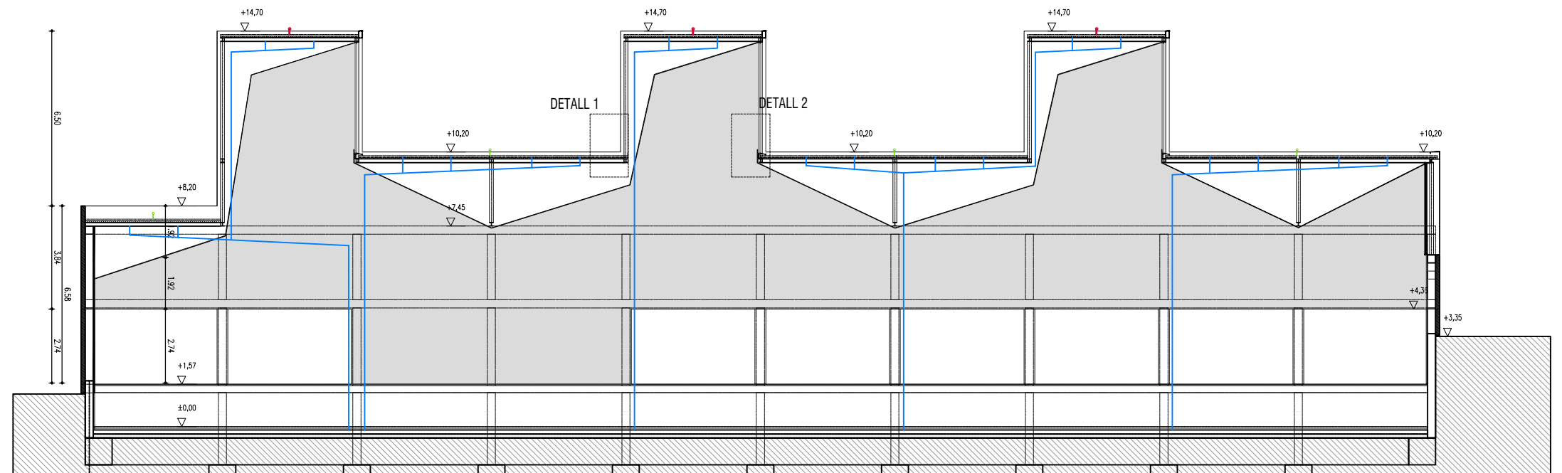
ESTAT ACTUAL SECCIÓ LONGITUDINAL
