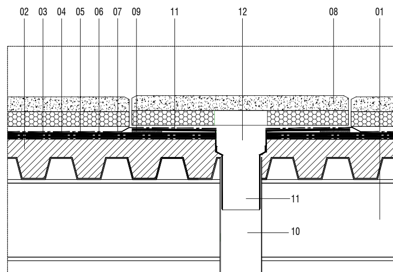
DETALL1 BONERA COBERTA A1 E.1/5 A3 E.1/10
