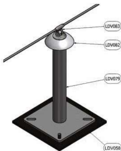
Fig.1 Configuración de anclaje intermedio
