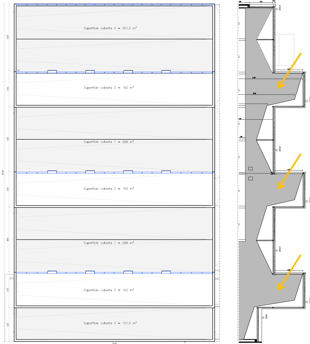
Figura A-10 Planta i secció Coberta
