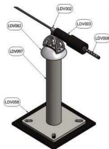
Fig. 2 Configuración de anclaje terminal
