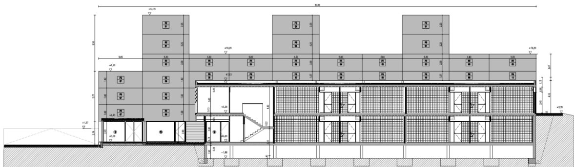
Figura A-6 Façana Est
