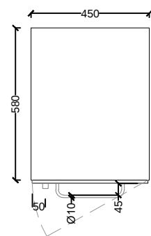
SECCIÓ AA'
