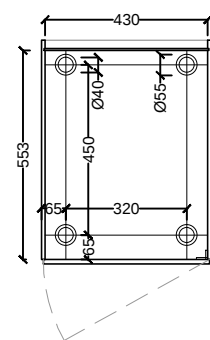
SECCIÓ BB'
