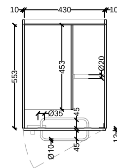
SECCIÓ CC'
