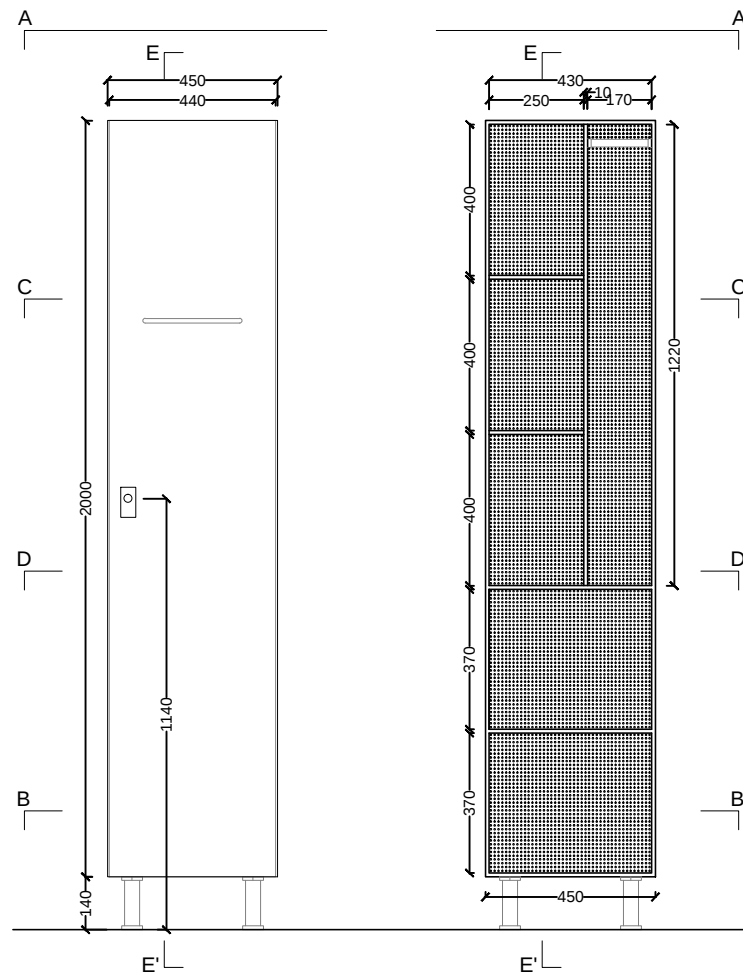
ALÇAT EXTERIOR
