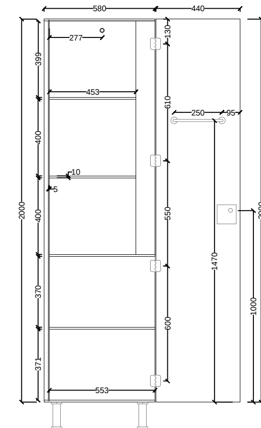
SECCIÓ EE' (porta oberta)
