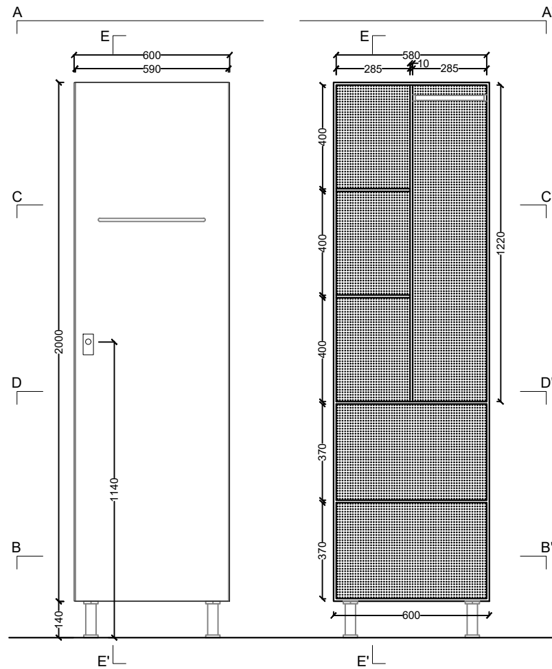
ALÇAT EXTERIOR
