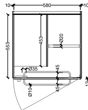
SECCIÓ CC'
