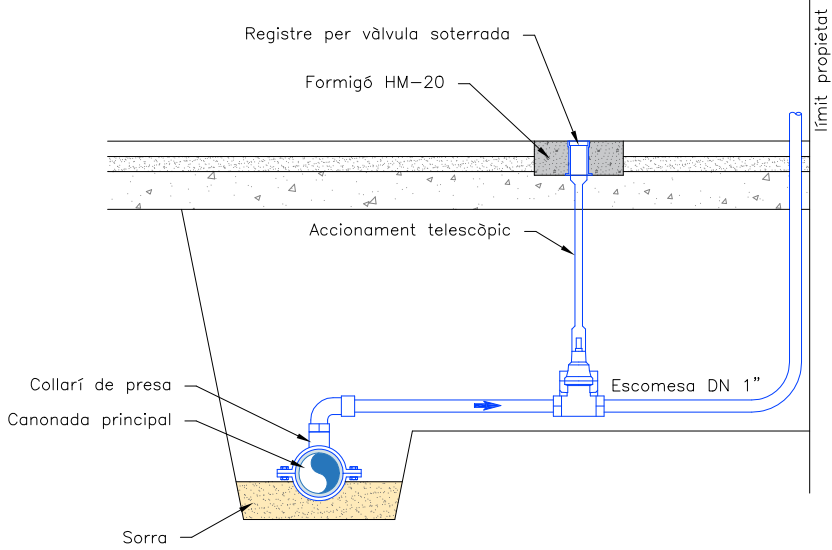
DETALL ESCOMESA Esc 1/20
