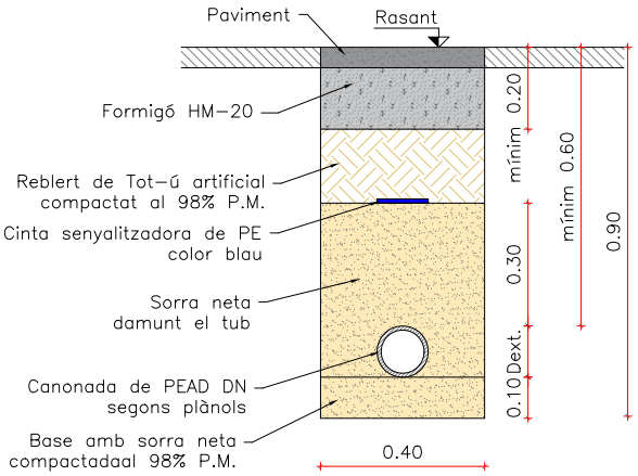
DETALL RASA EN PAVIMENT EXISTENT CANONADA PEAD Esc 1/20
