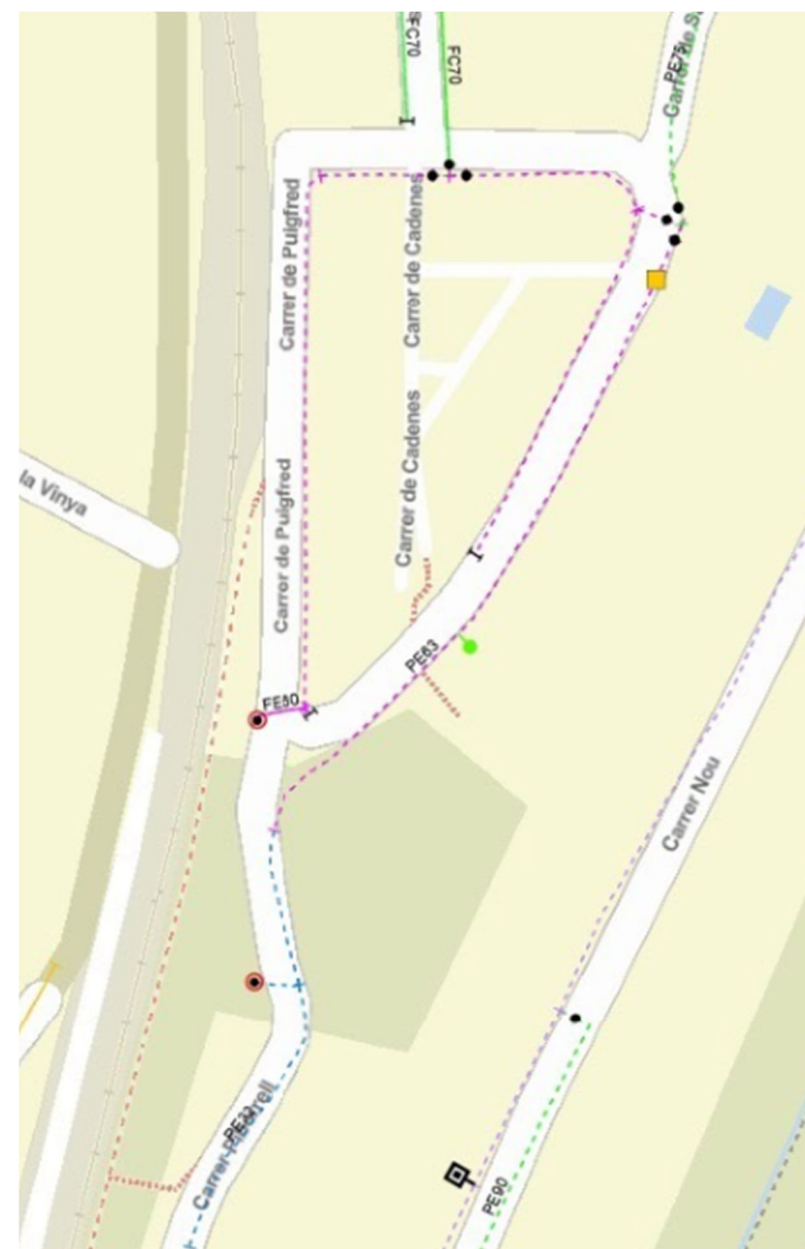
Figura 2. Planta estat actual xarxa d'aigua
