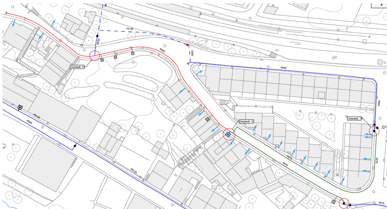
Figura 3. Planta proposada
