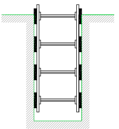
RASES AMB APUNTALAMENT PER SOBRECÀRREGA
