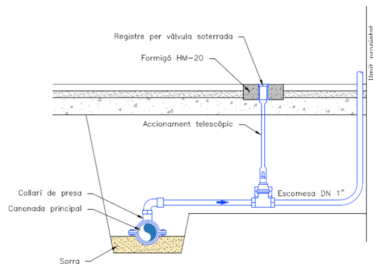
Figura 9. Detall connexió escomeses
