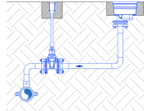
Figura 10. Detall connexió boques de reg
