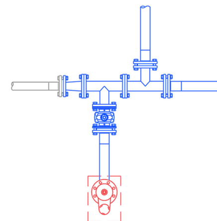
Figura 6. Detall connexió 3
