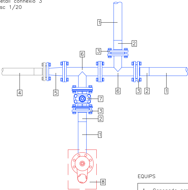
PLANTA
