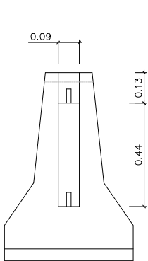
ALÇAT TRANSVERSAL
