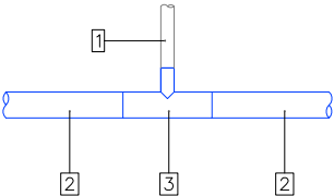
Detall connexió 4 Esc 1/20
