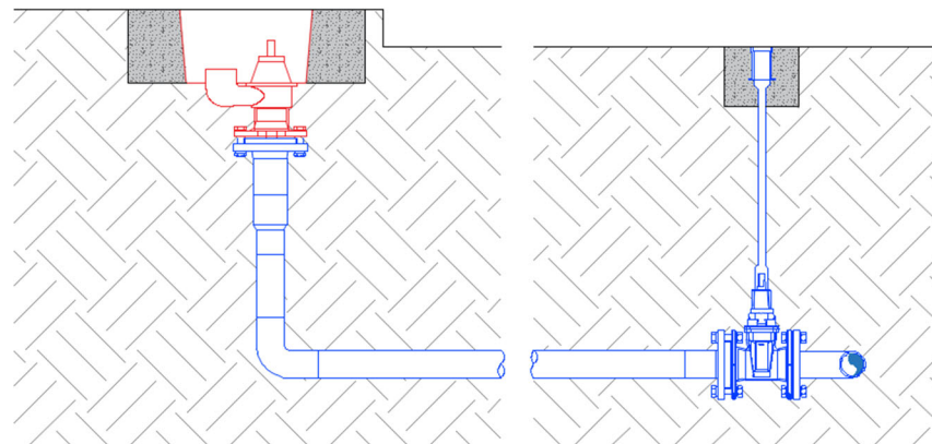
Figura 8. Detall hidrant
