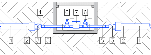
SECCIÓ
