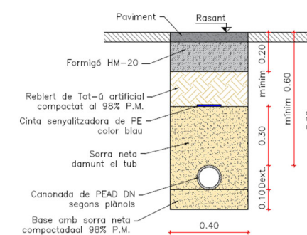
Figura 12. Detall rasa i reposició paviment
