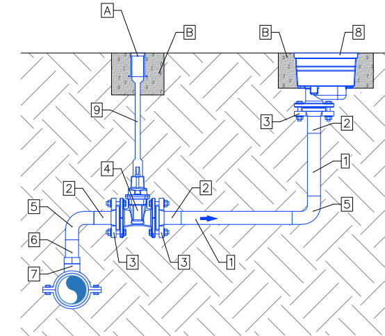
SECCIÓ
