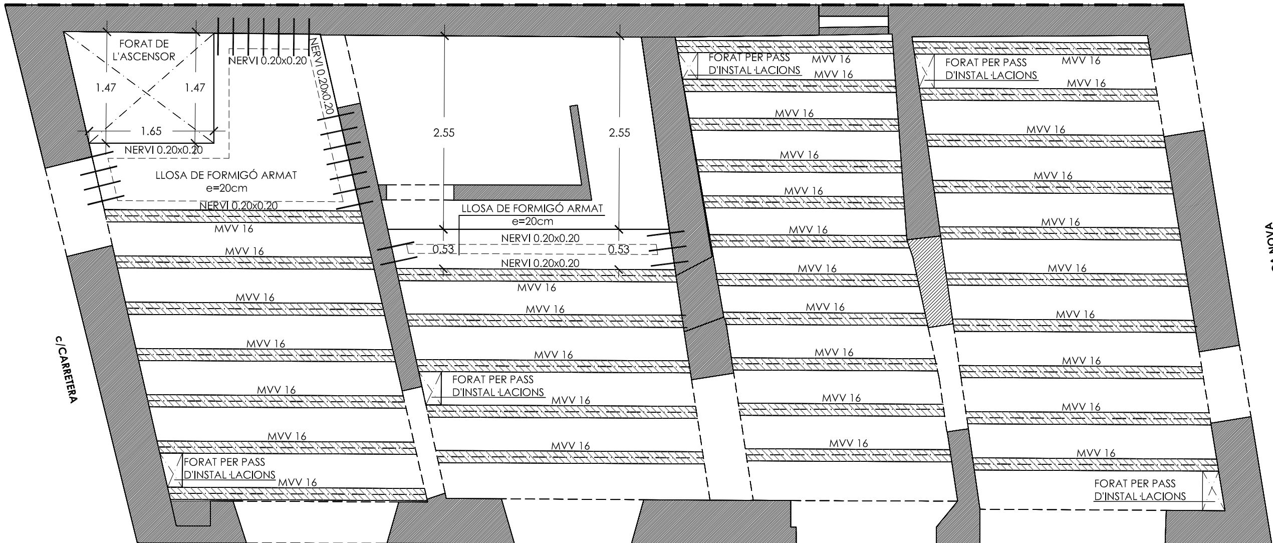
SOSTRE PLANTA BAIXA e:1/50
