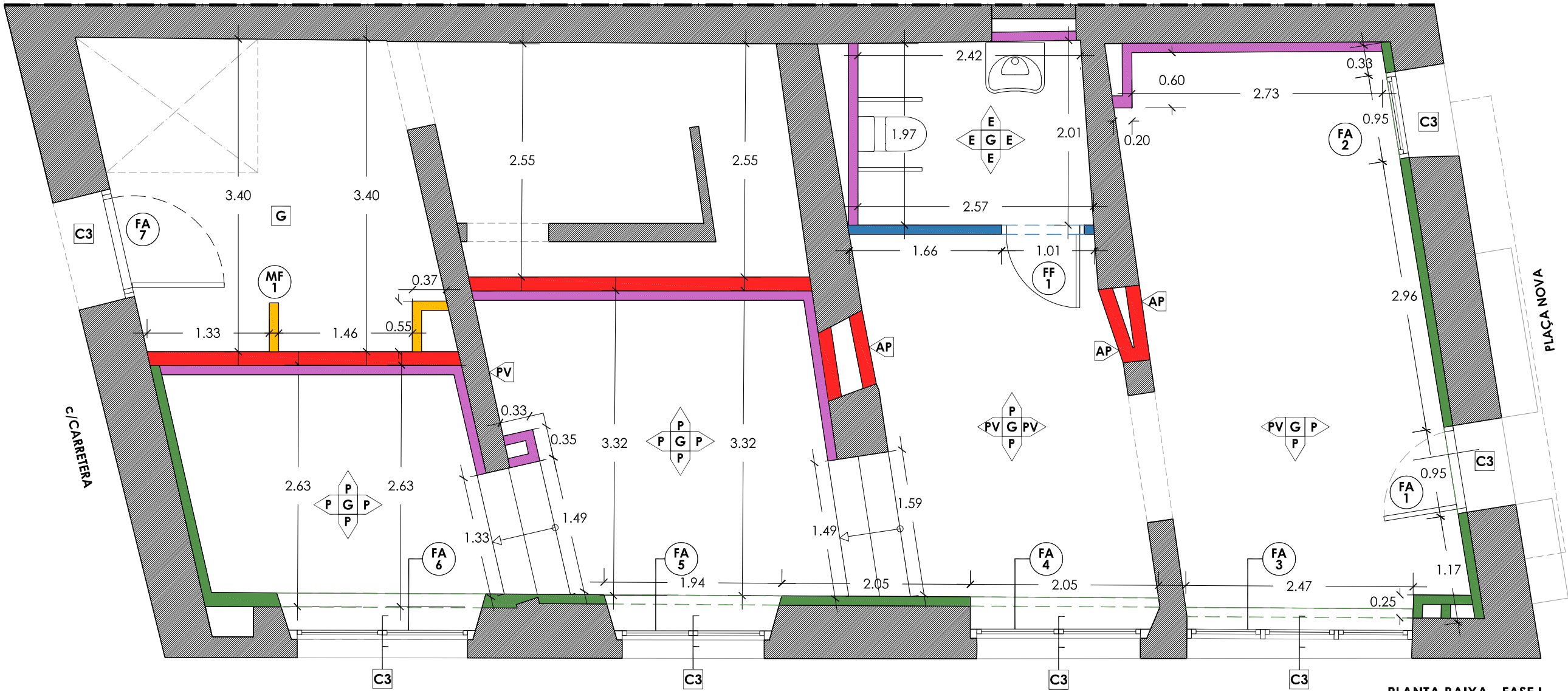
PLANTA BAIXA - FASE I
