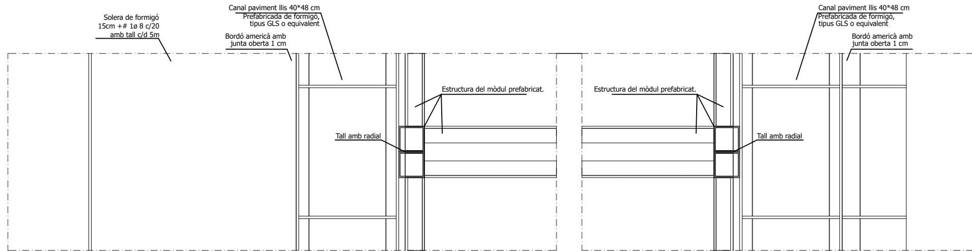
PLANTA A-A'
