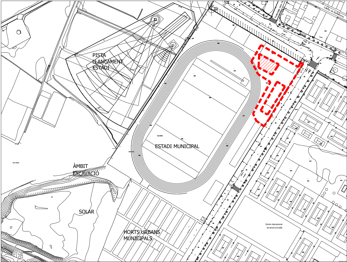
EMPLAÇAMENT
