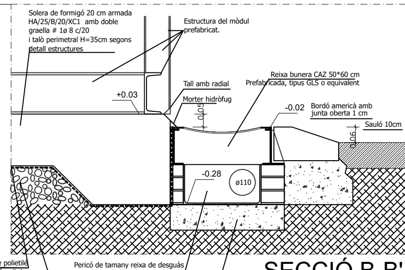
SECCIÓ B-B'
