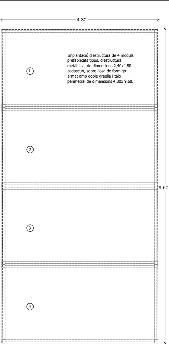
IMPLANTACIÓ MÒDULS PREFABRICATS SOBRE LLOSA DE FORMIGÓ ARMAT e:1/75
