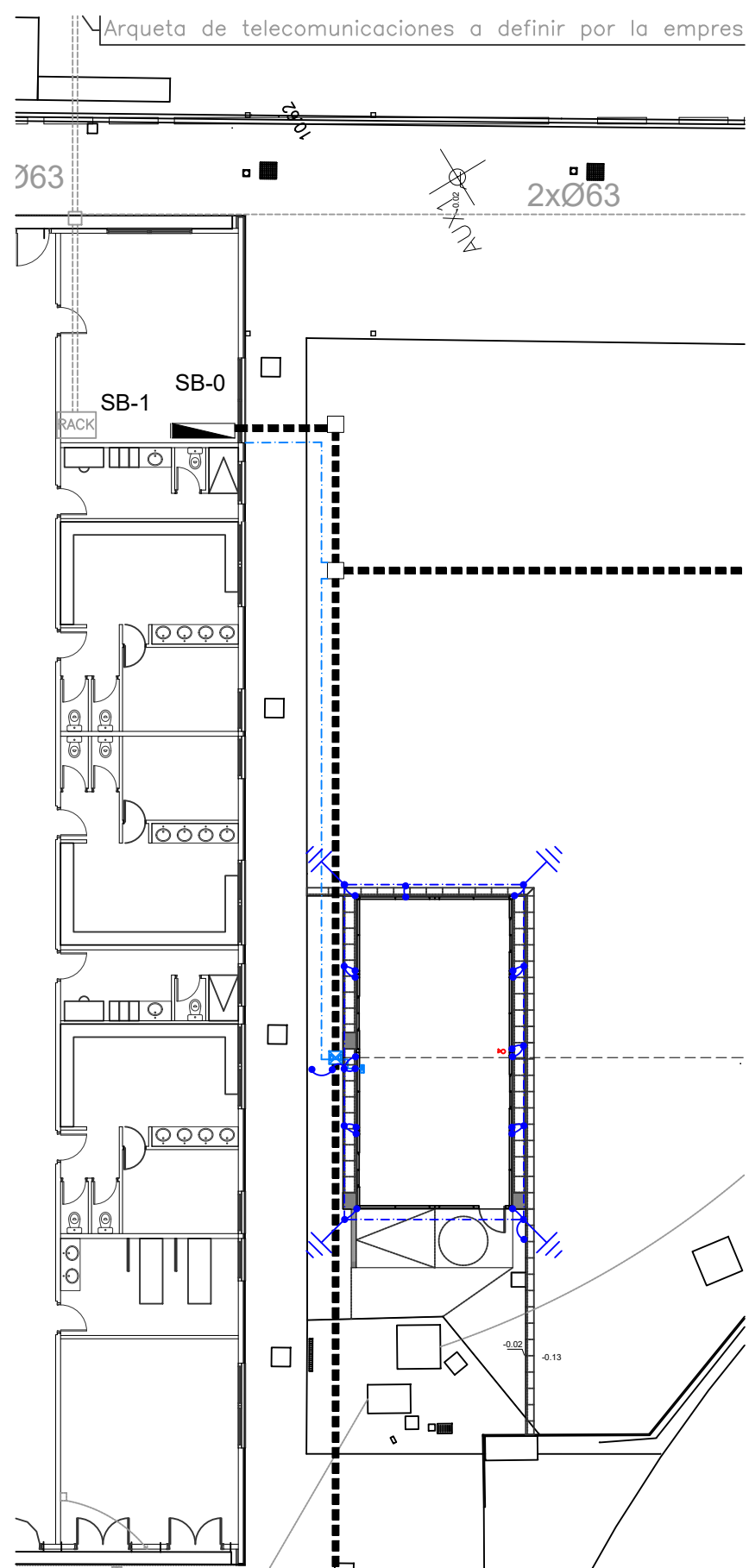
INSTAL·LACIÓ GENERAL I POSTA A TERRA e: 1/200
