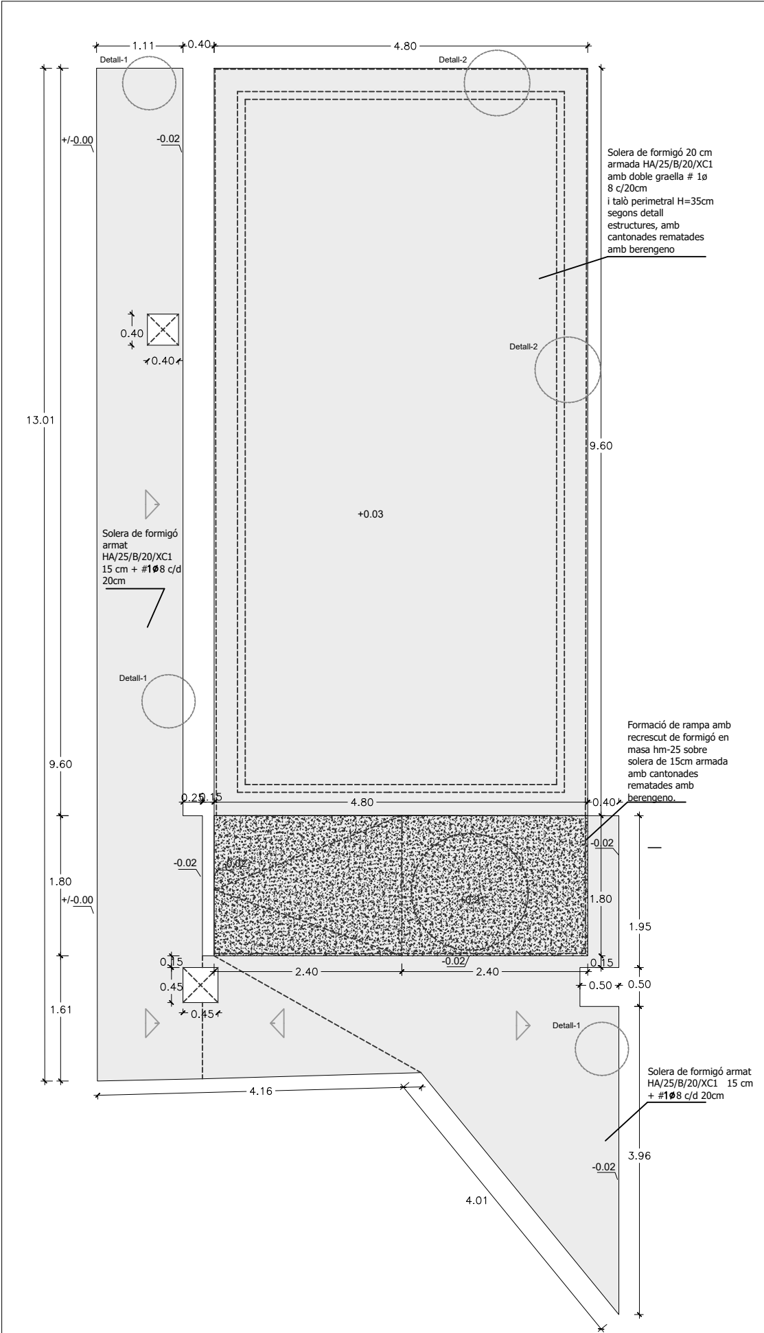
REPLANTEJAMENT DE LLOSA, SOLERES I RECRESQUIT DE RAMPA e:1/75
