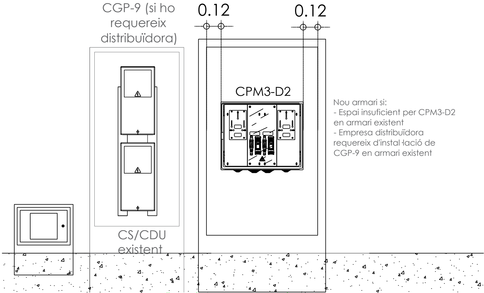
DETALL ALÇAT BB'
