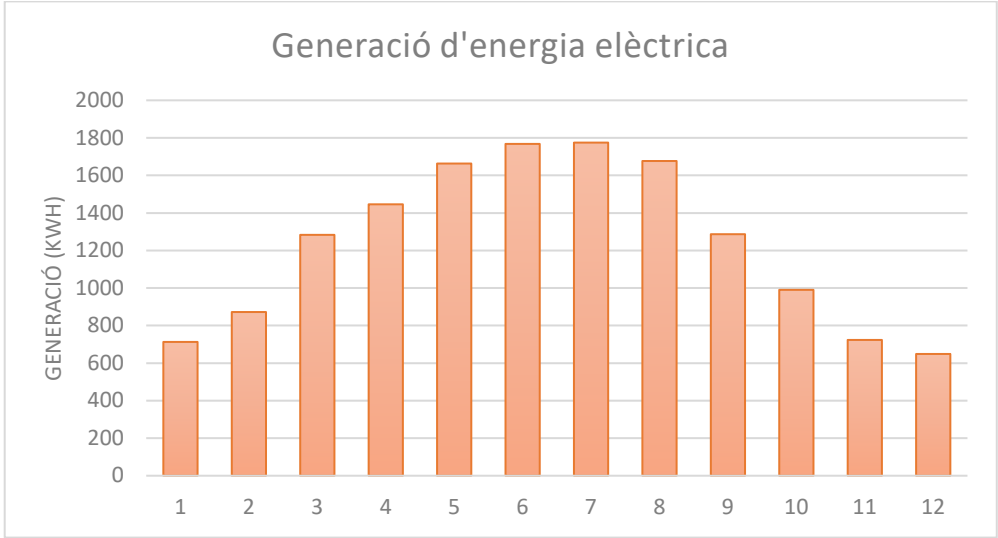
Figura 8 Generació mensual d'energia
