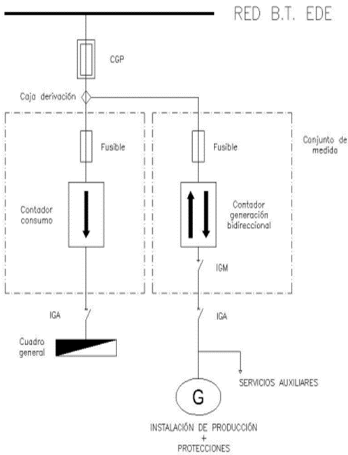
Figura 2 Esquema de connexió amb la xarxa de distribució. NRZ105
