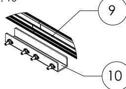
Detail Y 1:10
