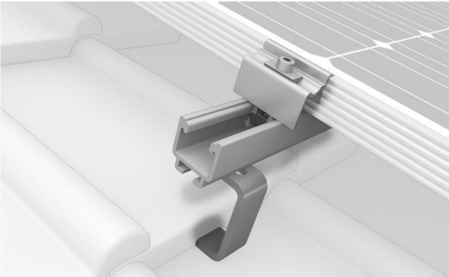
Figura 6 Exemple estructura de suport
