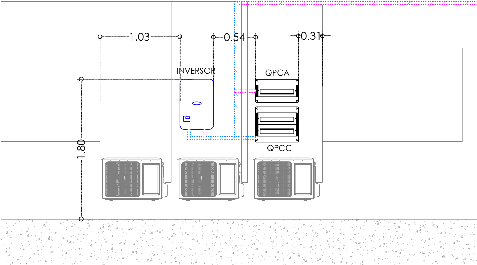
PLANTA AA'
