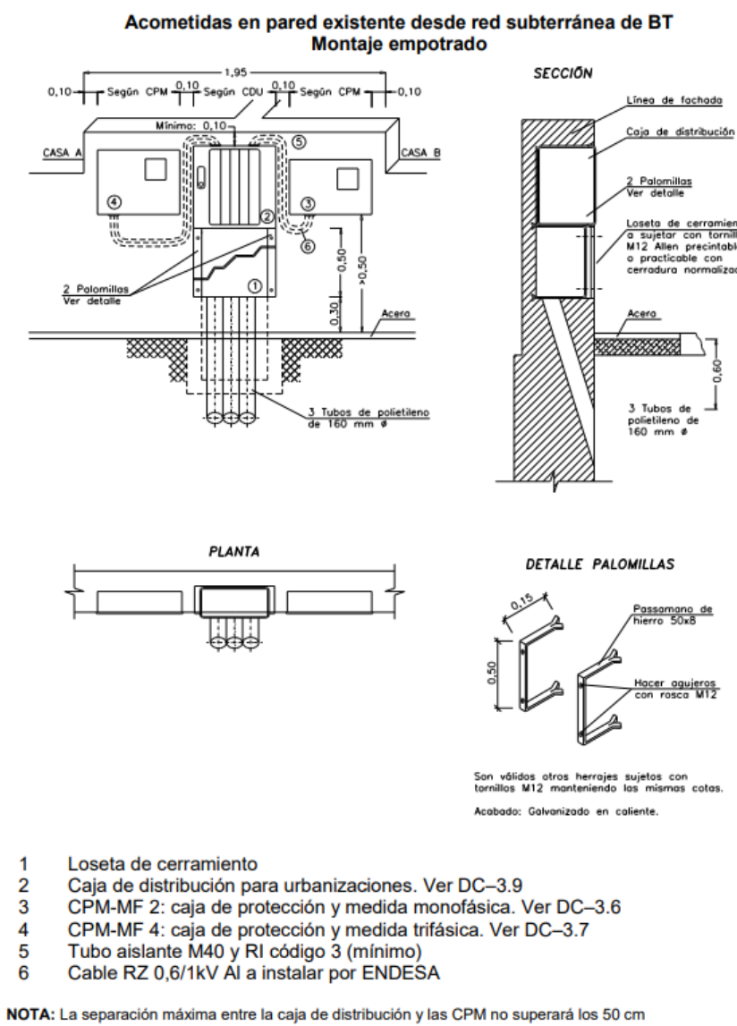
Figura 6 Detall constructiu escomeses en paret existent des de xarxa subterrània de BT - muntatge empotrat. Esquema amb CDU
