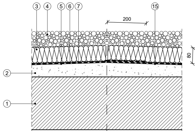
SECCIÓ PEL CARENER Escala (A3) 1/10
