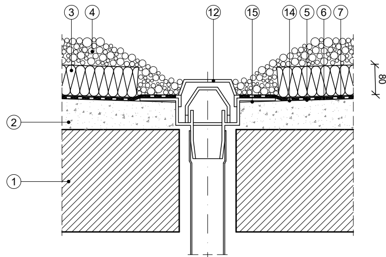
SECCIÓ PEL DESGUÀS Escala (A3) 1/10
