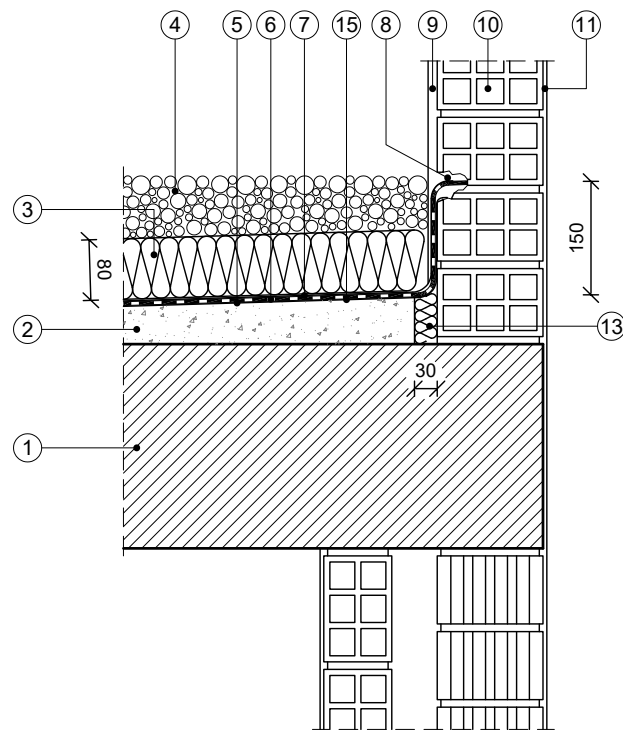
SECCIÓ PER LA VORA Escala (A3) 1/10
