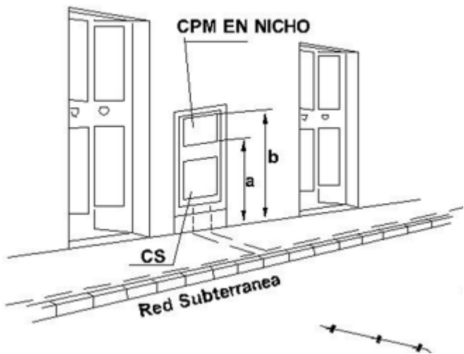
Figura 7 Detall constructiu escomeses en paret existent des de xarxa subterrània de BT - muntatge empotrat. Esquema amb CS
