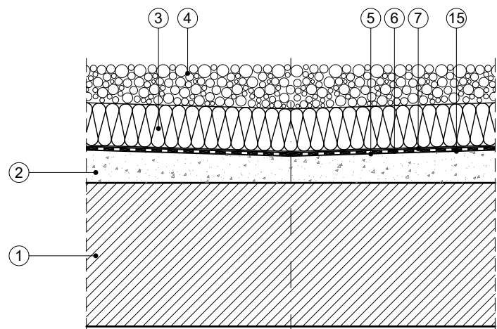
SECCIÓ PEL AIGUAFONS Escala (A3) 1/10
