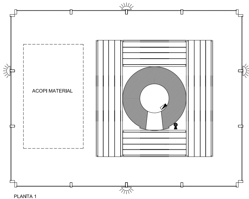
PLANTA 1
