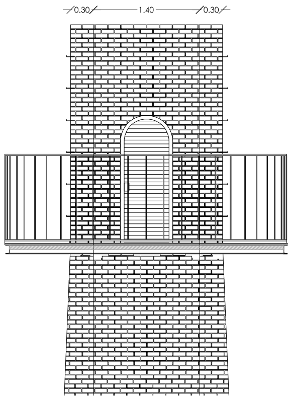
ALÇAT E: 1/50
