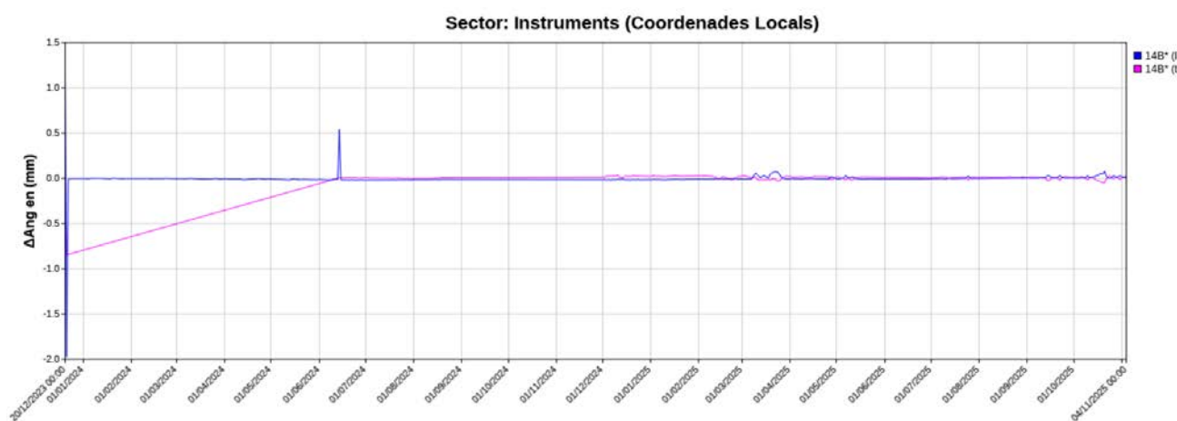
Gràfica dels moviments – Clinòmetre 14B
