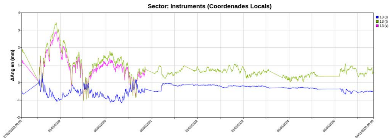
Gràfica dels moviments – Clinòmetre 13
