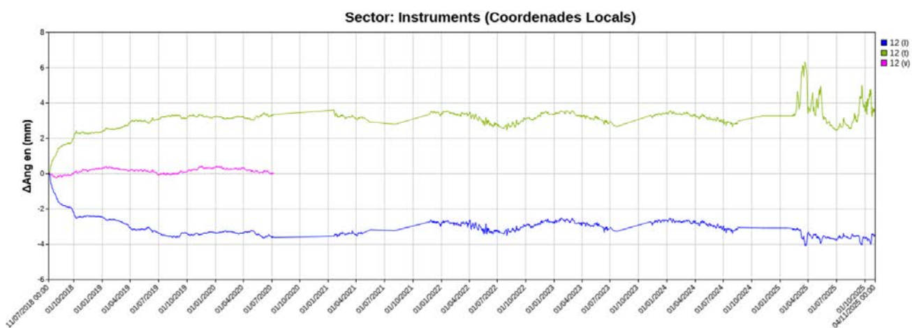
Gràfica dels moviments – Clinòmetre 12
