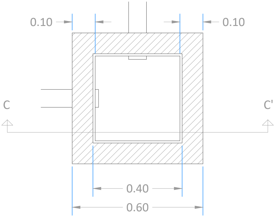
PLANTA
