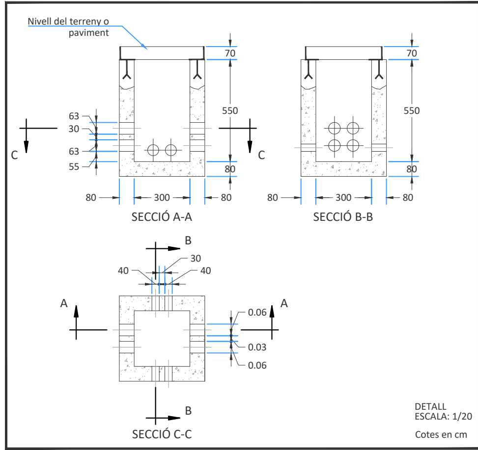
DIMENSIONS DE L'ARQUETA DE FORMIGÓ TIUS M
