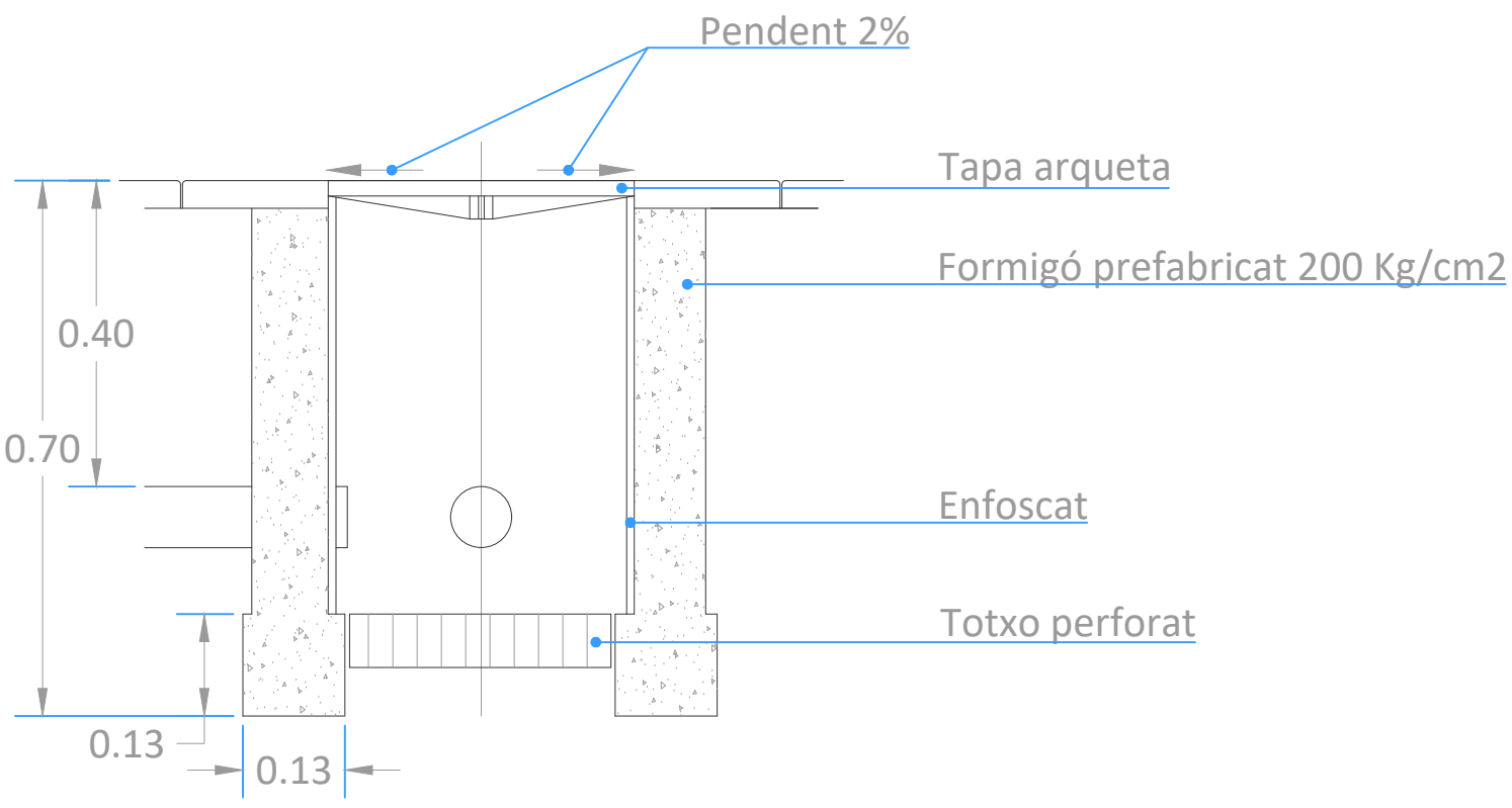
SECCIÓ C - C'
