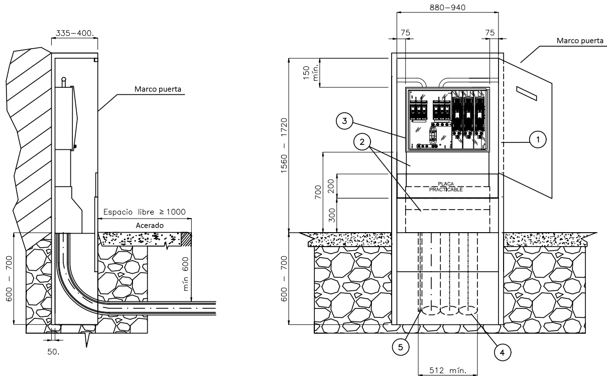
ESQUEMA CAJA SECCIONAMIENTO CON ACOMETIDA PARTE SUPERIOR
