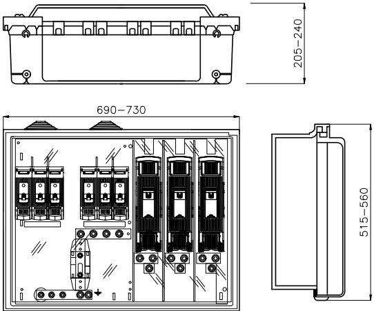
CAJA DISTRIBUCIÓN URBANA (CDU) s/norma informativa CNL004
