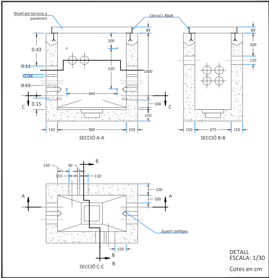
DIMENSIONS DE L'ARQUETA DE FORMIGÓ TIPUS DM
