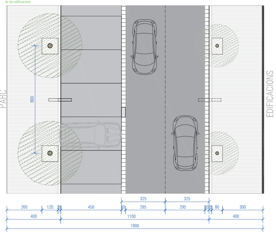
SECCIO TIPUS 1 CARRER REVALL I CARRER DEL RIU
