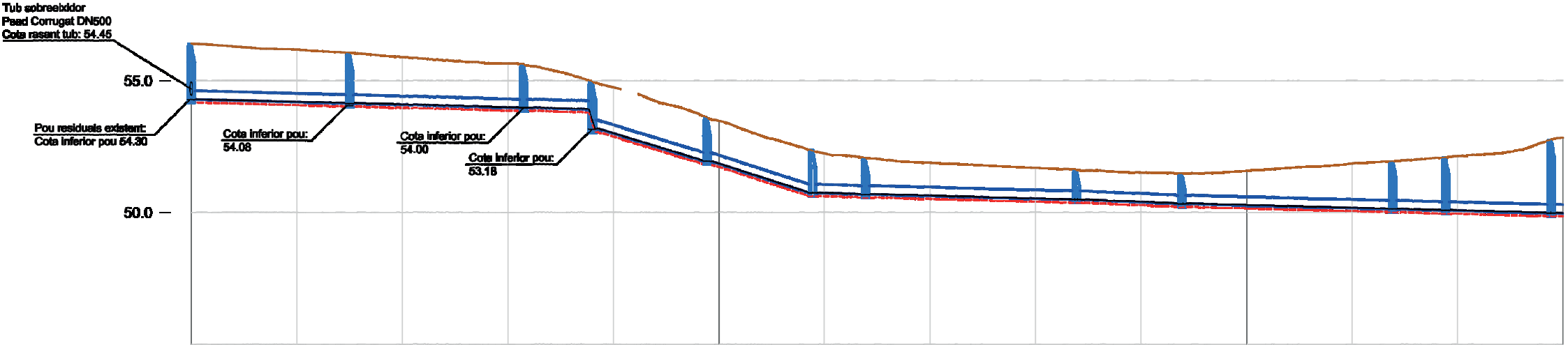
Eix Residuals DN315 Escala H:1000 V: 200
