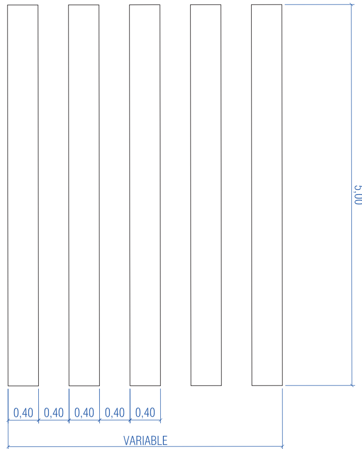
PAS DE VIANANTS SENSE SEMÀFORS
