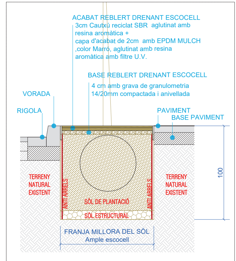
SECCIÓ S1 E:1/25
