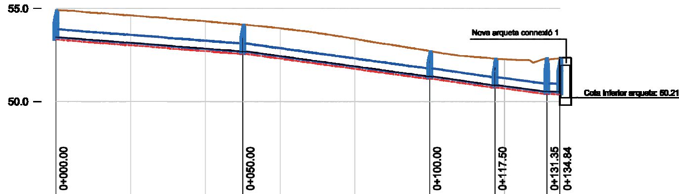
Eix Pluvials Tram 1 Escala H:1000 V: 200
