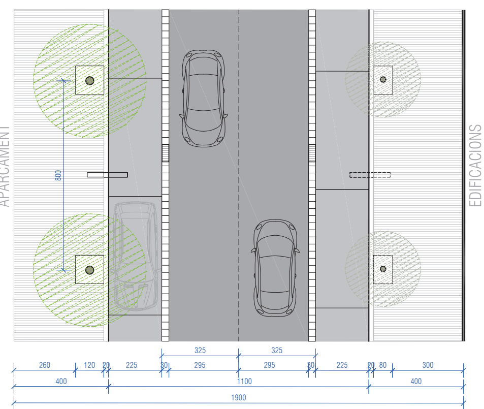
SECCIO TIPUS 2 CARRER DEL RIU
