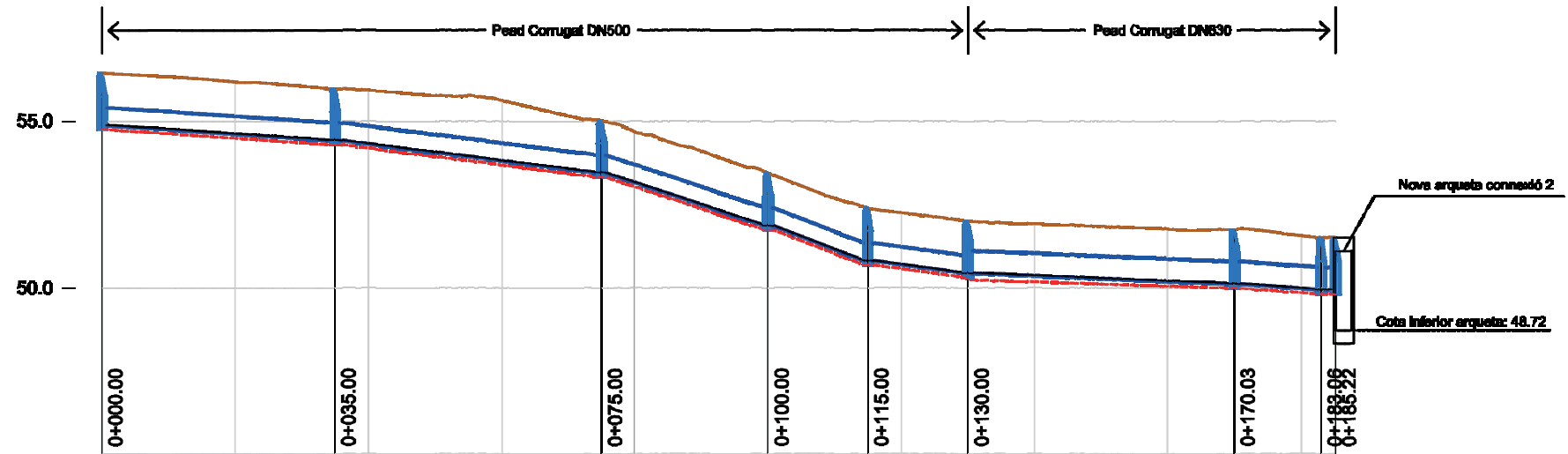
Eix Pluvials Tram 4 Escala: H:1000 V: 200
