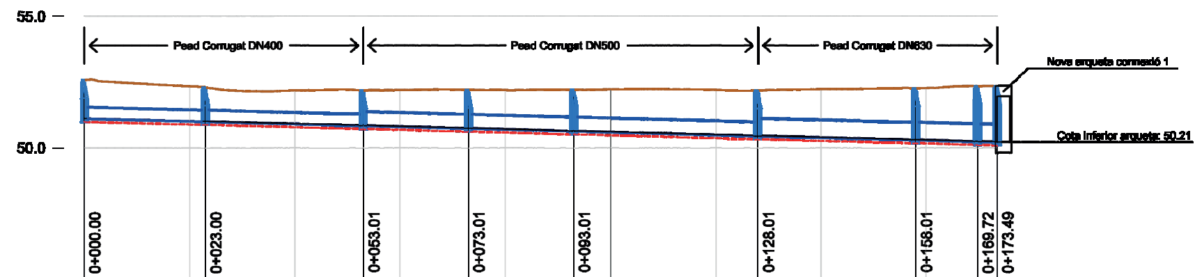
Eix Pluvials Tram 2 Escala H:1000 V: 200
