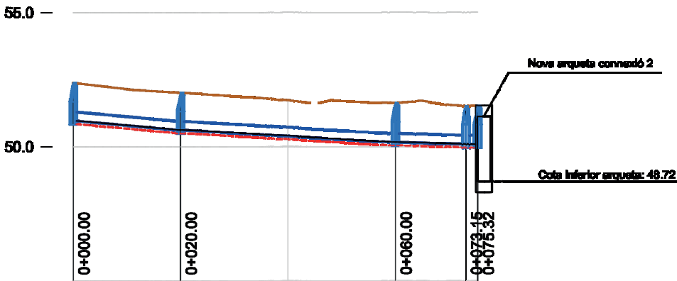
Eix Pluvials Tram 3 Escala: H:1000 V: 200
