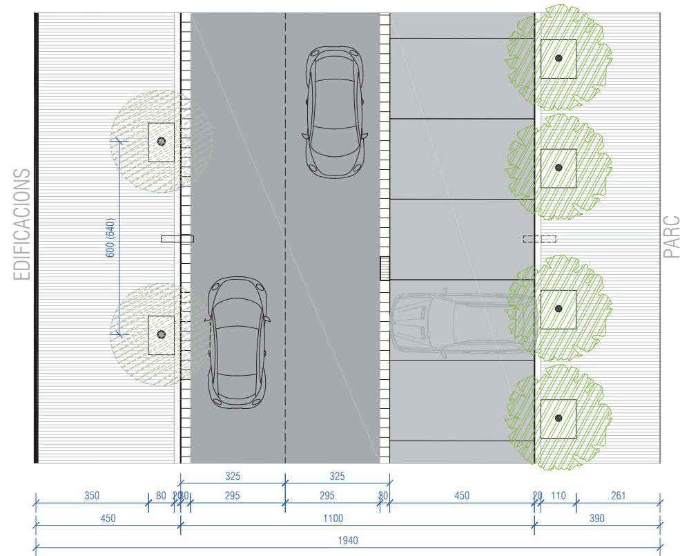
SECCIO TIPUS c/SALVADOR ESPRIU
