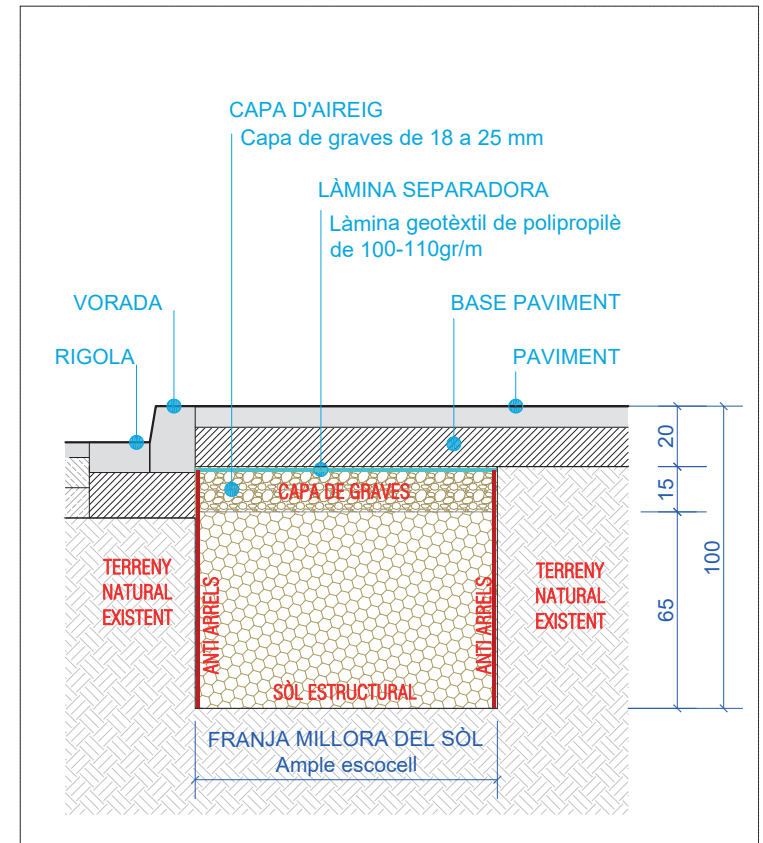
SECCIÓ S2 E:1/25
