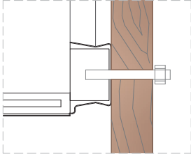
DETALL SUPORT PASSERA DE FLUSTA E:1/3
