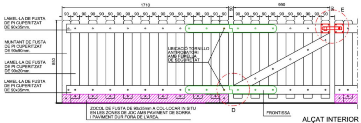
Perfil longitudinal tanca tipus Anglès (vista des d'interior àrea)
