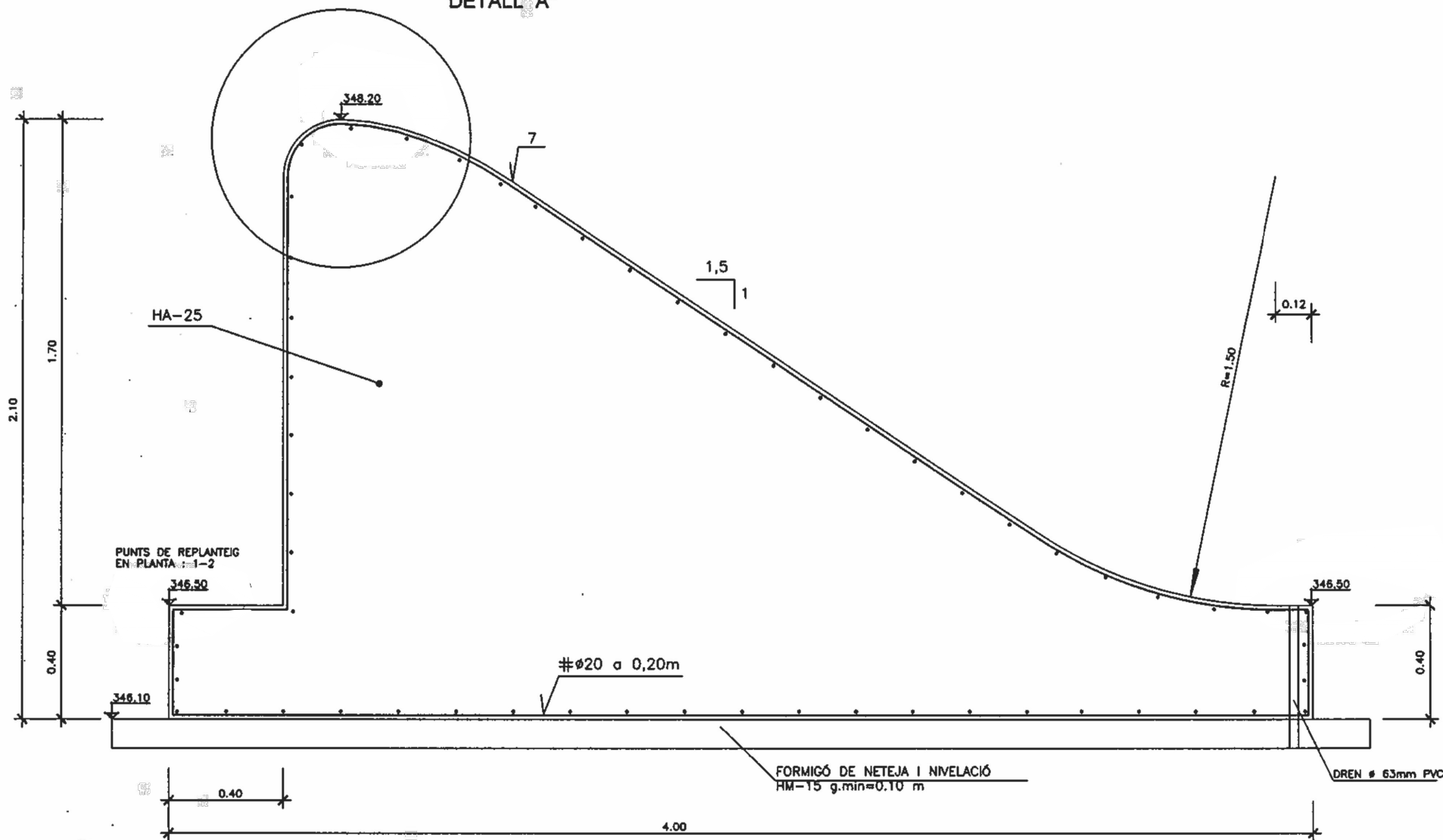
DETALL "A"
