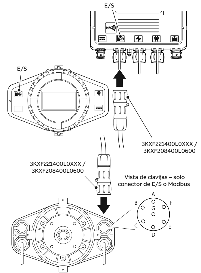
Figura 1 Conexión Modbus
