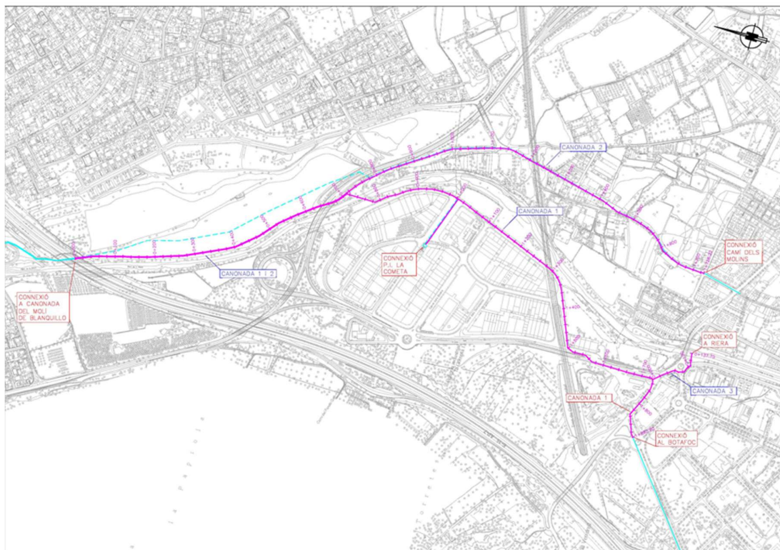
Traçat de les canonades de transport
