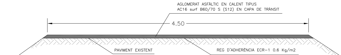
SECCIÓ TIPUS CAMÍ DE SERRATEIX A CASTELLADRAL (DIVERSOS TRAMS)
