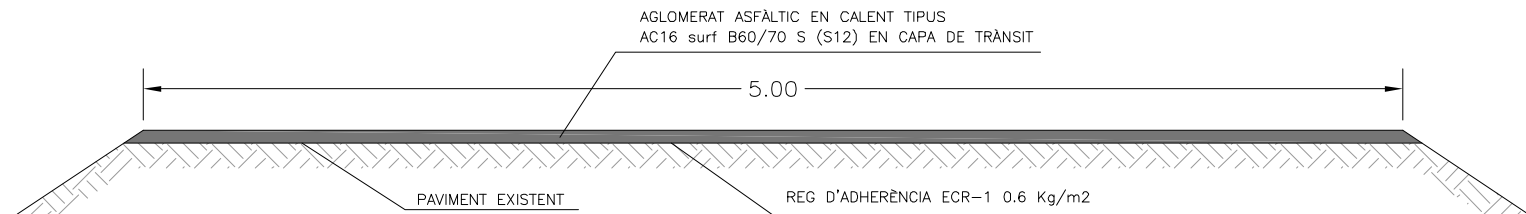
SECCIÓ TIPUS CAMÍ DE VIVER A PUIG-REIG (DIVERSOS TRAMS)
