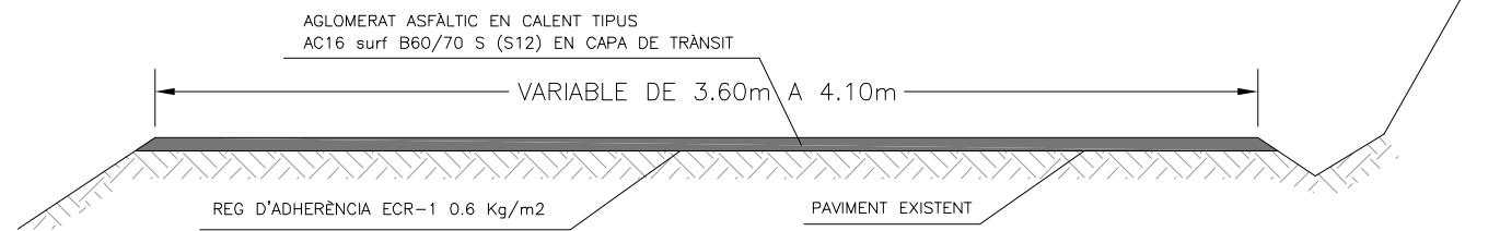
SECCIÓ TIPUS CAMÍ DE SERRATEIX A CARDONA (DIVERSOS TRAMS)
