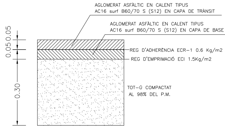
DETALL FERM ZONA FLONJALLS I ARRELS (Camí de Serrateix a Cardona)
