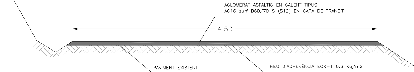
SECCIÓ TIPUS CAMÍ DE VIVER A SANT JOAN DE MONTDARN (DIVERSOS TRAMS)
