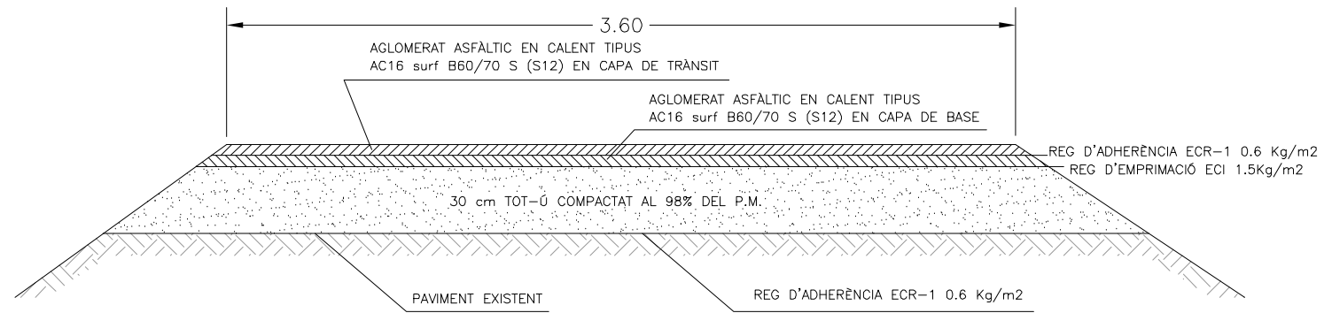
SECCIÓ TIPUS CAMÍ DE SERRATEIX A CARDONA (ZONA DE FLONJALLS I ARRELS)
