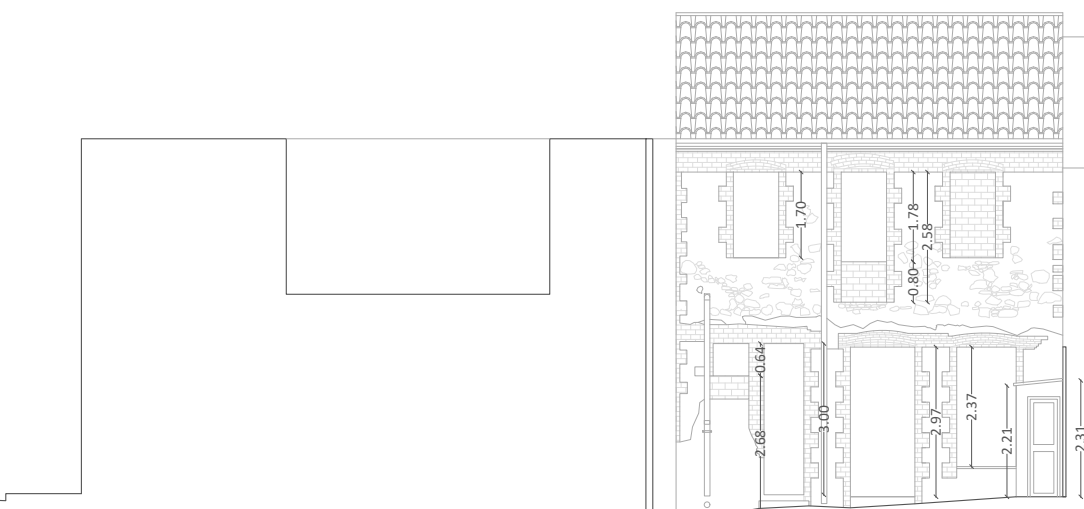
ALÇAT FAÇANA INTERIOR CASA
