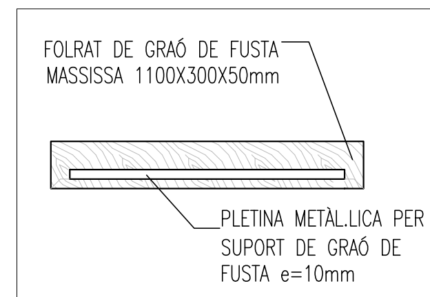
DETALL GRAÓ EN TRAM D'ESCALA DE PLANTA BAIXA A PLANTA PRIMERA
