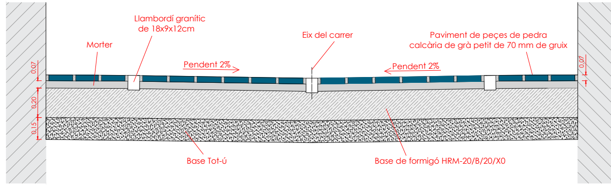
Detall secció A-A'
