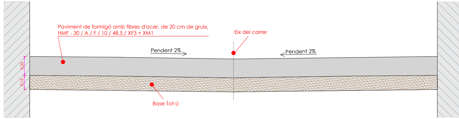
Detall secció A-A' e. 1/25
