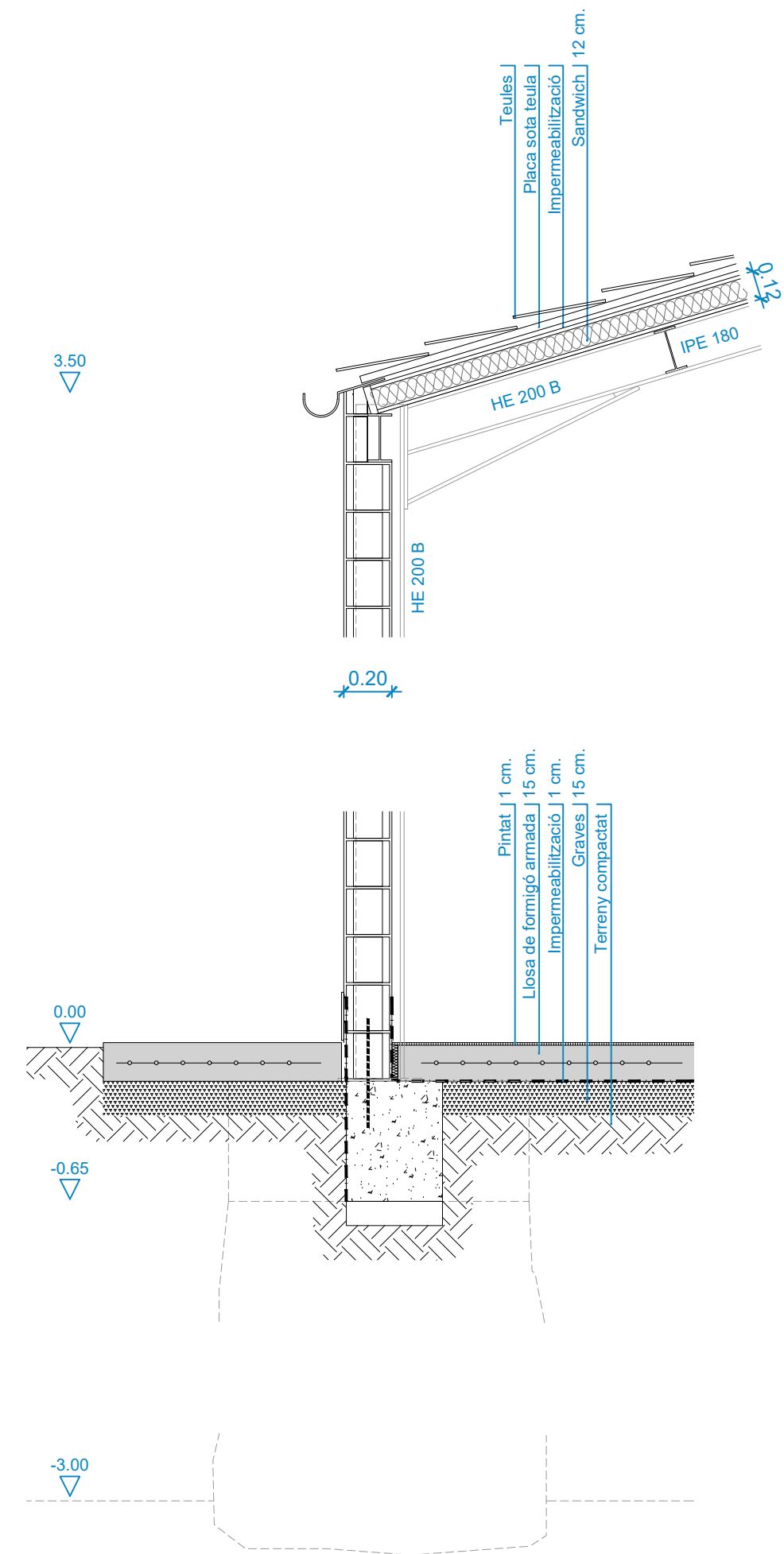
SECCIÓ DETALL
