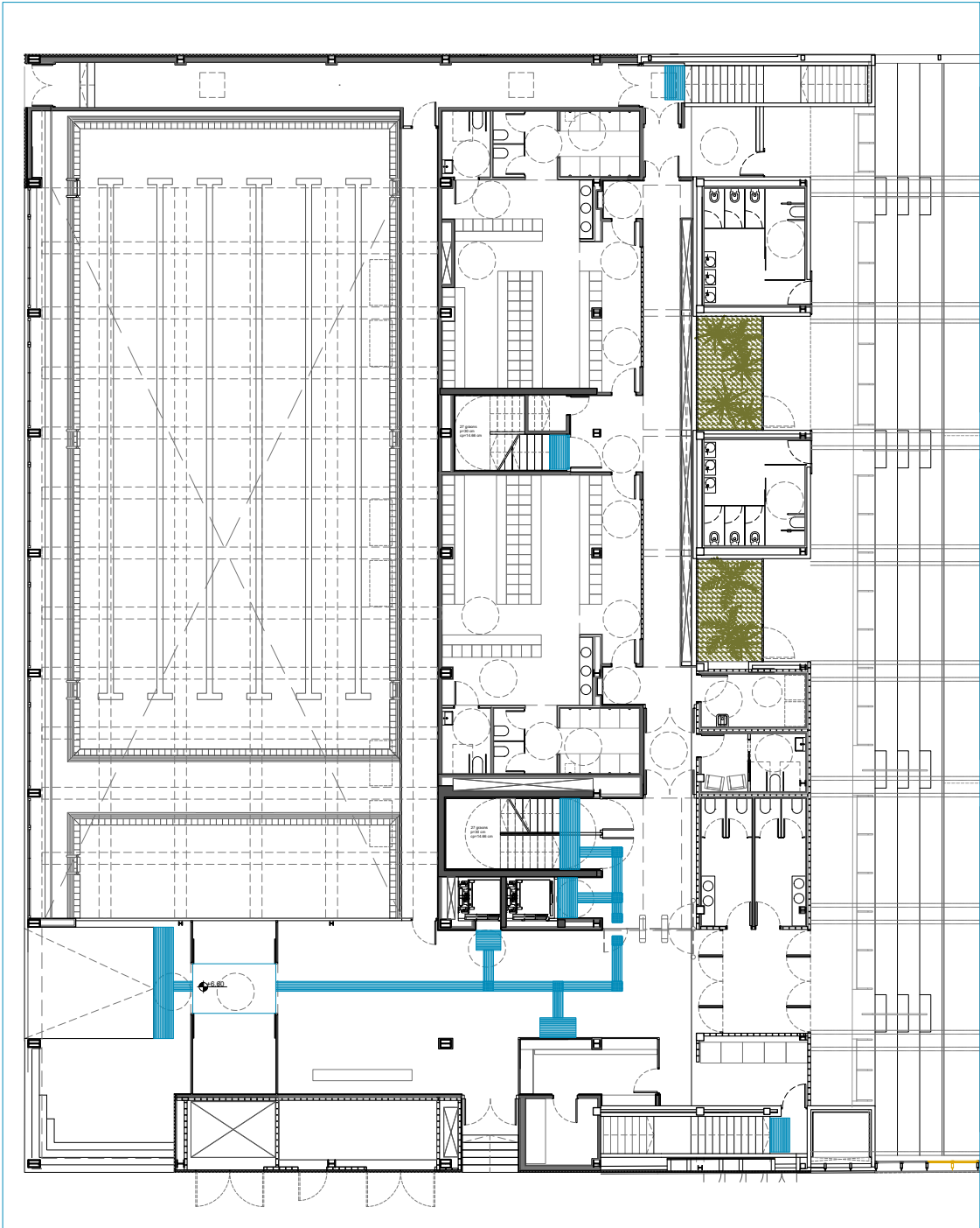
PLANTA BAIXA
