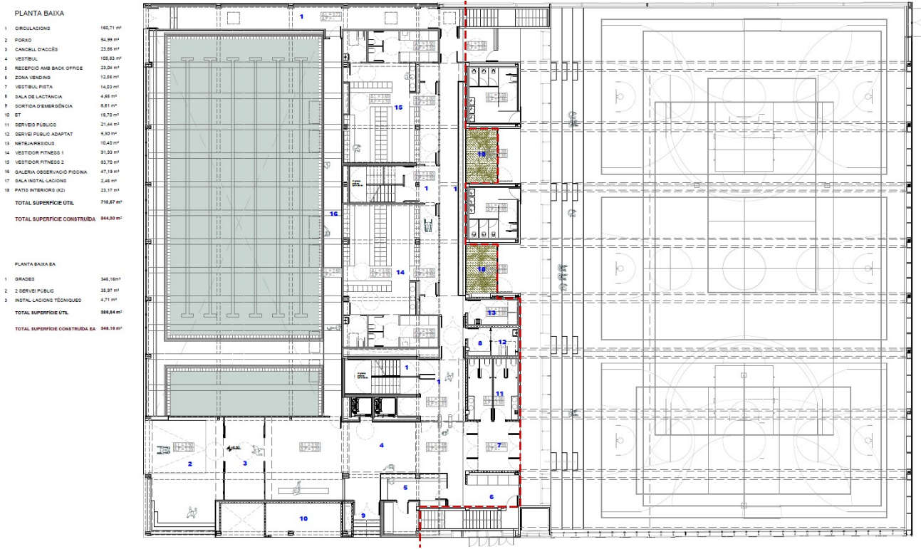
Planta baixa
