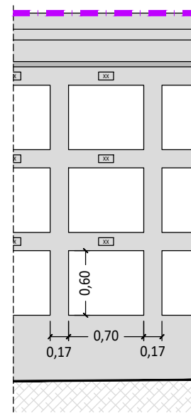
ALÇATS TIPUS
