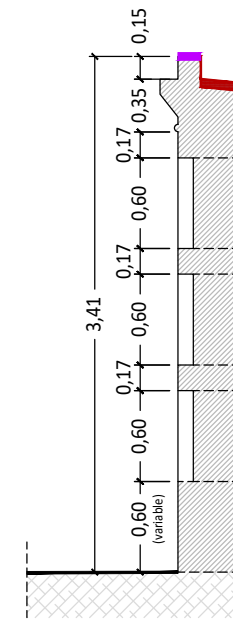
SECCIÓ TIPUS
