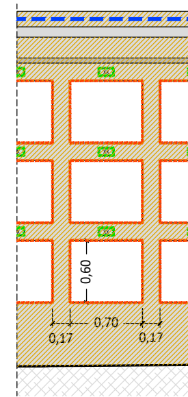
ALÇATS TIPUS
