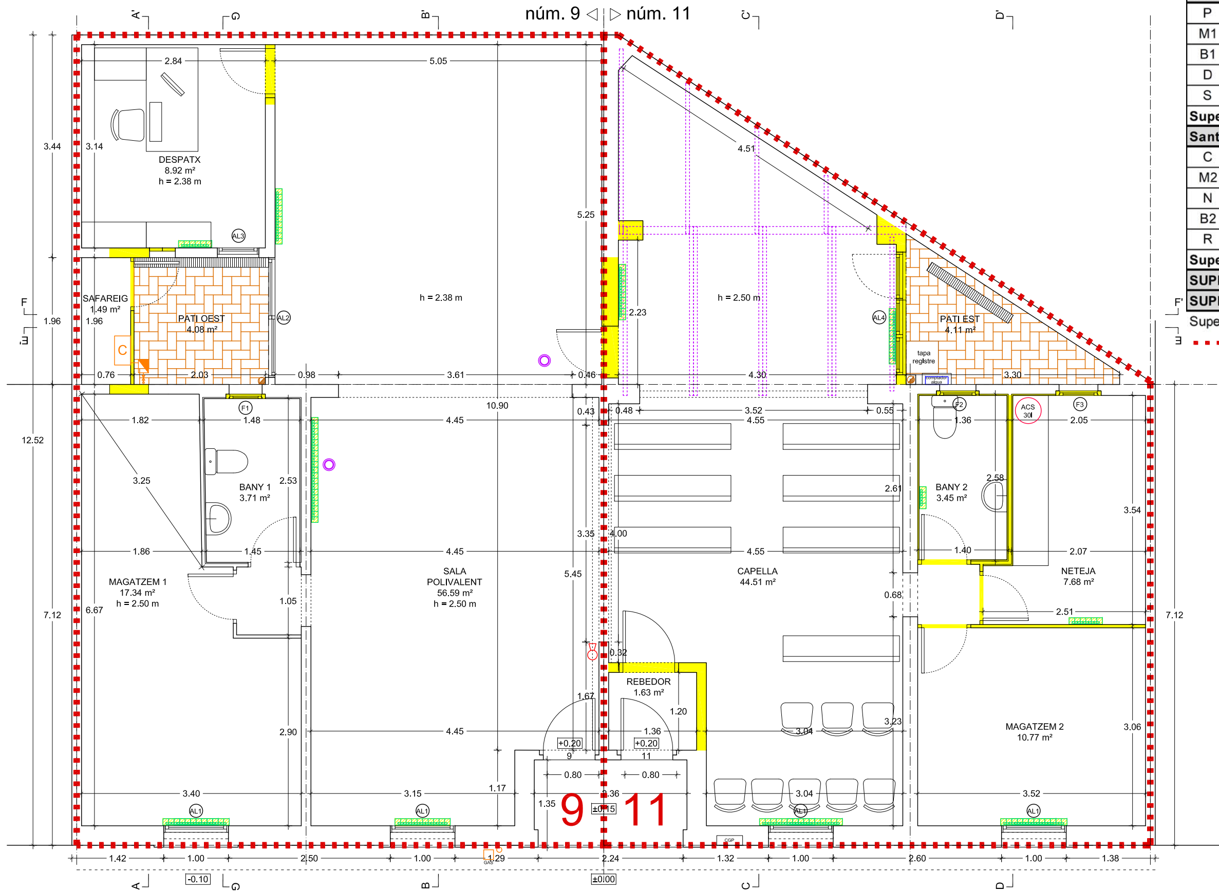
PLANTA BAIXA
