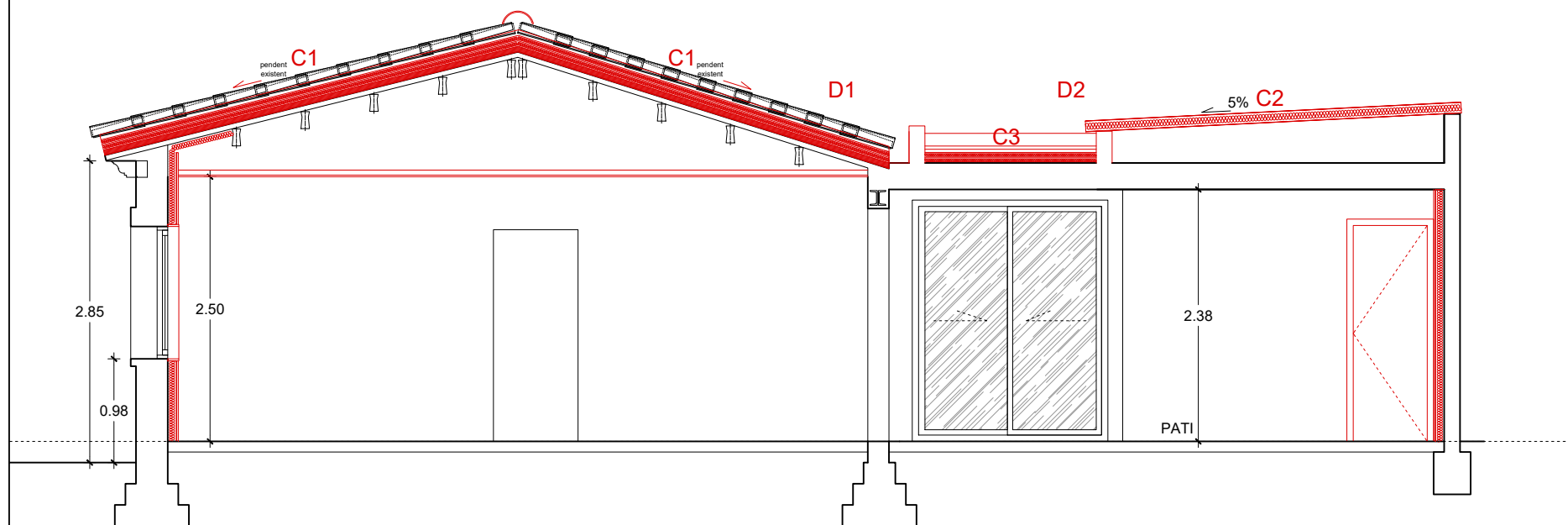
SECCIÓ TRANSVERSAL B-B'
