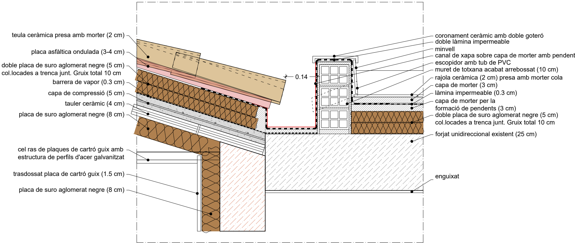
DETALL 1 TROBADA C1-C3
