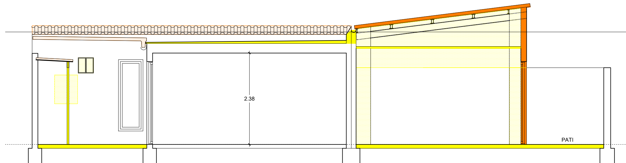
SECCIÓ LONGITUDINAL F-F'
