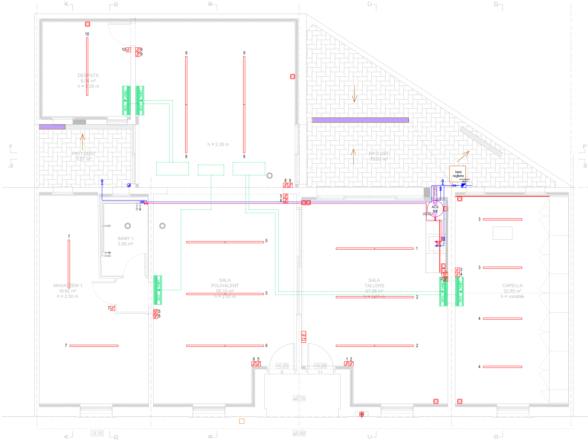
PLANTA BAIXA
