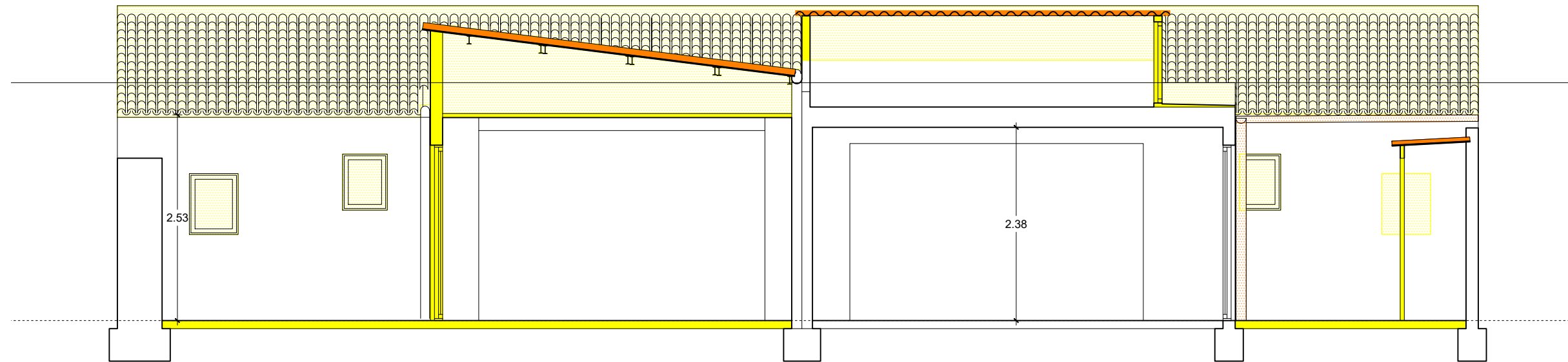
SECCIÓ LONGITUDINAL E-E'
