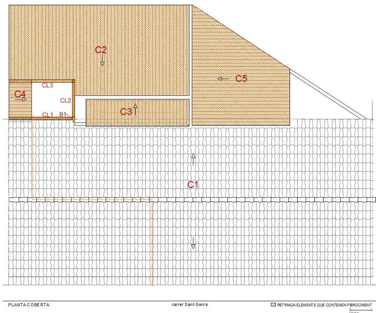
Fig. 1: estat actual de les cobertes dels edificis del carrer Sant Genís 9 i 11 i localització dels elements de fibrociment que contenen amiant.
