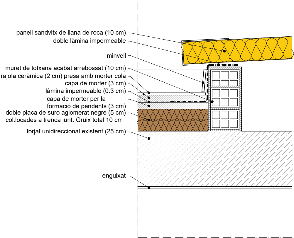
DETALL 2 TROBADA C3-C2
