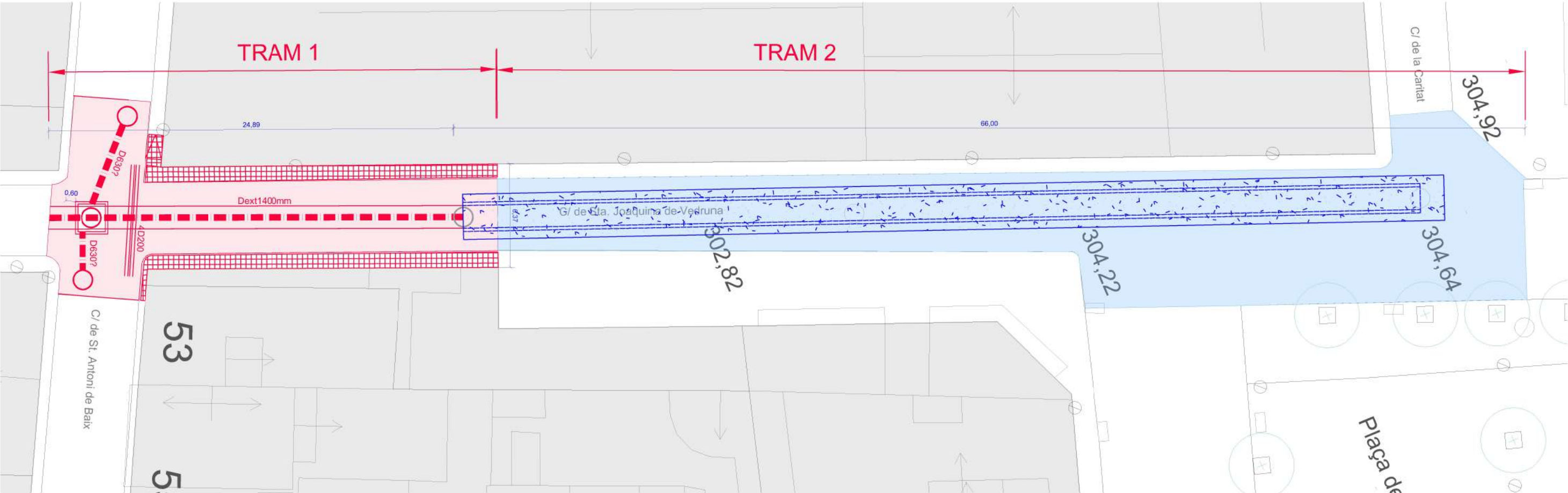
PLANTA E. 1/250
