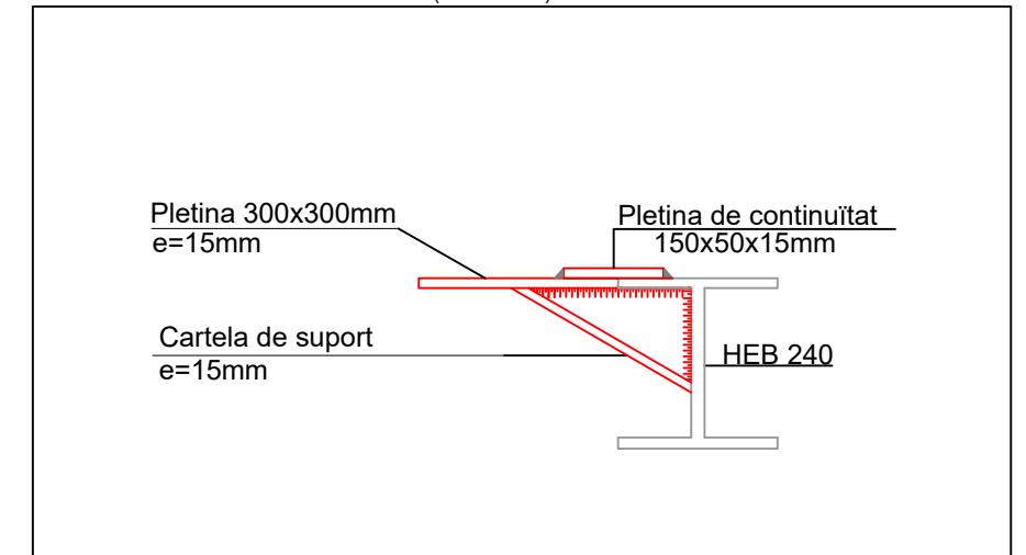
DETALL 2. SUPORTS BOMBA DE CALOR (4 UNITATS). ESCALA 1:125
