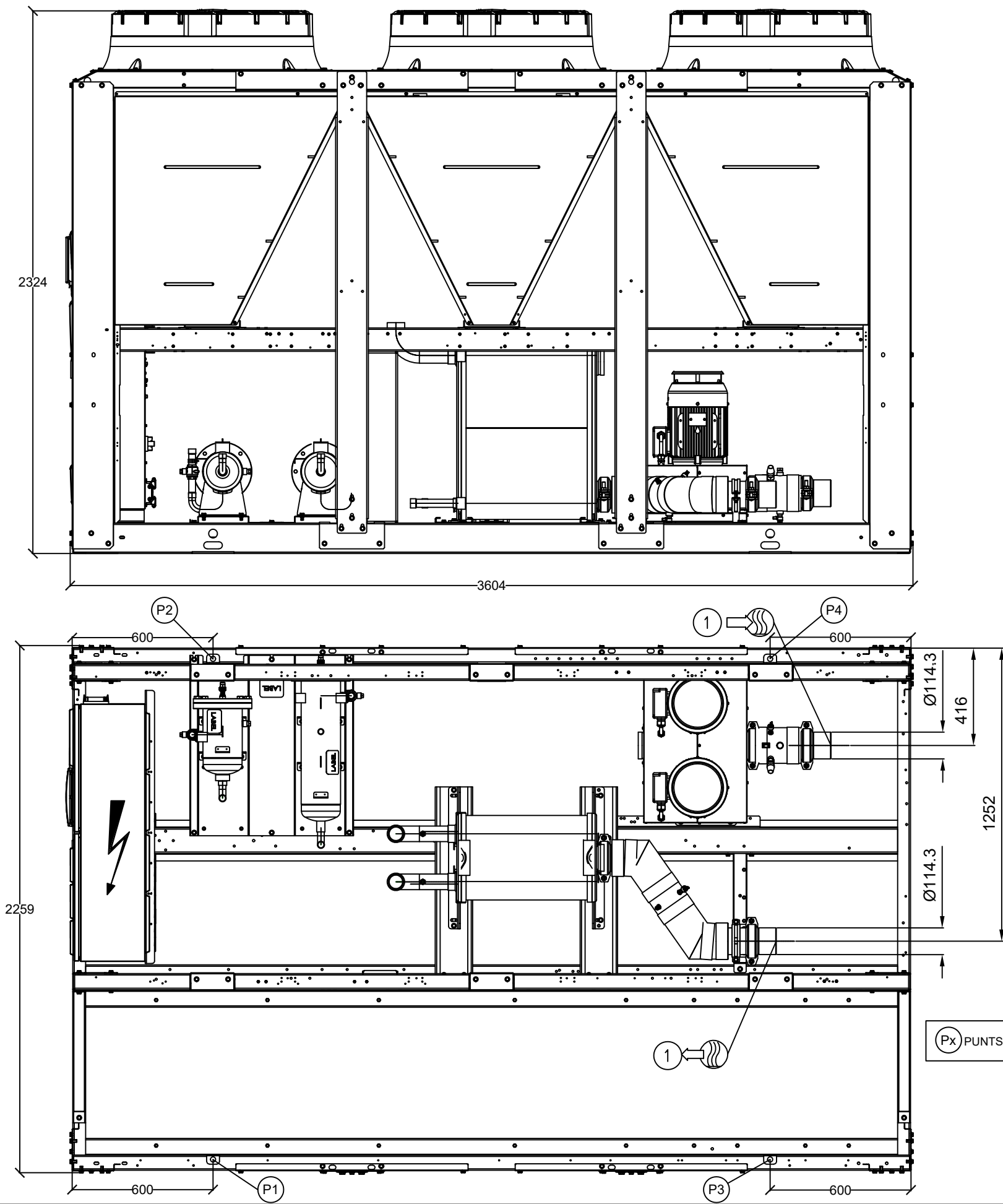
BOMBA DE CALOR TIPUS. CARRIER model 30RQP 370R
