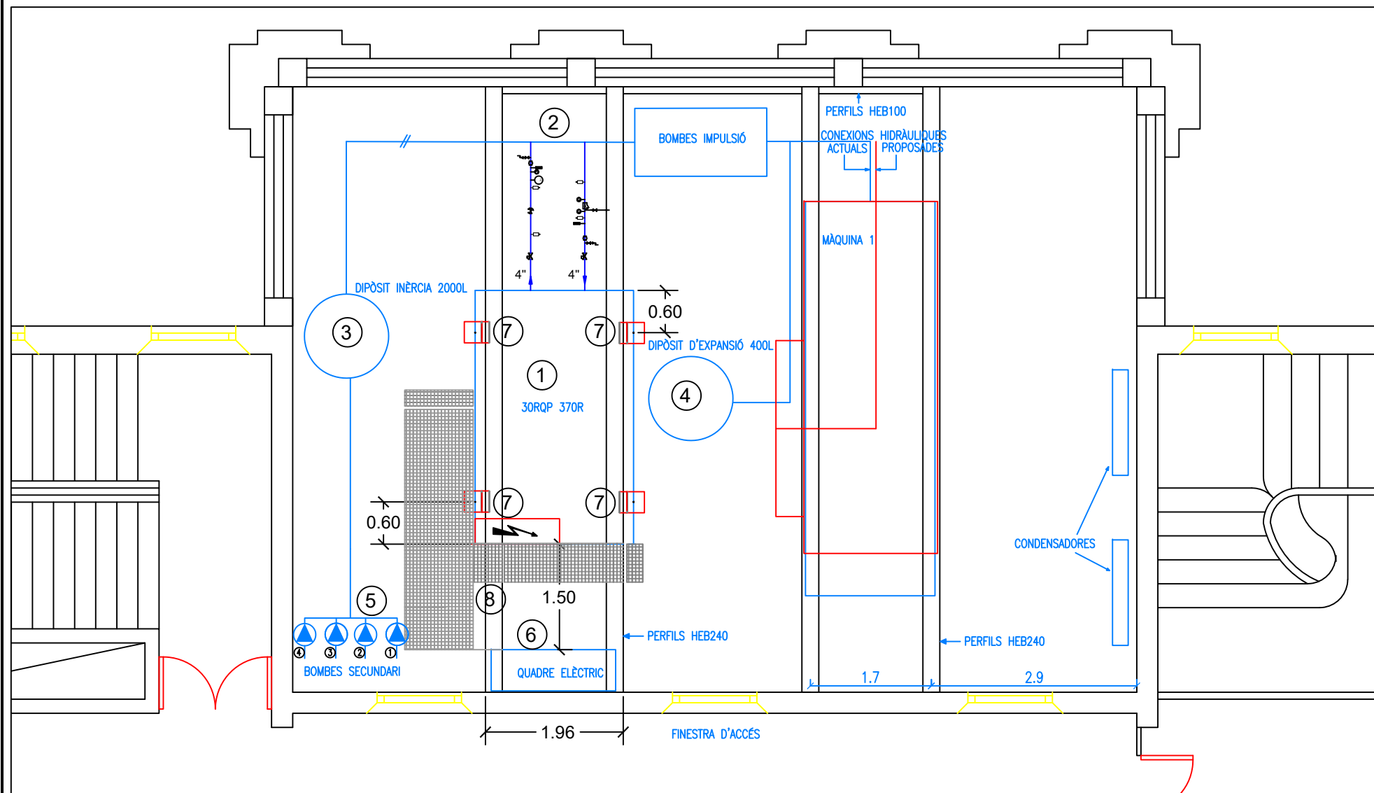
DETALL 2. SUPORTS BOMBA DE CALOR (4 UNITATS). ESCALA 1:125
