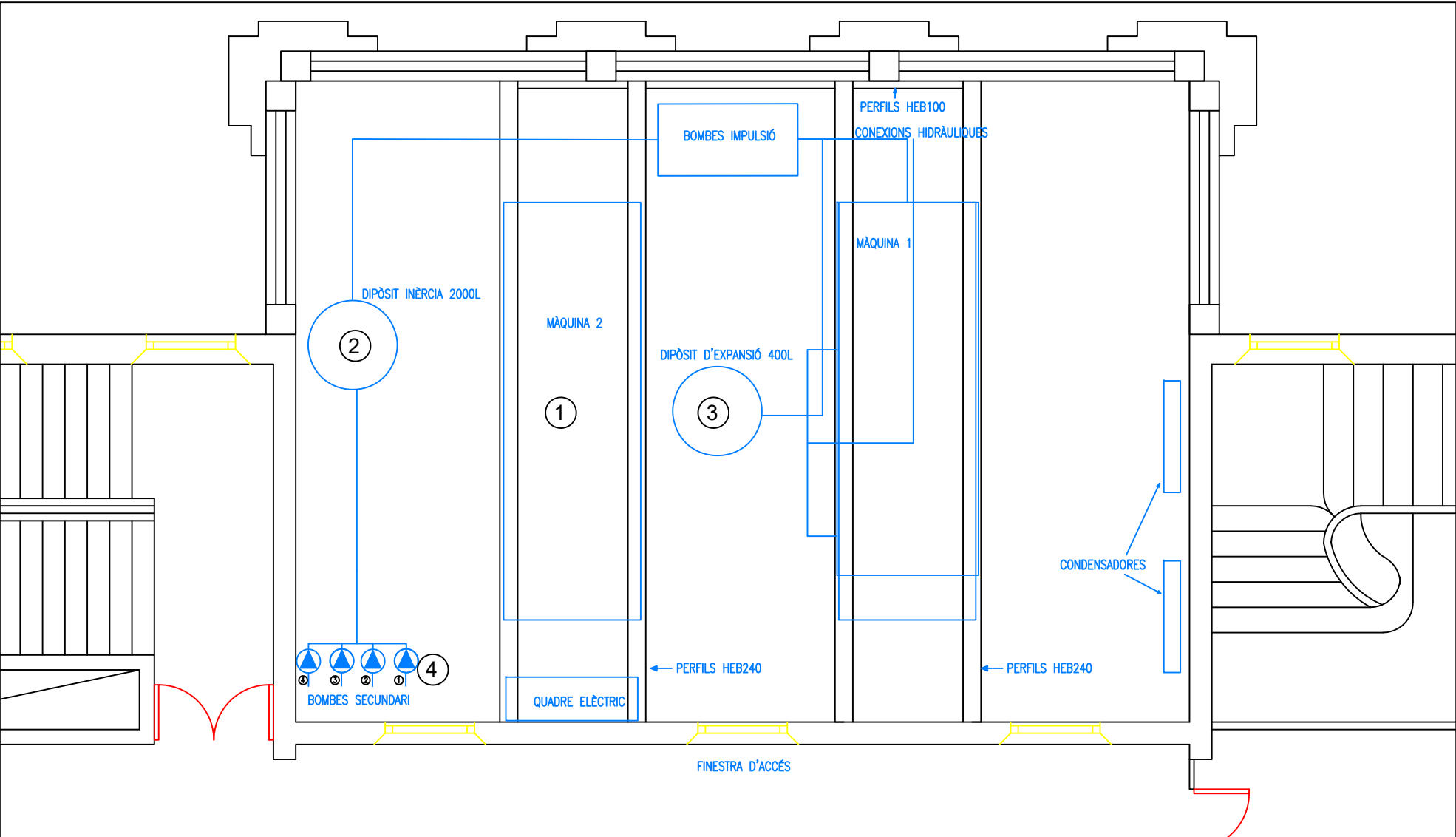
SITUACIÓ ACTUAL. ESCALA 1:75
