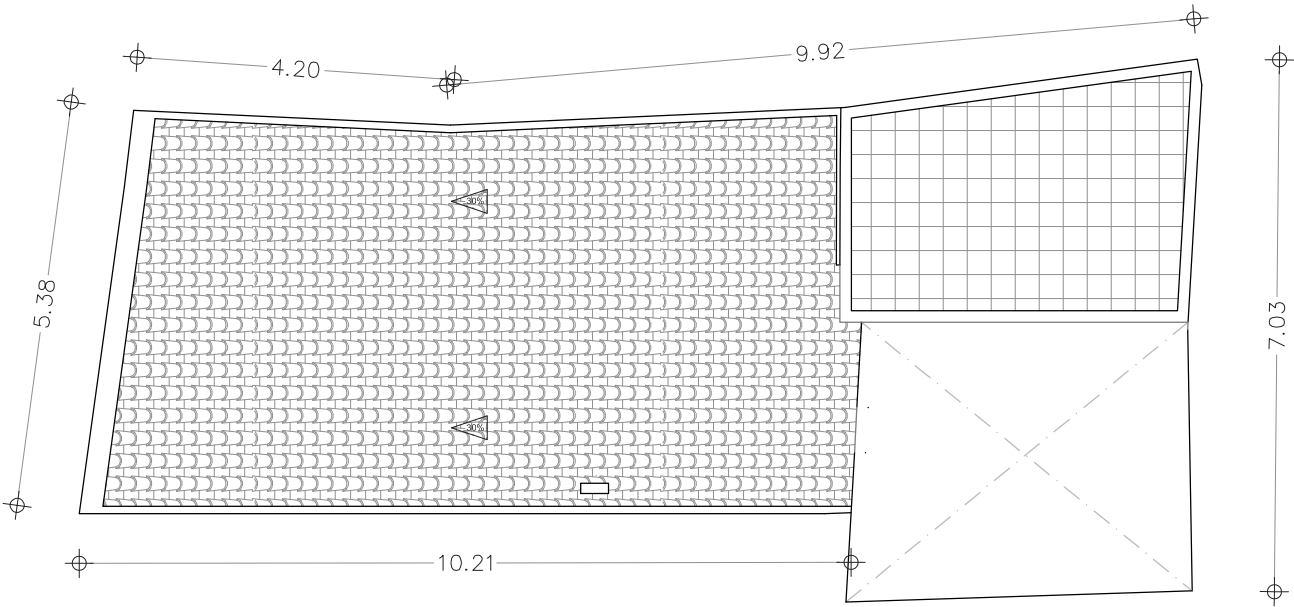
planta sotacoberta
