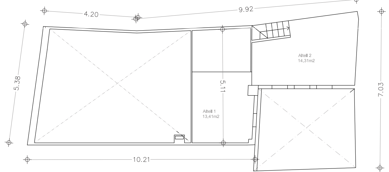
planta sotacoberta
