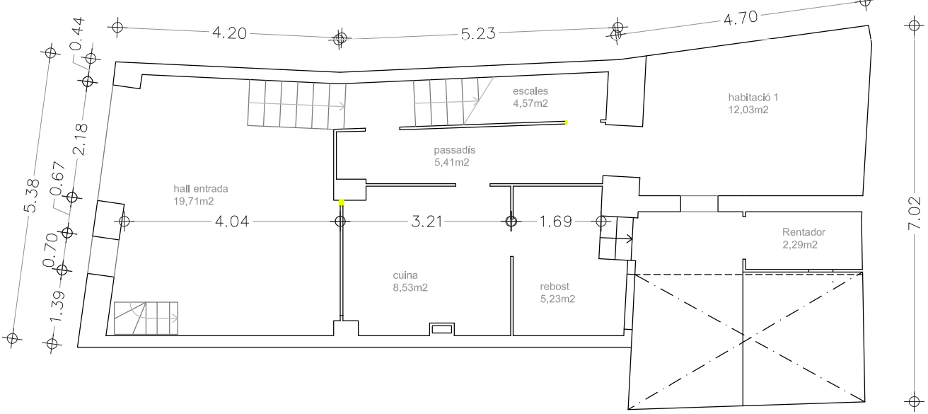
planta entresol
