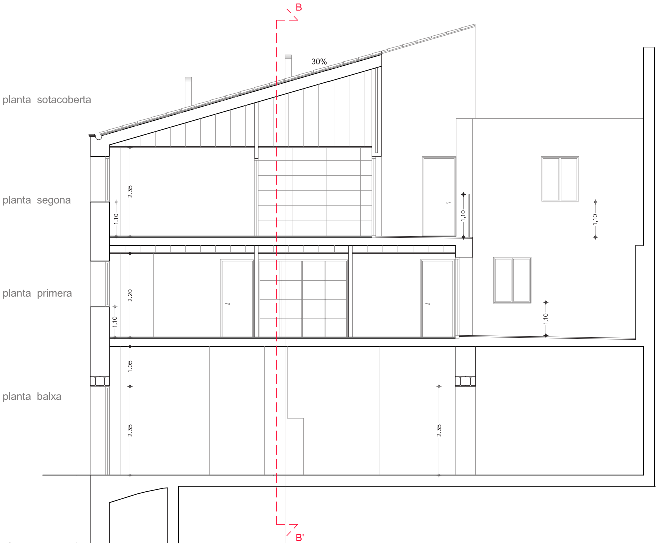
Secció B-B'
