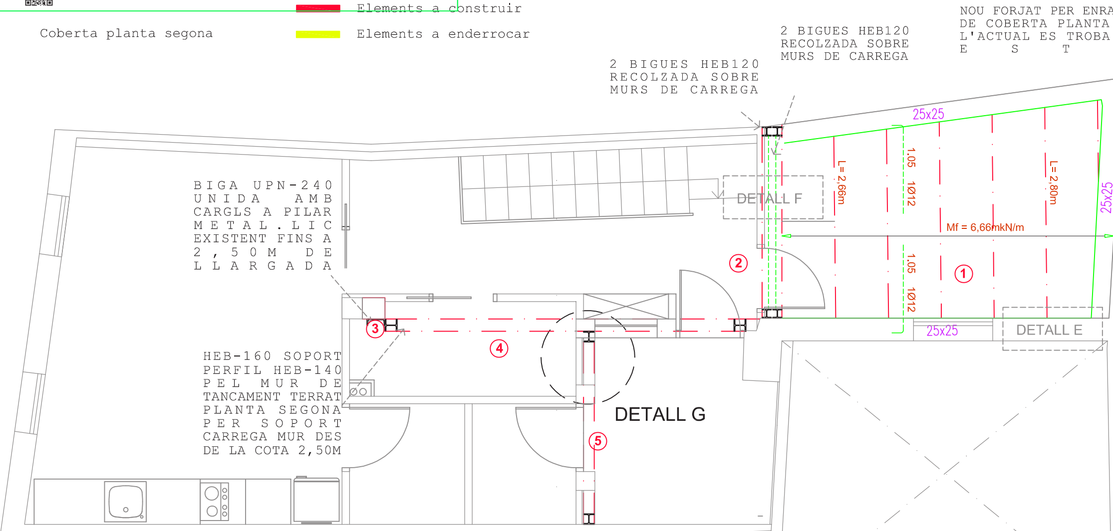
planta segona
