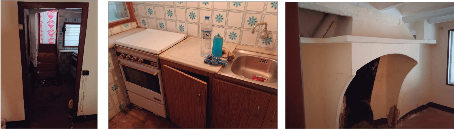
19.20.21. ENDERROC TOTAL DELS ELEMENTS CONSTRUCTIUS DE LA PLANTA ENTRESOL
