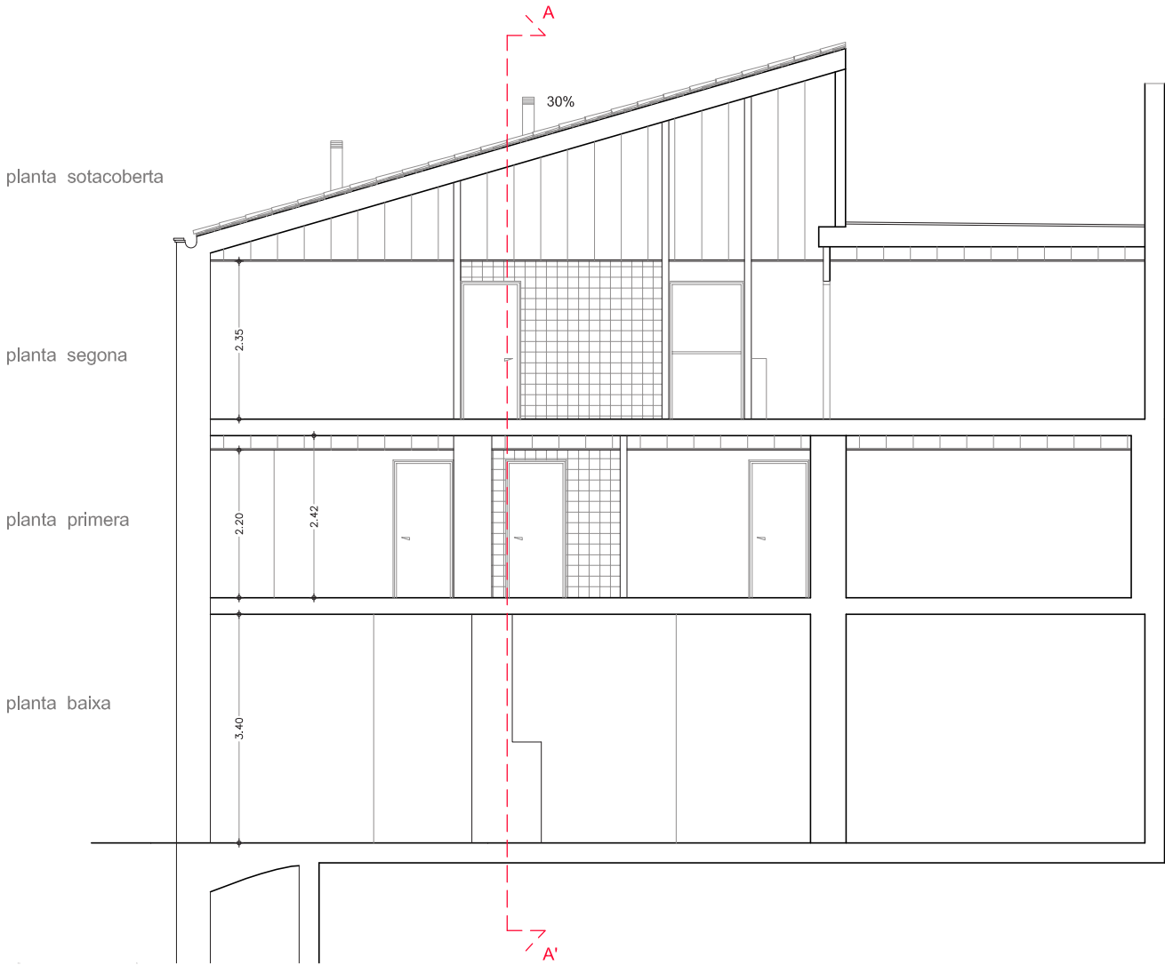
Secció A-A'
