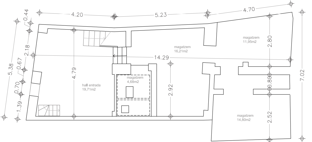
planta semisoterrani
