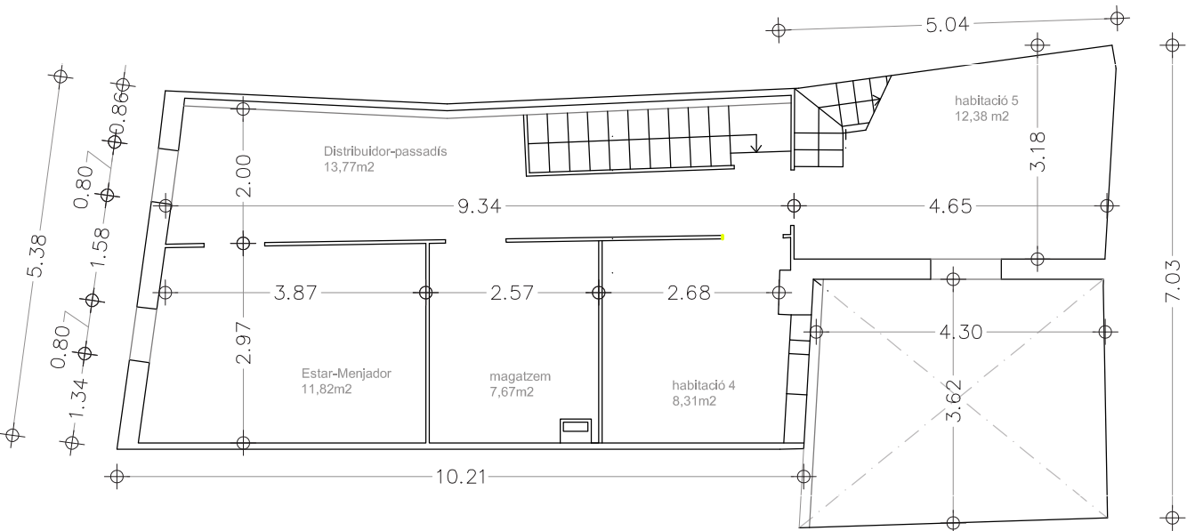
planta segona
