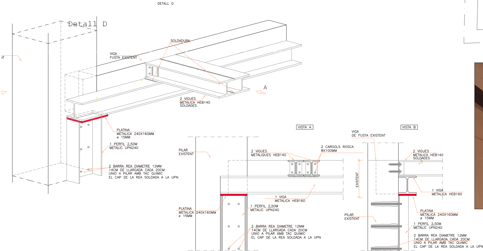
planta primera Forjat planta Primera
