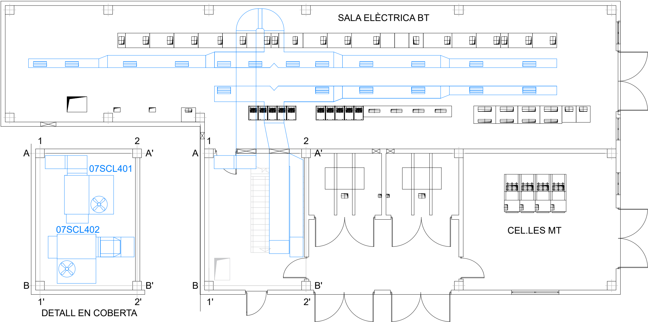
PLANTA ITAM LLOBREGAT E 1/4000
