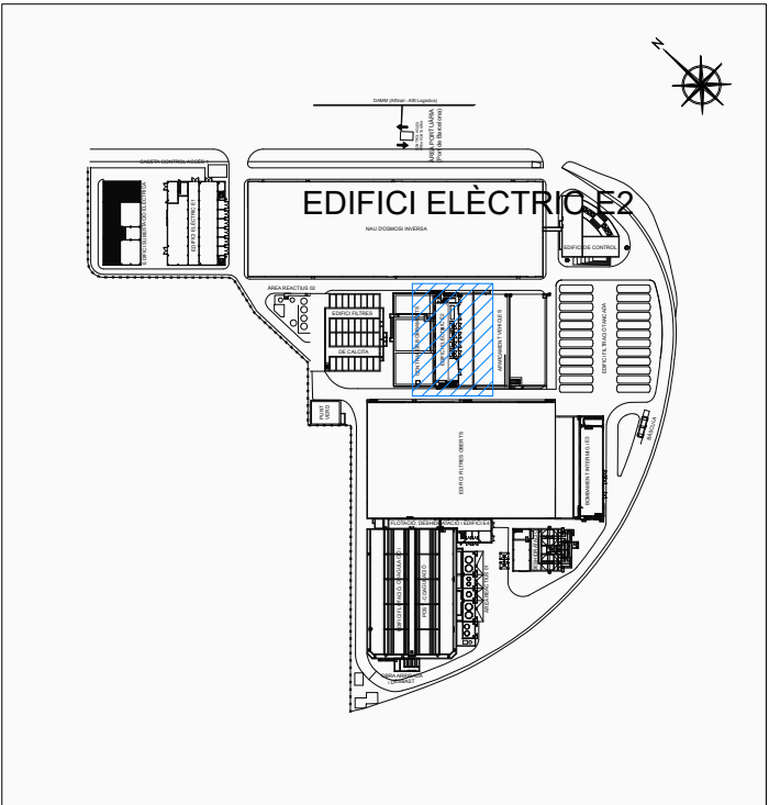
PLANTA ITAM LLOBREGAT E 1/4000
