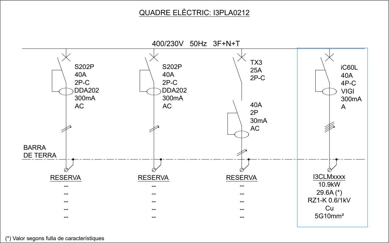
DETALL INSTAL·LACIÓ ELÈCTRICA
