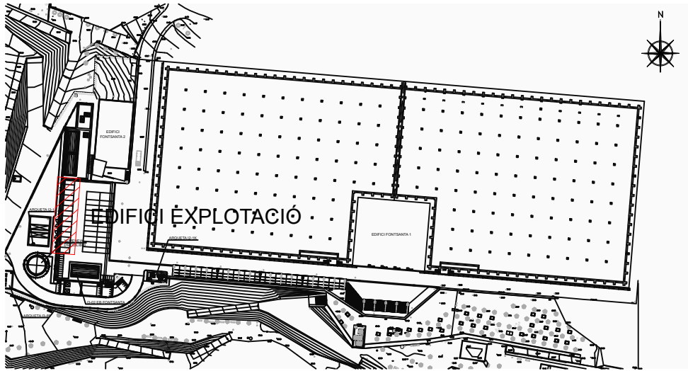
PLANTA EDIFICI FONTSANTA E 1/2500
