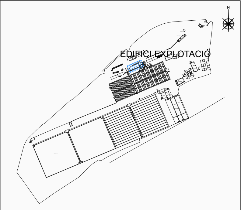
PLANTA ETAP TER E 1/10000
