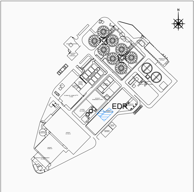
PLANTA ETAP LLOBREGAT E 1/5000
