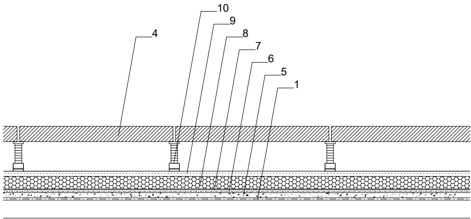
PROPOSTA. SECCIÓ DETALL TIPUS. Esc: 1 / 15
