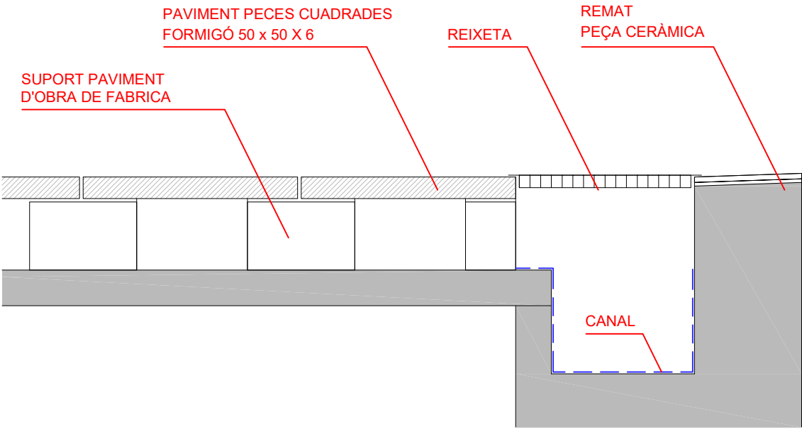
ESTAT ACTUAL. SECCIÓ ZONA CANAL. Esc: 1 / 15
