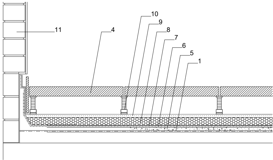
PROPOSTA. SECCIÓ ENTREGA PARAMENTS VERTICALS. Esc: 1 / 15
