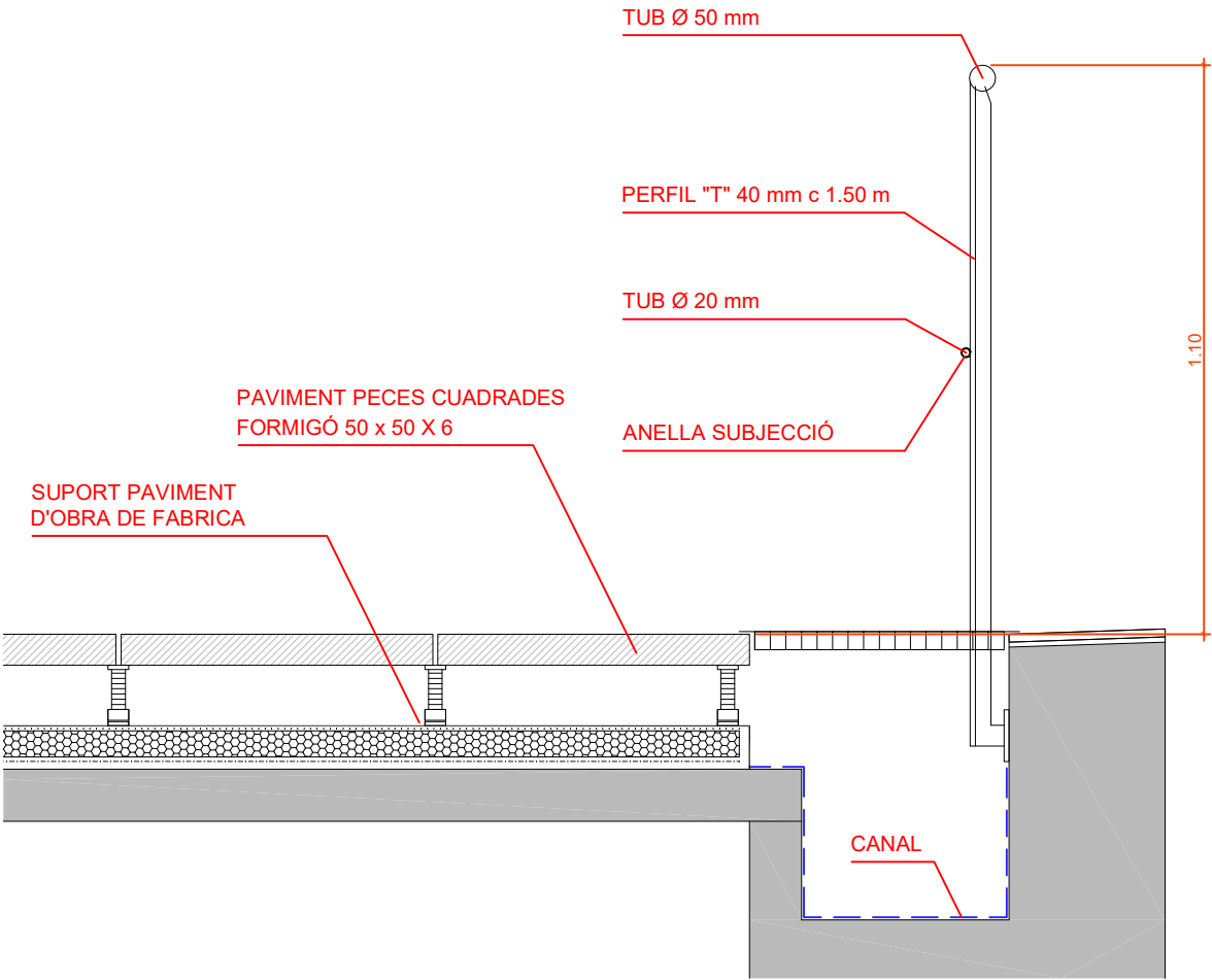
PROPOSTA. SECCIÓ ZONA CANAL. Esc: 1 / 15
