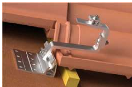
Detalle: Gancho en aluminio GTA 3
