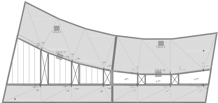
COBERTA PLANA 1:100
