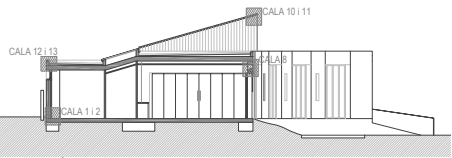
SECCO TRANSVERSAL 4 1:100
