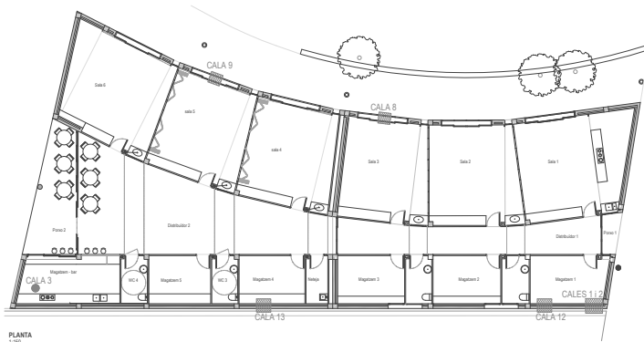
PLANTA 1:100
