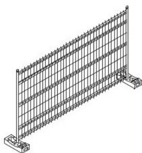
DETALL Tanca metàl·lica tipus Rivisa
