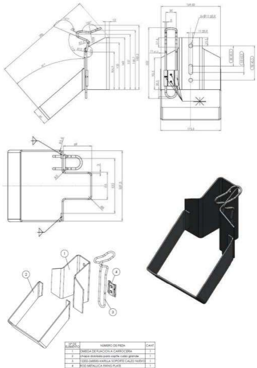
Figura 5. Soporte calzo
