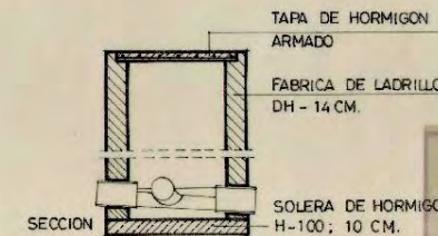
SECCION
