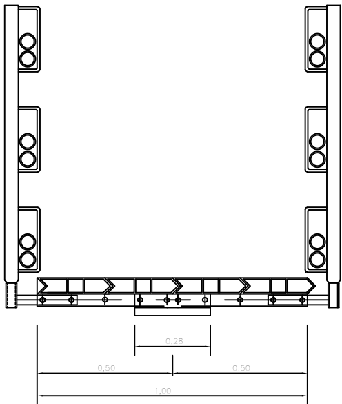
SECCIÓ ESCALA 1/10
