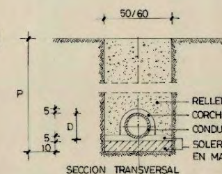
SECCION TRANSVERSAL
