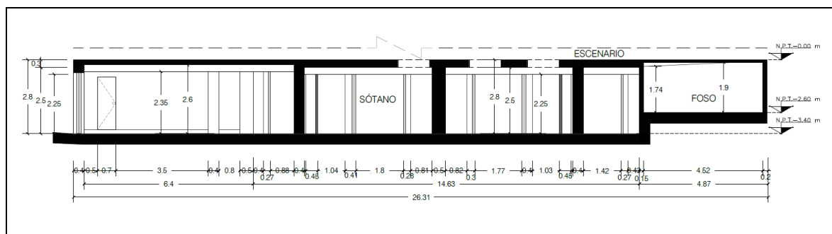
Secció del soterrani
