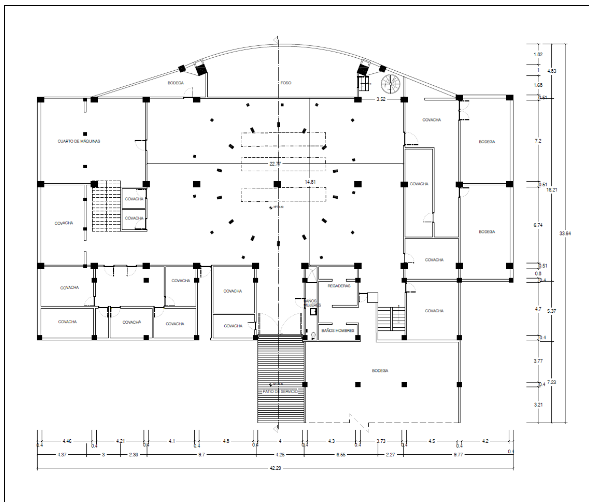
Planta soterrani
