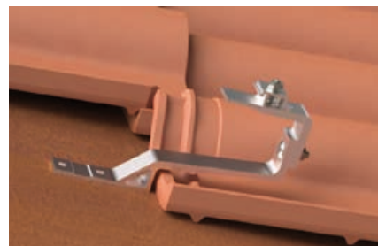
Detalle: Gancho para teja plana en aluminio GTA 1
