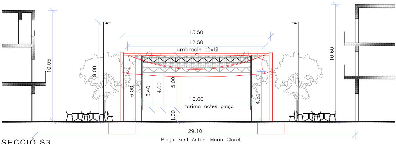
SECCIÓ S3
