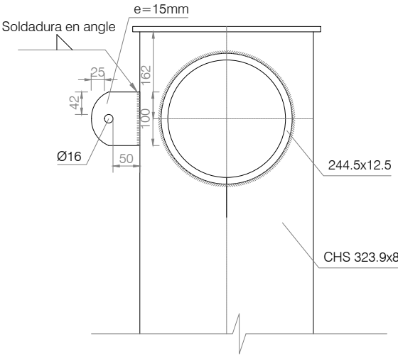
C-DET-03
