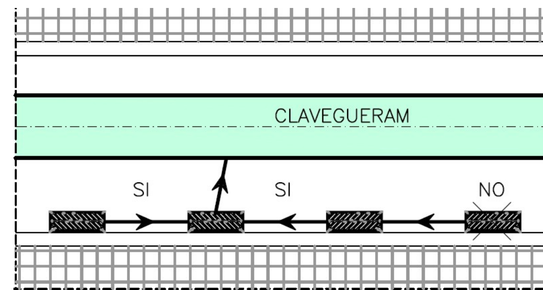
Figura 1. Esquema de disposició d'embornals i connexions.
